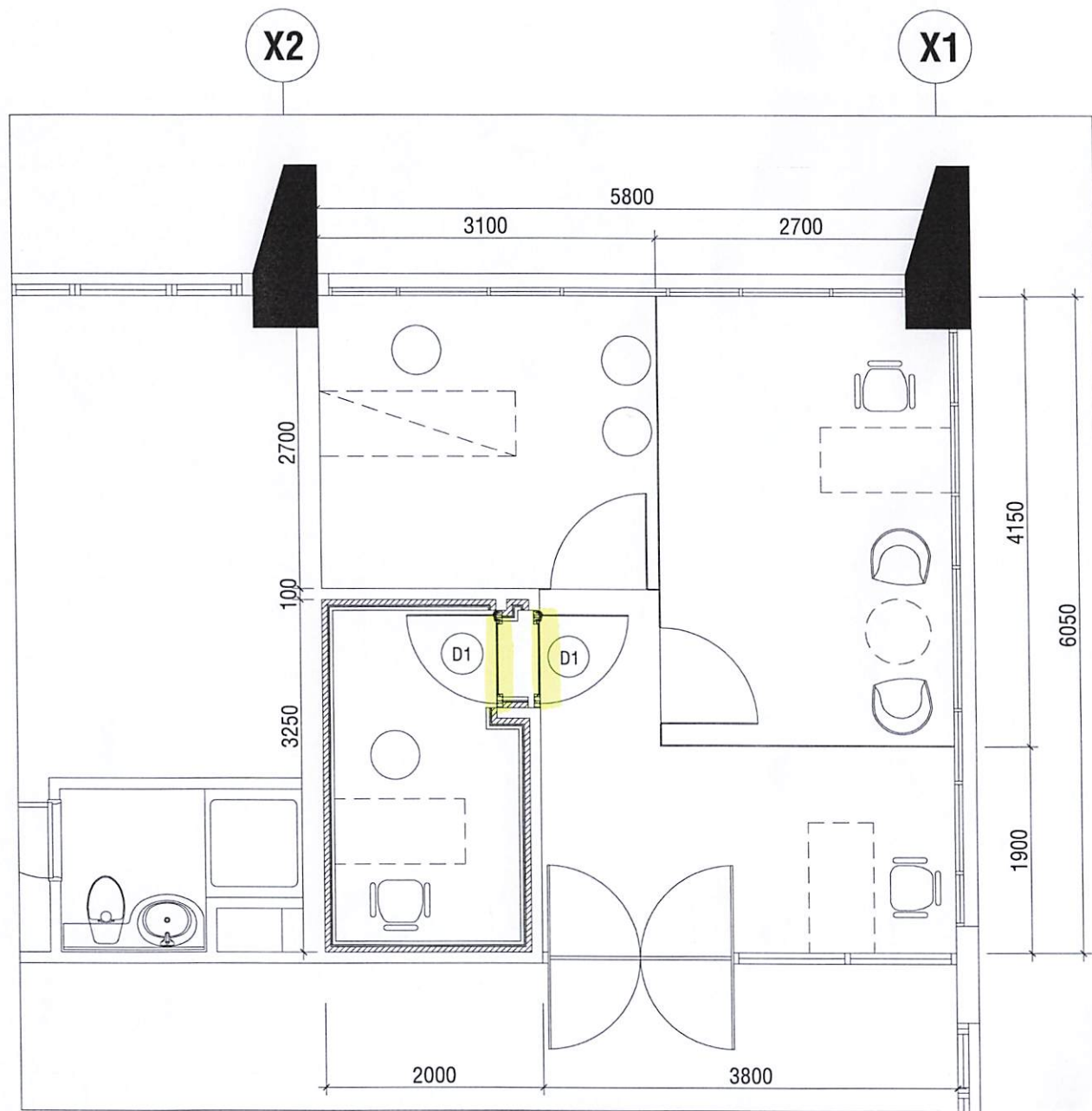
MẶT BẰNG CỬA ĐI NHÔM KÍNH LẦU 12 BLOCK A
