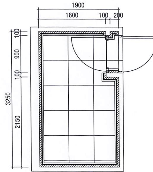
MẶT BẰNG TRẢI THẨM
