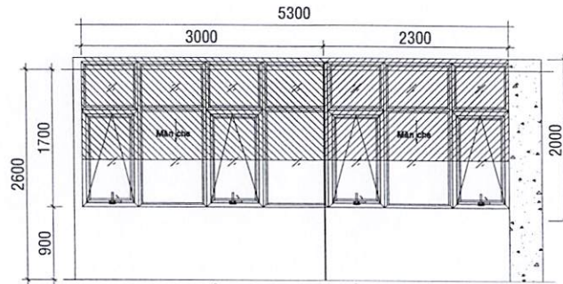
MẶT ĐÚNG BỐ TRÍ MÀN CHE CỬA SỐ LẦU 12 BLOCK A HƯỚNG NHÌN 1
