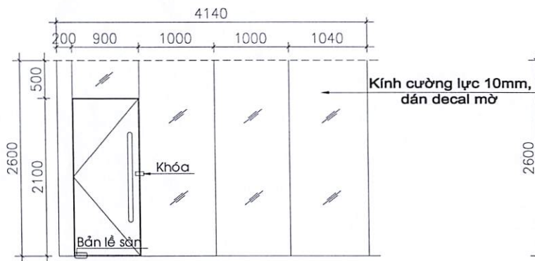
VÁCH KÍNH VK4
