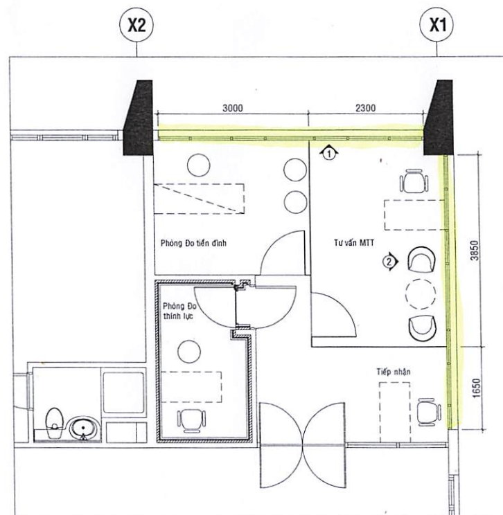
MẶT BẰNG BỐ TRÍ MÀN CHE CỬA SỔ LẦU 12 BLOCK A
