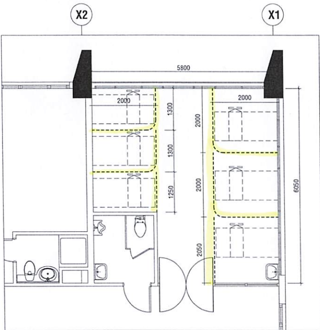
MẶT BẰNG BỐ TRÍ RÈM CHE Y TẾ LẦU 7 BLOCK A
