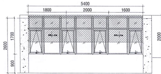
MẶT ĐÚNG BỐ TRÍ MÀN CHE CỬA SỐ LẦU 13 BLOCK B HƯỚNG NHÌN 5
