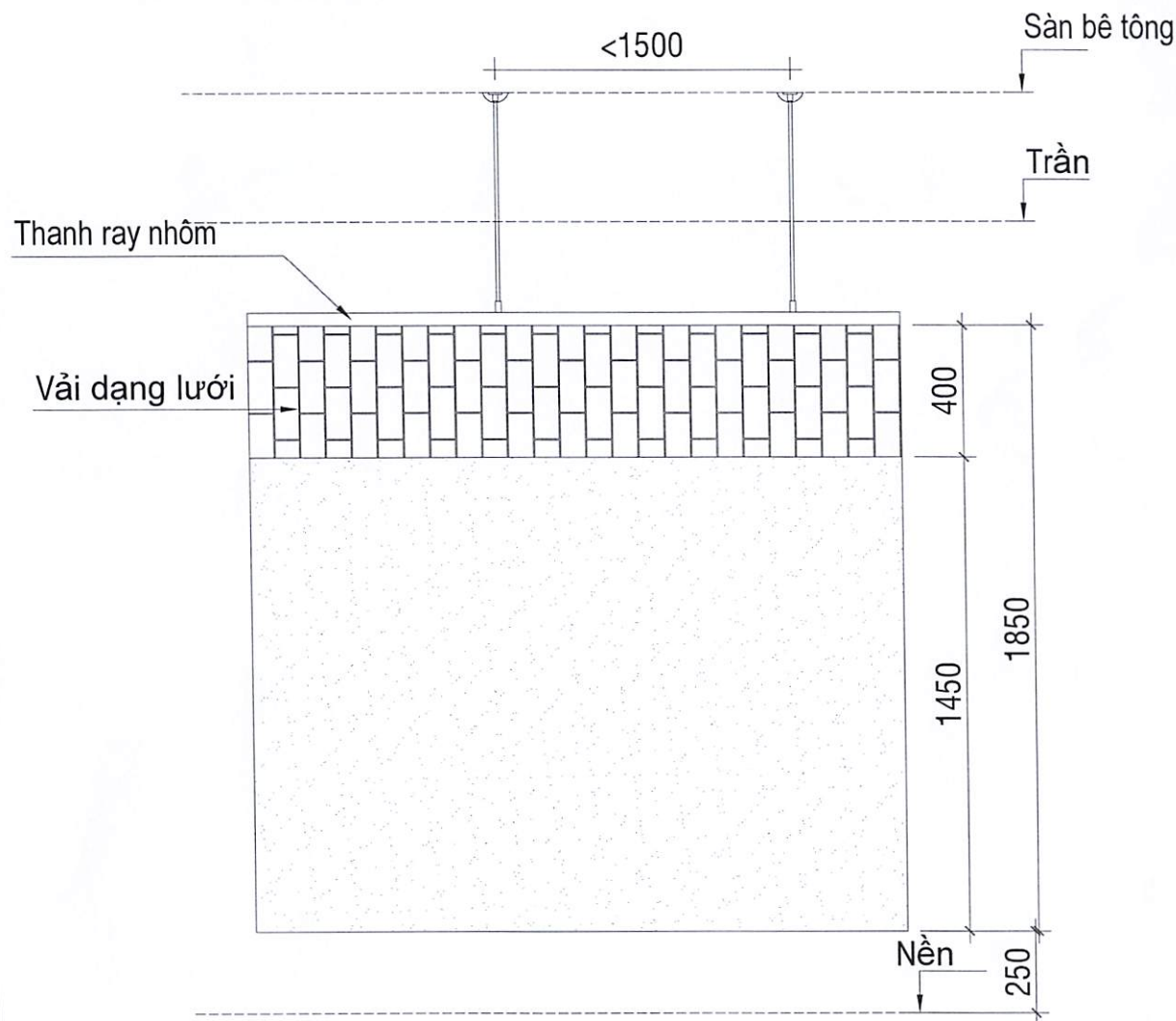
CHI TIẾT RÈM CHE
