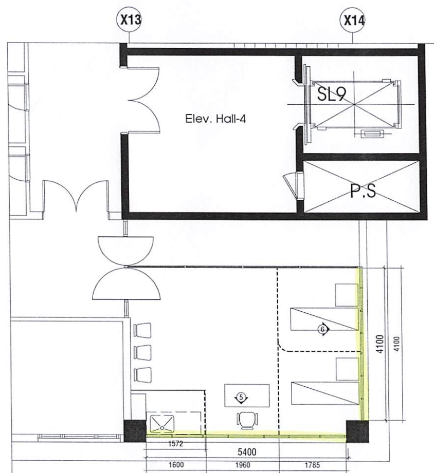
MẶT BẰNG BỐ TRÍ MÀN CHE CỬA SỔ LẦU 13 BLOCK B
