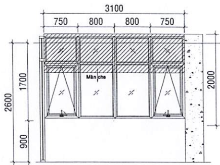
MẶT ĐÚNG BỐ TRÍ MÀN CHE CỬA SỐ LẦU 7 BLOCK B
