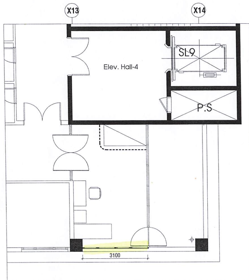
MẶT BẰNG BỐ TRÍ MÀN CHE CỬA SỔ LẦU 7 BLOCK B
