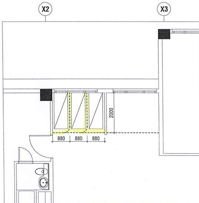
MẶT BẰNG BỐ TRÍ RÈM CHE Y TẾ LẦU 9 BLOCK A
