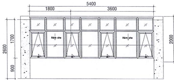
MẶT ĐÚNG BỐ TRÍ MÀN CHE CỬA SỐ LẦU 12 BLOCK B HƯỚNG NHÌN 3
