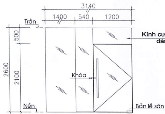
VÁCH KÍNH VK2
