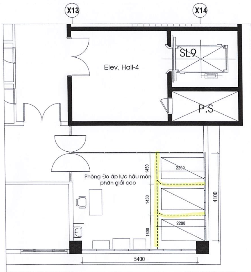
MẶT BẰNG BỐ TRÍ RÈM CHE Y TẾ LẦU 12 BLOCK B
