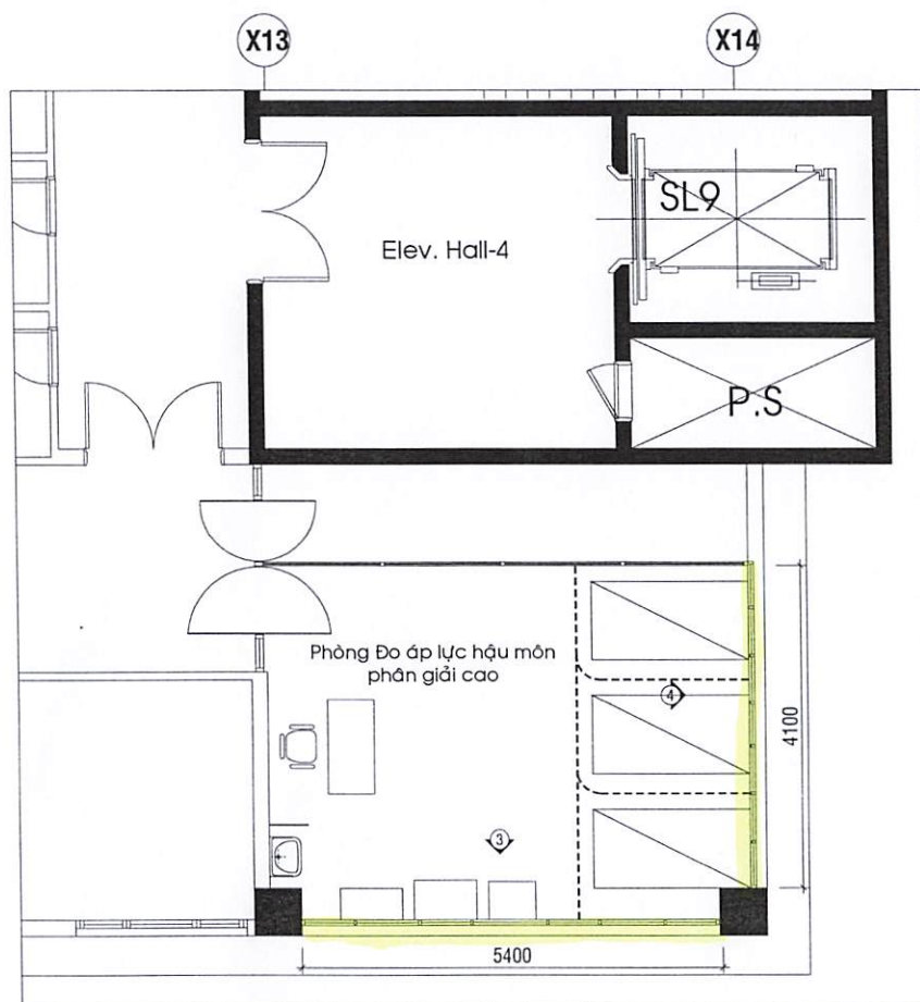
MẶT BẰNG BỐ TRÍ MÀN CHE CỬA SỔ LẦU 12 BLOCK B
