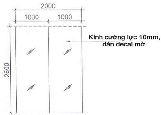
VÁCH KÍNH VK7
