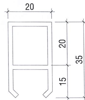
CHI TIẾT THANH RAY NHÔM
