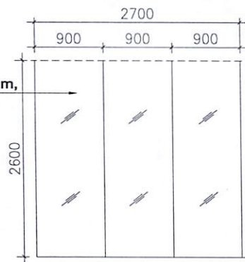
VÁCH KÍNH VK5
