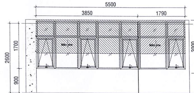
MẶT ĐÚNG BỐ TRÍ MÀN CHE CỬA SỐ LẦU 12 BLOCK A HƯỚNG NHÌN 2
