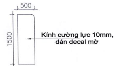
VÁCH KÍNH VK6
