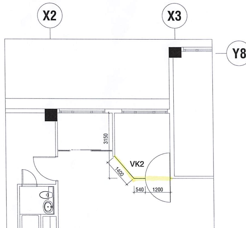
MẶT BẰNG VÁCH KÍNH LẦU 8 BLOCK A
