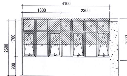
MẶT ĐÚNG BỐ TRÍ MÀN CHE CỬA SỐ LẦU 12 BLOCK B HƯỚNG NHÌN 4
