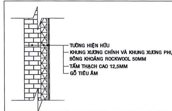
CHI TIẾT VÁCH THẠCH CAO
