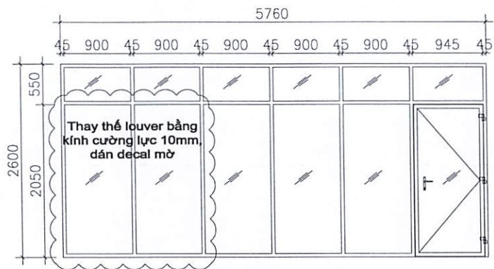
VÁCH KÍNH VK1
