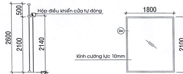
CÁNH CỬA LÙA
