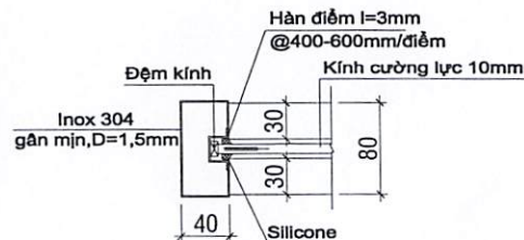
CHI TIẾT D1
