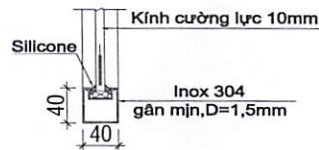
CHI TIẾT D4
