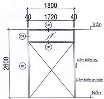
MẶT ĐỨNG VÁCH KÍNH
