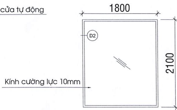
CÁNH CỬA LÙA
