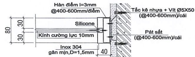
CHI TIẾT D3
