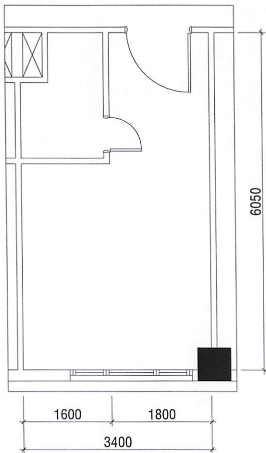
PHÒNG 24 LẦU 7 (TRƯỚC KHI CẢI TẠO)
