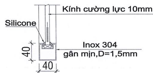
CHI TIẾT D2
