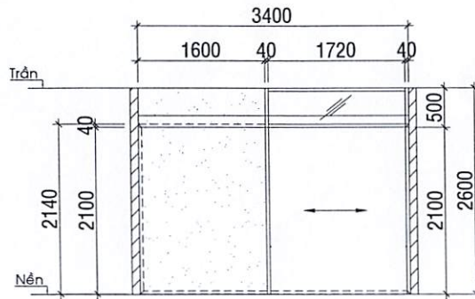
MẶT ĐỨNG CỬA LÙA
