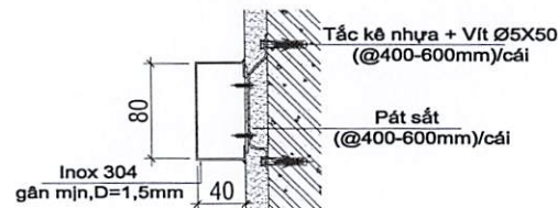
CHI TIẾT D2
