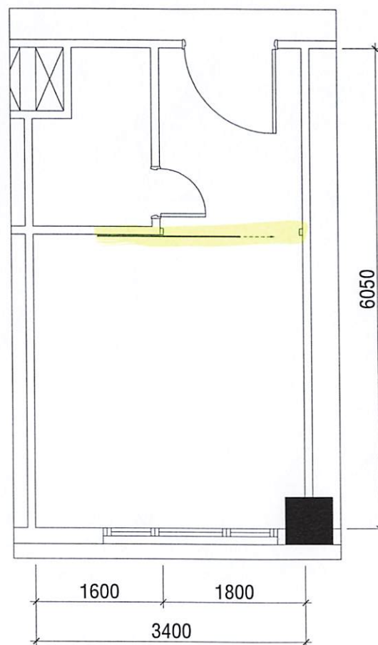
PHÒNG 24 LẦU 7 (SAU KHI CẢI TẠO)
