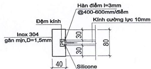
CHI TIẾT D1
