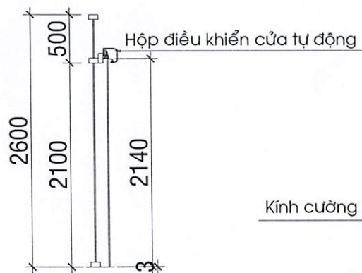
MẶT CẮT
