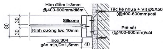
CHI TIẾT D3
