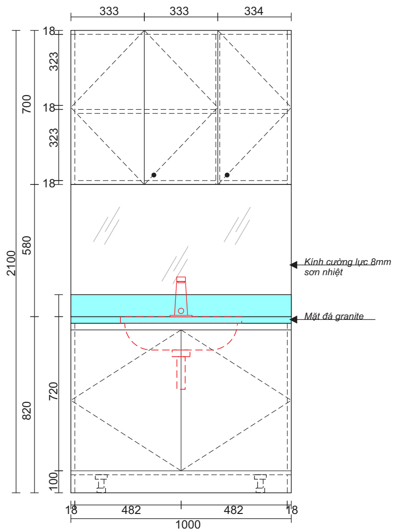
MẶT ĐỨNG
