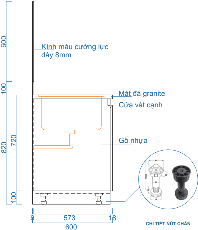
MẶT BÊN
