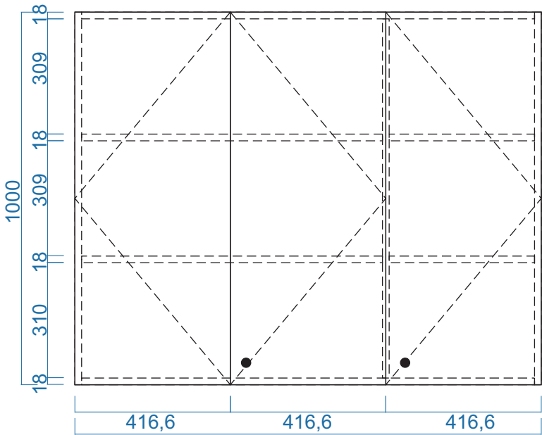
MẶT ĐỨNG
