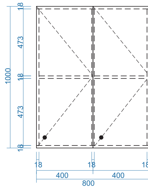
MẶT ĐÚNG
