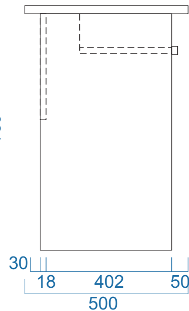
MẶT BÊN
