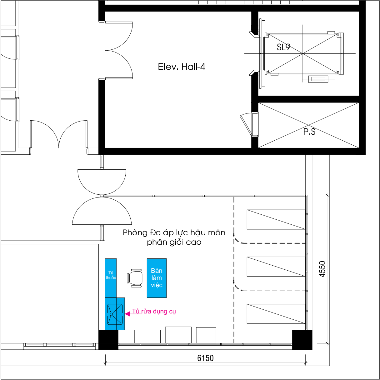
MẶT BẰNG BỐ TRÍ NỘI THẤT PHÒNG ĐO ÁP LỰC HẬU MÔN PHÂN GIẢI CAO KHOA HẬU MÔN TRỰC TRÀNG
