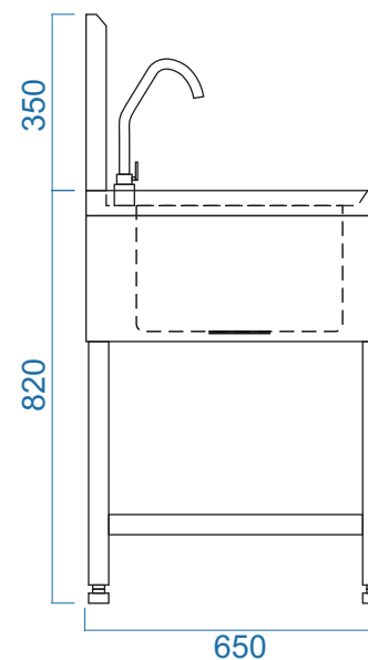
MẶT BÊN
