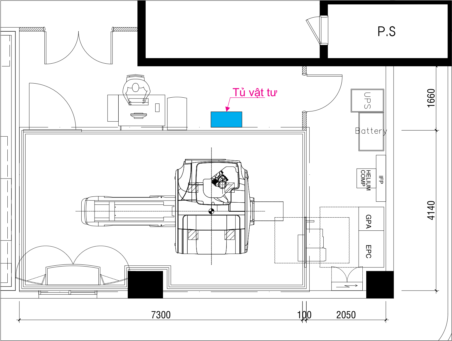
MẶT BẰNG BỐ TRÍ NỘI THẤT PHÒNG MRI - TRỆT A
