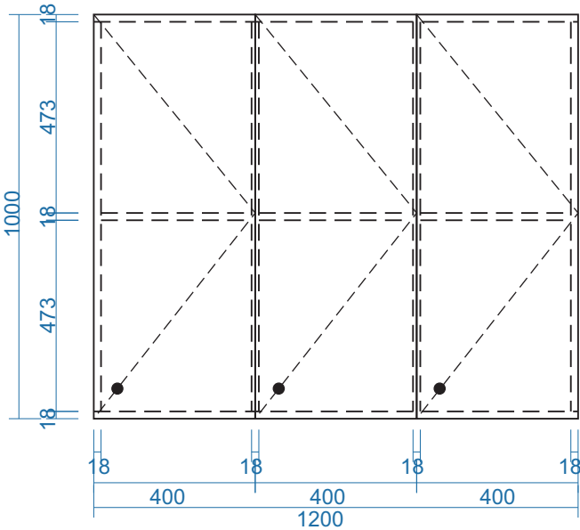
MẶT ĐỨNG
