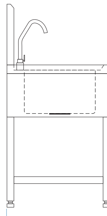
MẶT BÊN
