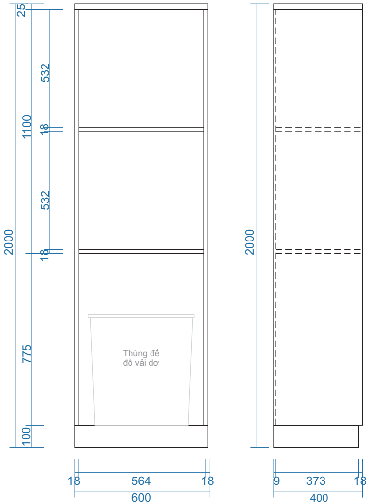
MẶT ĐỨNG
