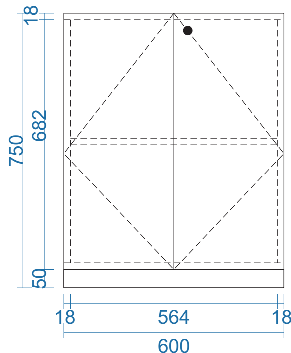
MẶT ĐỨNG
