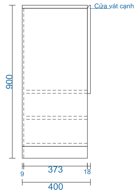
MẶT BÊN
