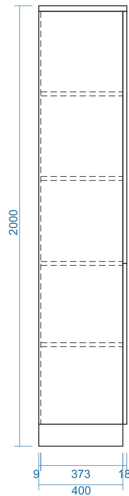
MẶT BÊN
