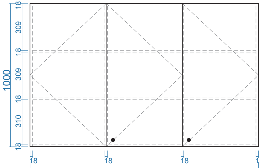
MẶT ĐỨNG
