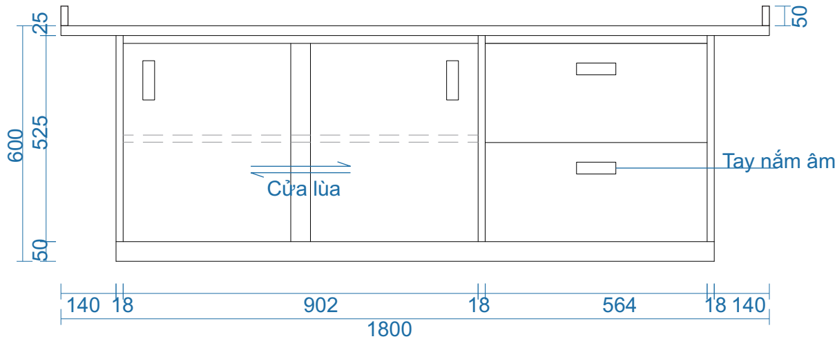
MẶT ĐỨNG
