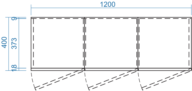
MẶT BẰNG
