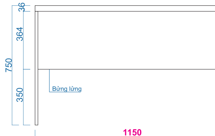
MẶT ĐỨNG
