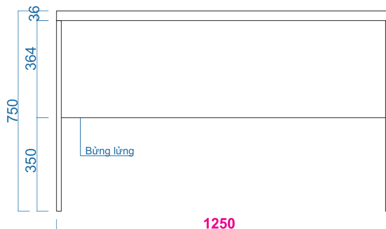
MẶT ĐỨNG
