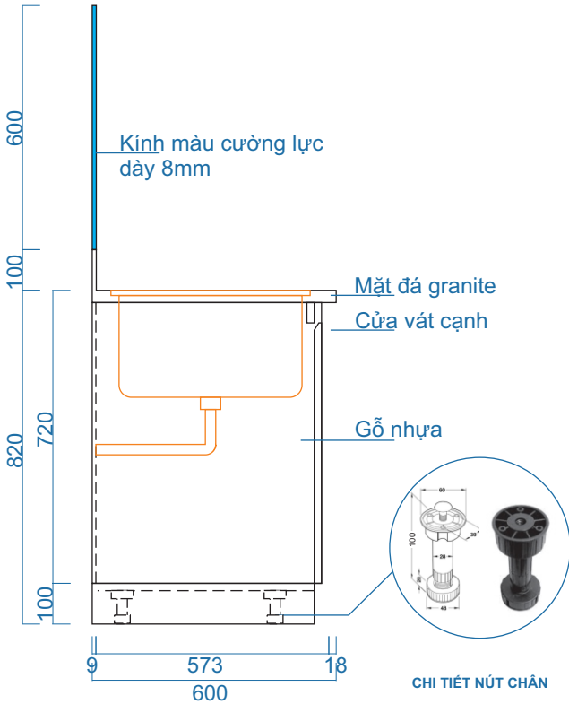
MẶT BÊN
