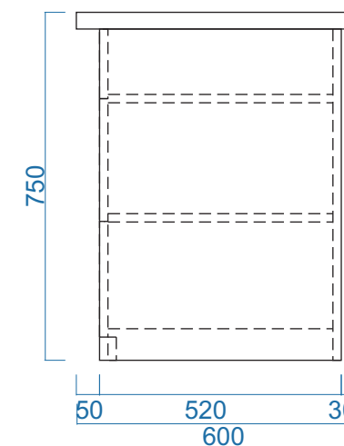
MẶT BÊN
