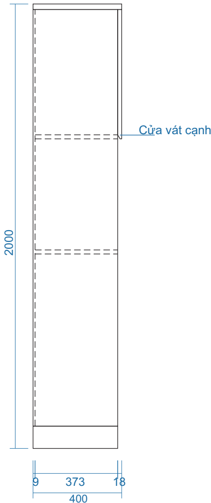
MẶT BÊN
