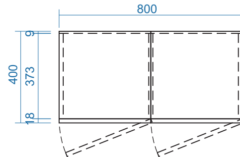
MẶT BẰNG
