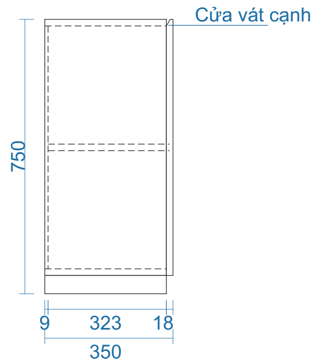
MẶT BÊN
