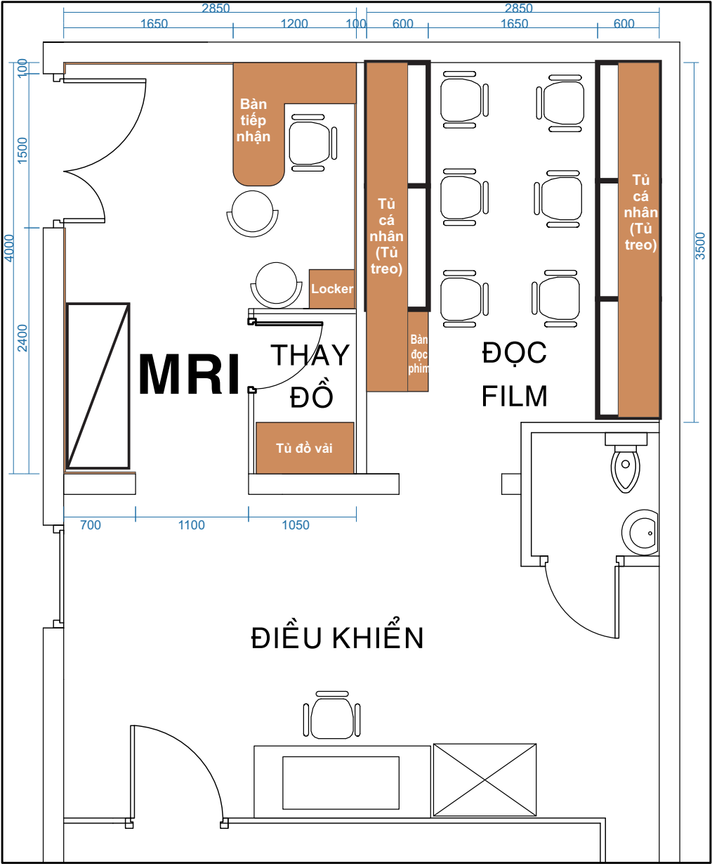
MẶT BẰNG CẢI TẠO PHÒNG MRI TRỆT B
