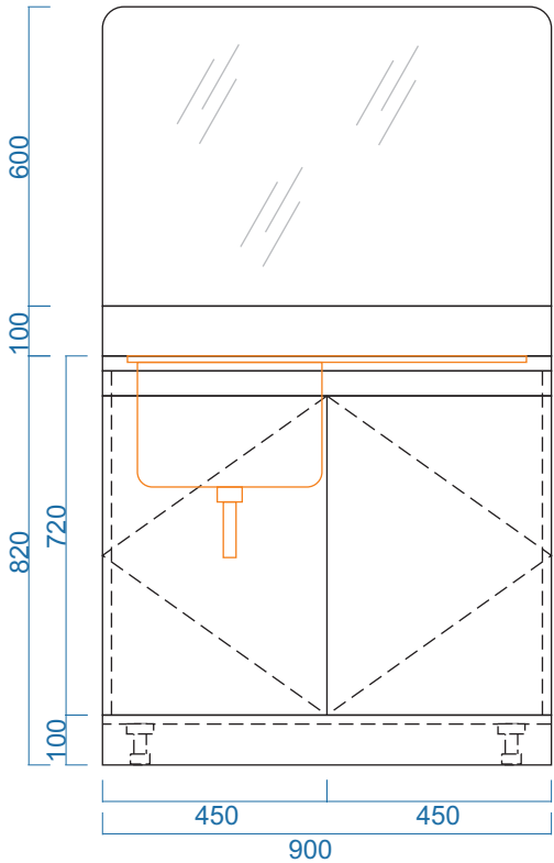
MẶT ĐỨNG
