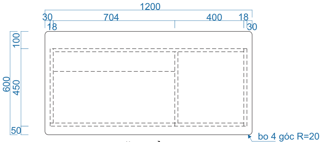
MẶT BẰNG
