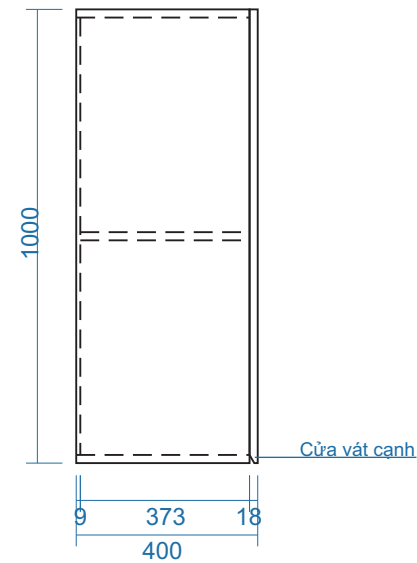
MẶT BÊN
