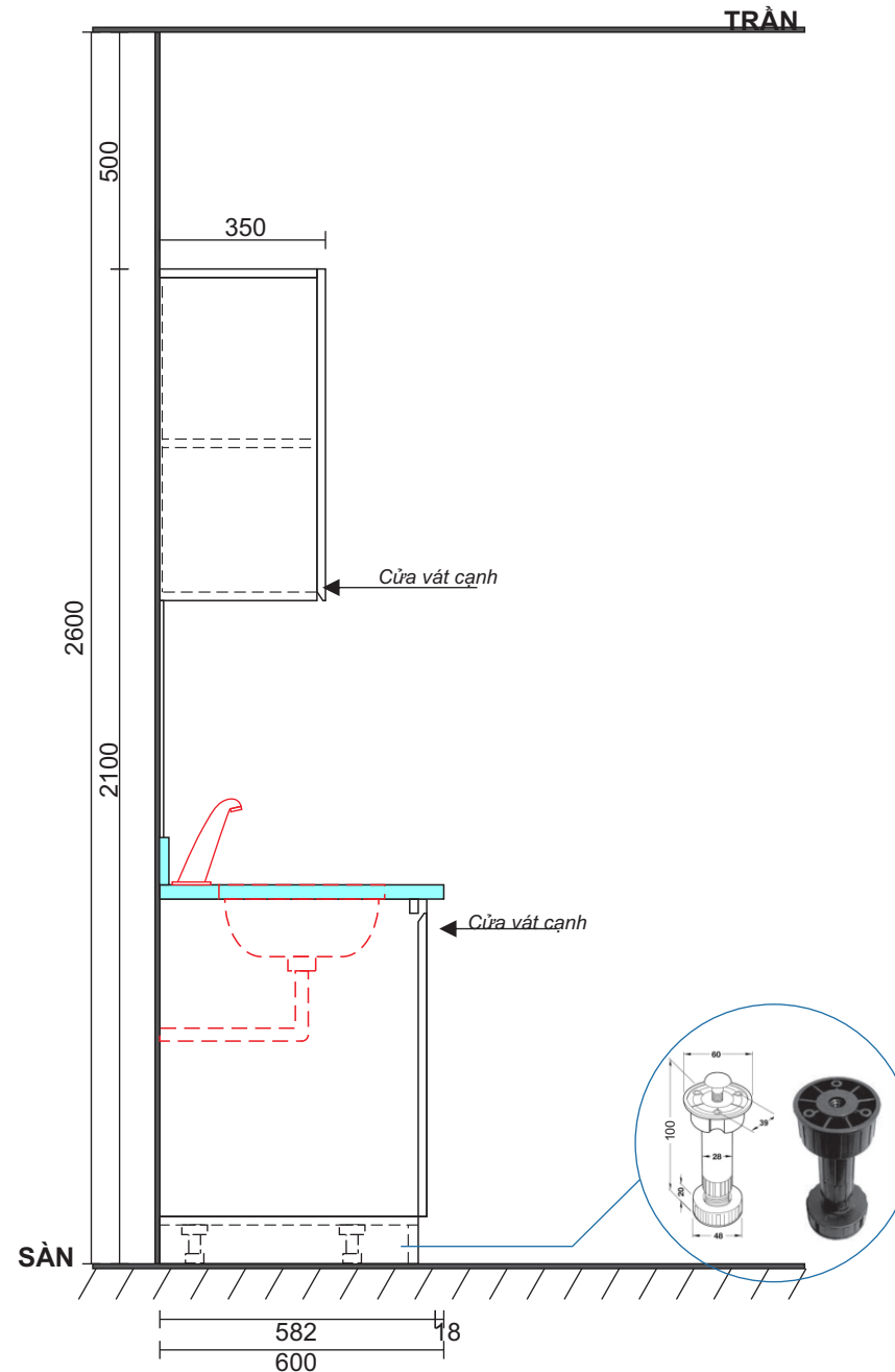
MẶT BÊN
