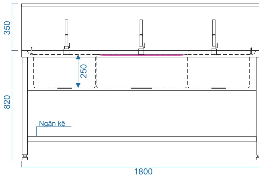
MẶT ĐỨNG
