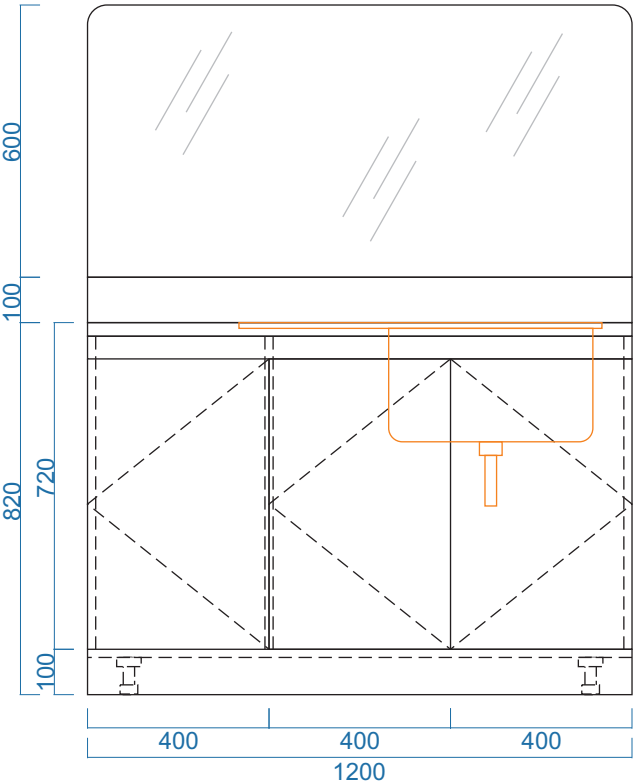
MẶT ĐỨNG
