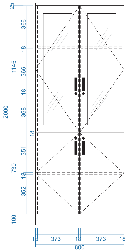
MẶT ĐỨNG
