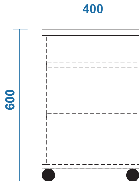
MẶT BÊN
