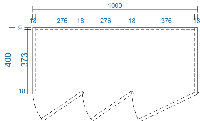
MẶT BẰNG
