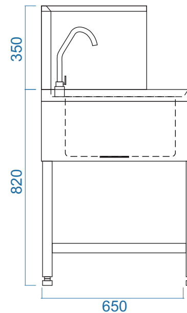
MẶT BÊN
