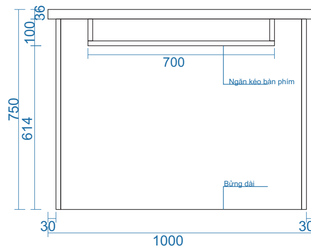
MẶT ĐỨNG
