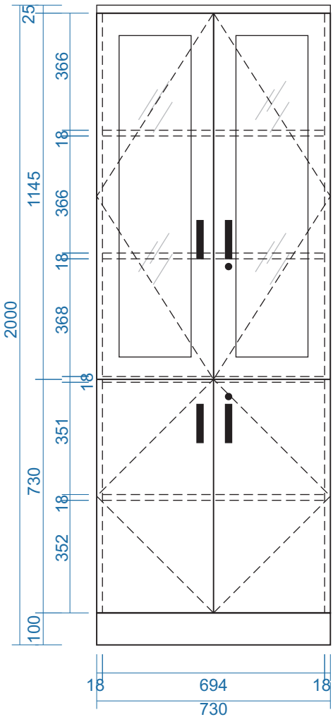
MẶT ĐỨNG
