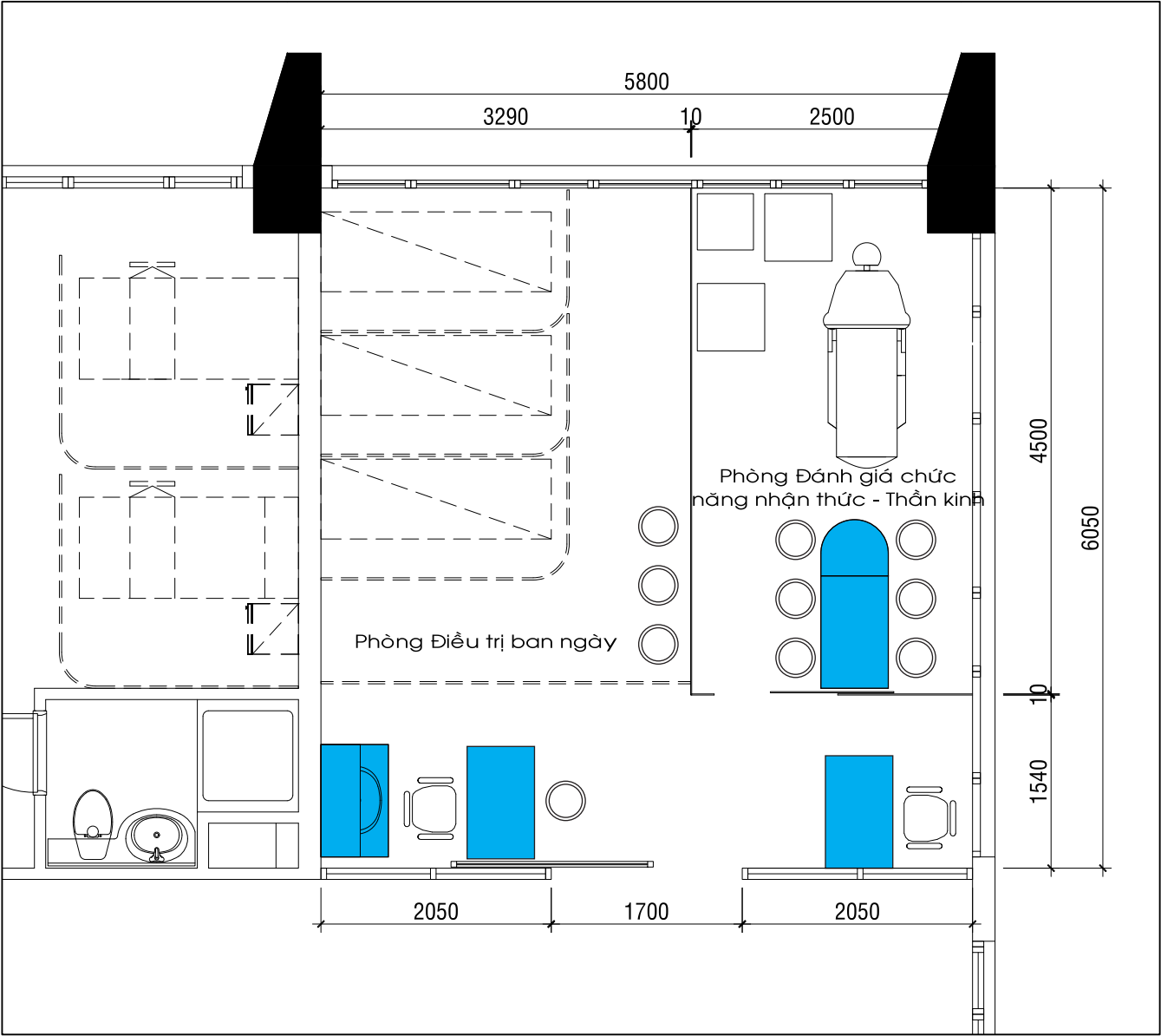
MẶT BẰNG BỐ TRÍ NỘI THẤT PHÒNG ĐIỀU TRỊ BAN NGÀY, PHÒNG ĐÁNH GIÁ CHỨC NĂNG NHẬN THỨC KHOA THẦN KINH
