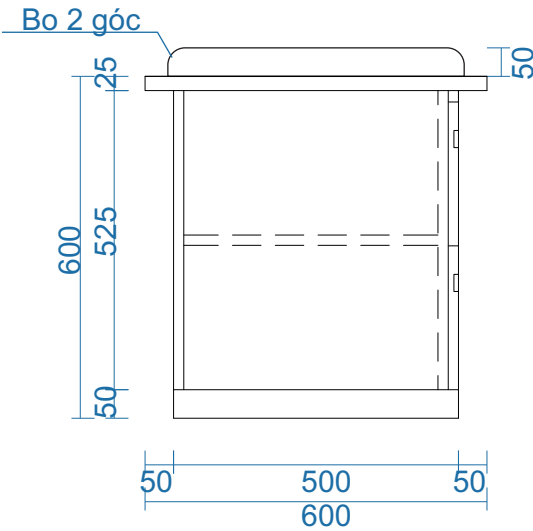
MẶT BÊN
