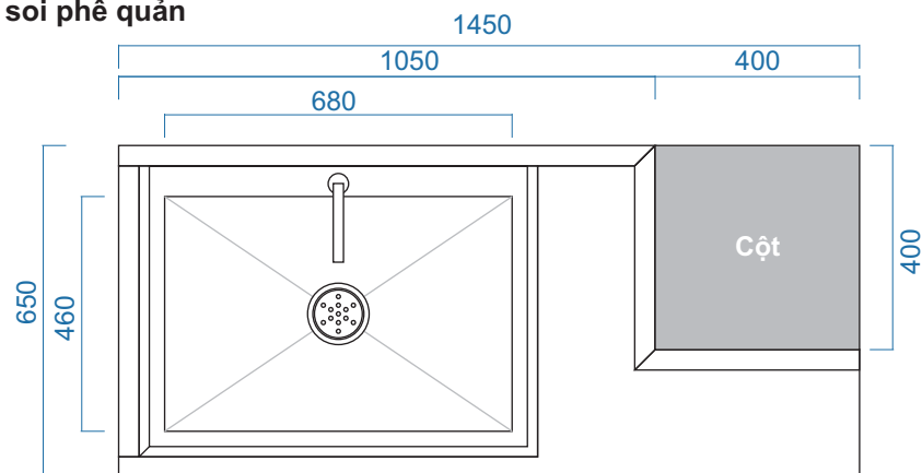
MẶT BẰNG
