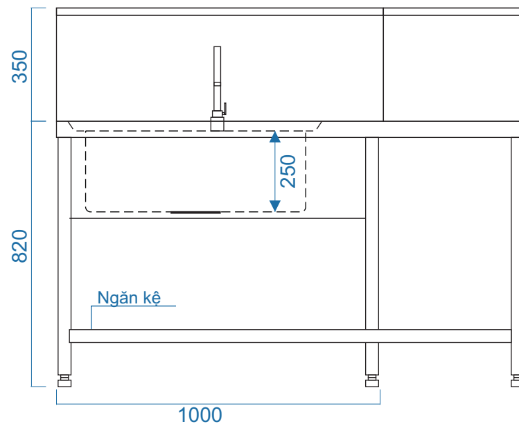
MẶT ĐỨNG
