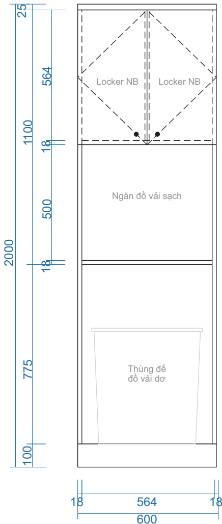
MẶT ĐỨNG
