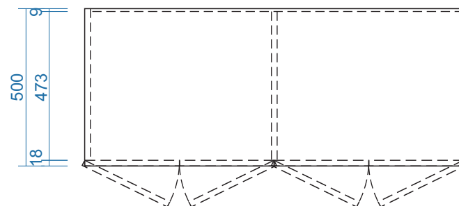
MẶT BÀNG
