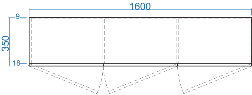
MẶT BẰNG
