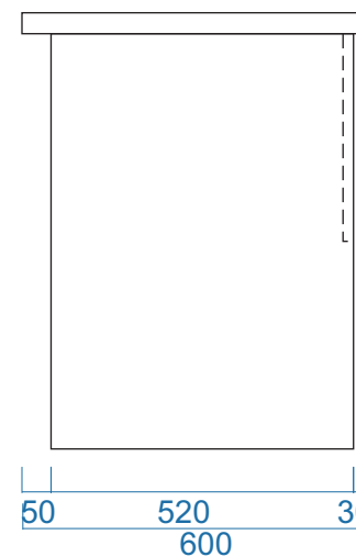
MẶT BÊN
