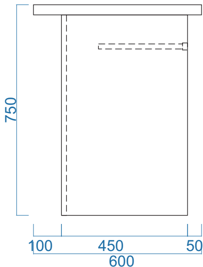
MẶT BÊN
