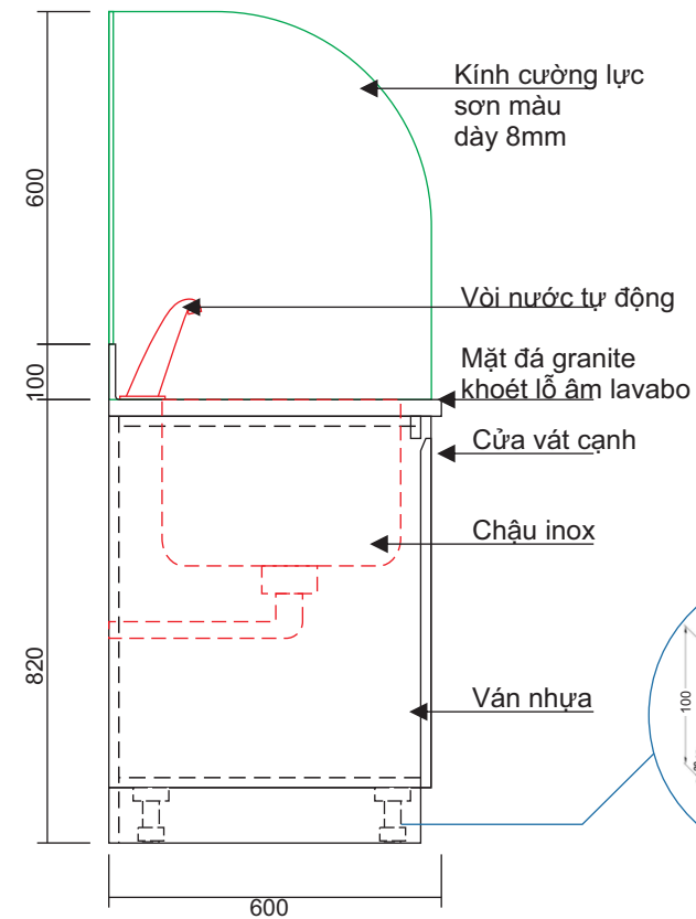
MẶT BÊN
