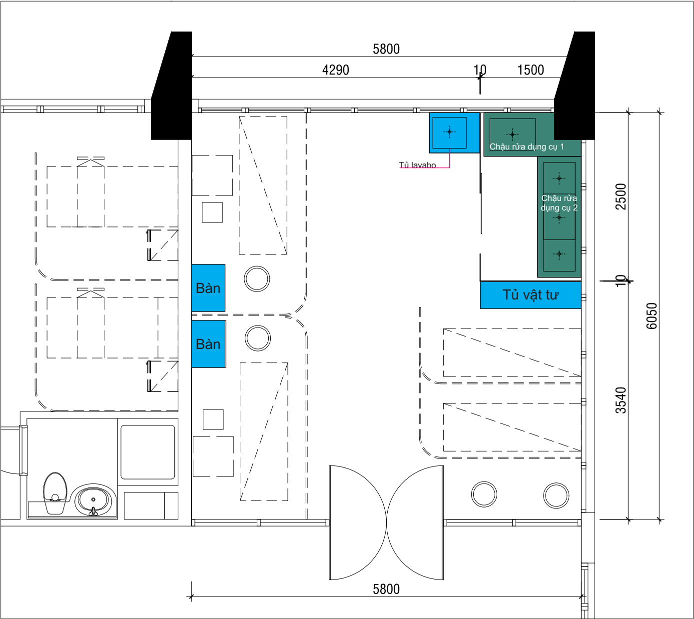
MẶT BẰNG BỐ TRÍ NỘI THẤT PHÒNG NỘI SOI PHÉ QUẢN KHÓA HỒ HẤP
