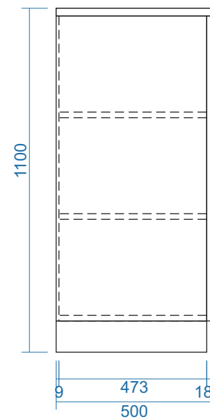
MẶT BÊN
