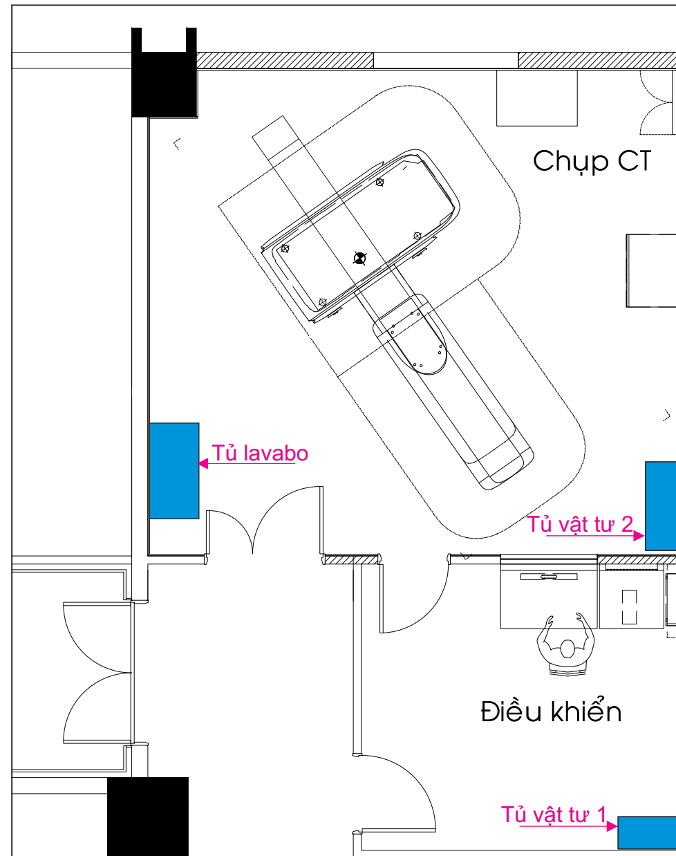
MẶT BẰNG BỐ TRÍ NỘI THẤT PHÒNG CT - TRỆT A
