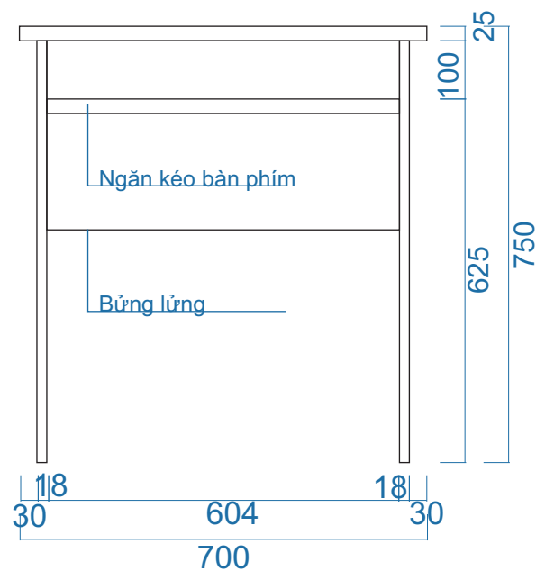
MẶT ĐỨNG
