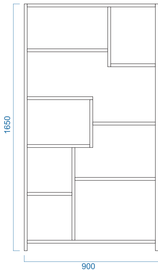
MẶT ĐỨNG
