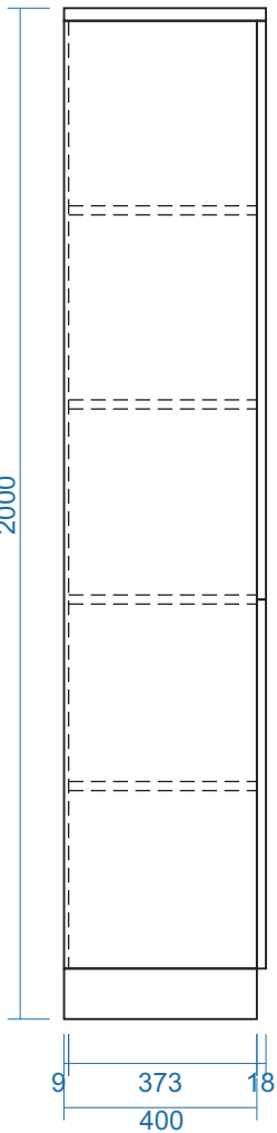
MẶT BÊN
