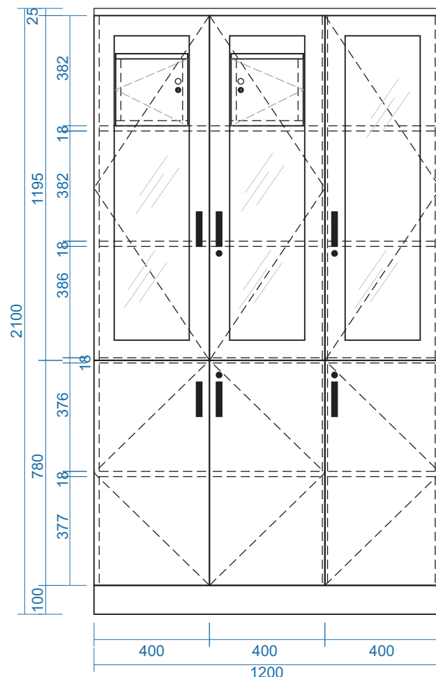
MẶT ĐỨNG
