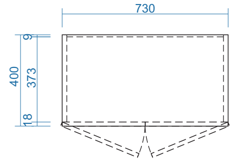
MẶT BẰNG
