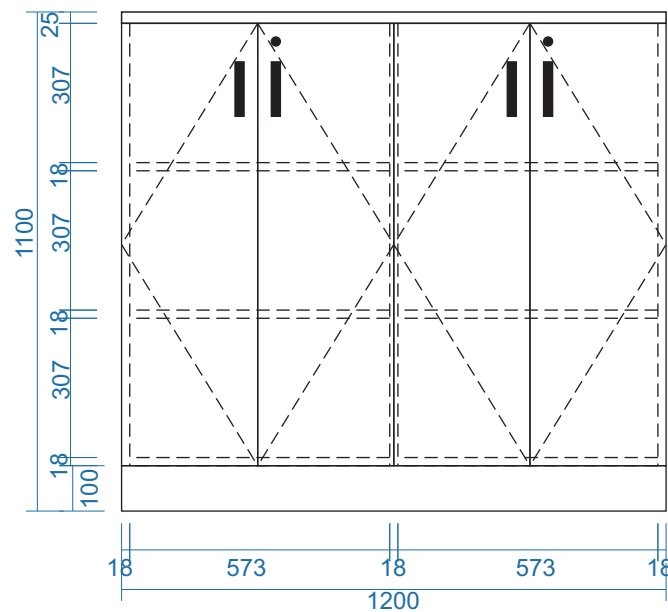
MẶT ĐỨNG
