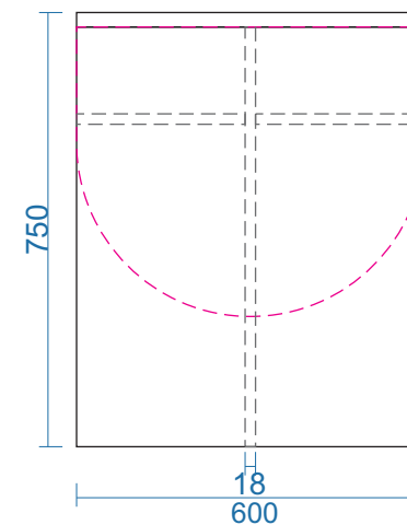
MẶT BÊN
