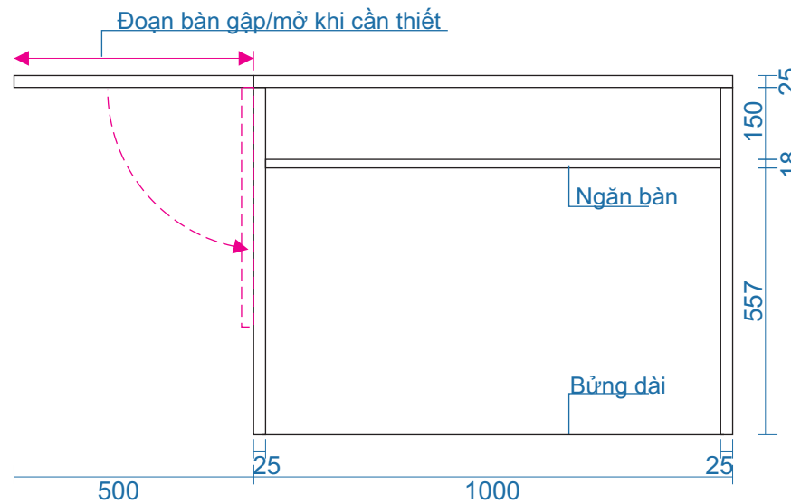
MẶT ĐÚNG
