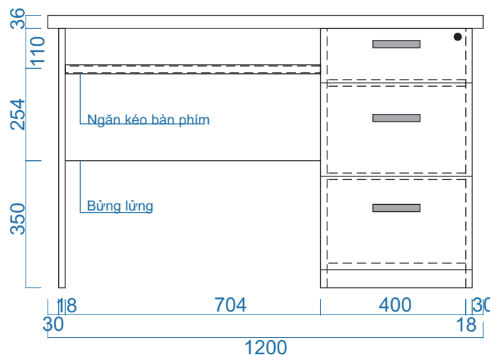
MẶT ĐỨNG
