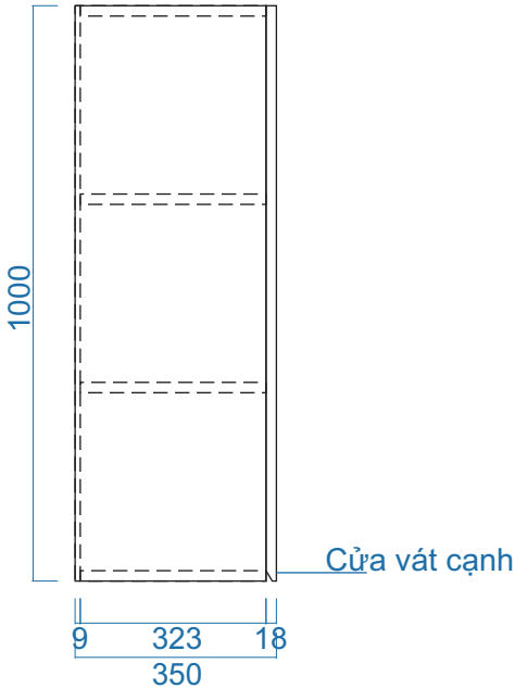
MẶT BÊN
