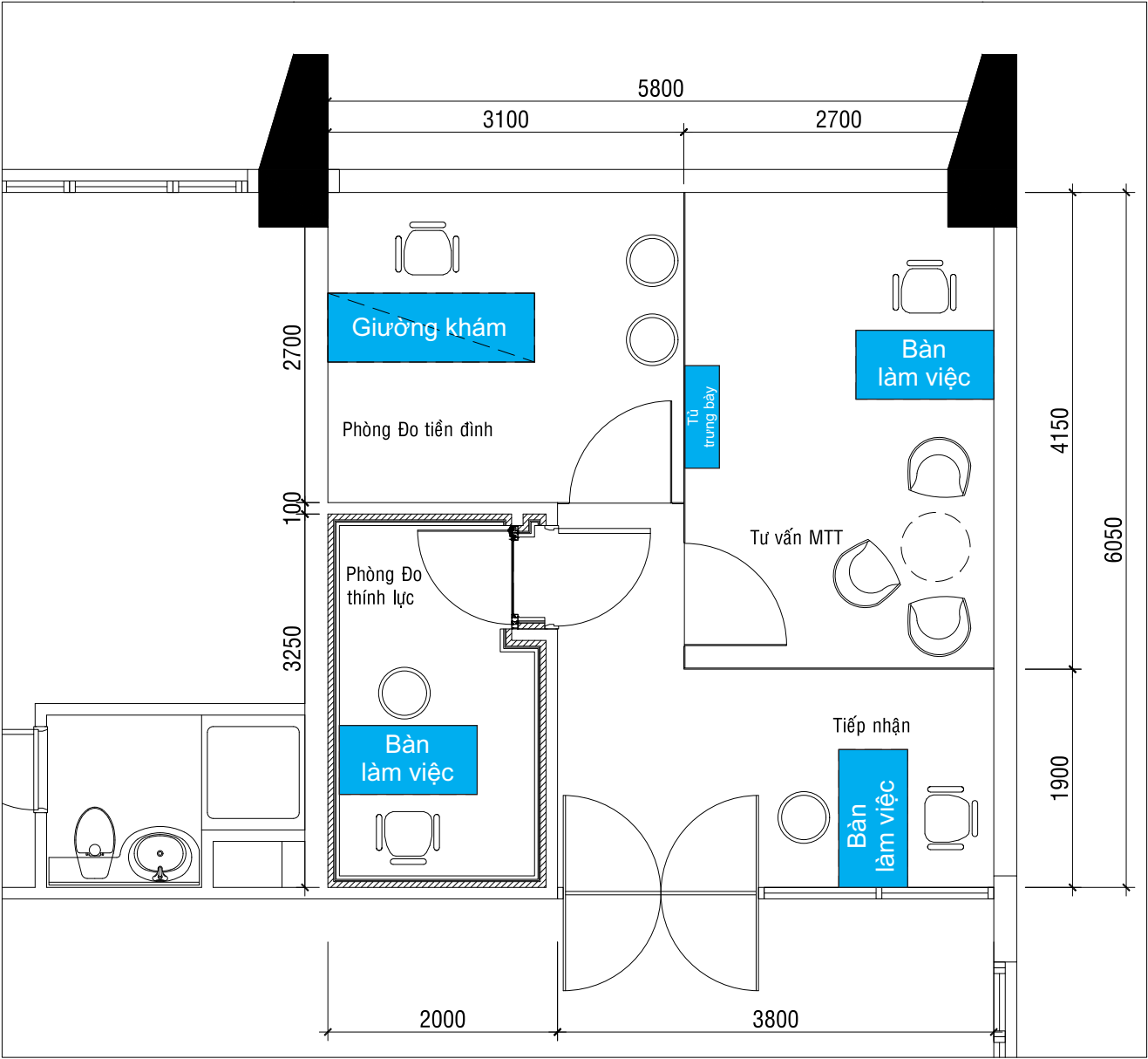
MẶT BẰNG BỐ TRÍ NỘI THẤT PHÒNG THĂM DÒ CHỨC NĂNG TẠI MŨI HỌNG KHOA TAI MŨI HỌNG
