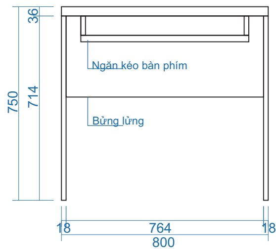
MẶT ĐỨNG
