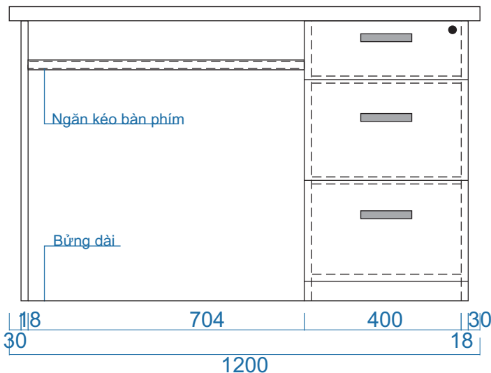
MẶT ĐỨNG
