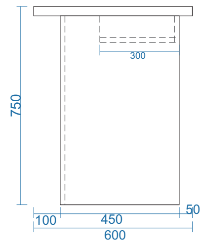
MẶT BÊN
