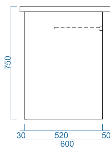
MẶT BÊN
