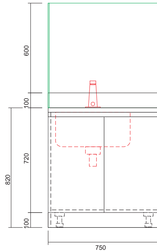
MẶT ĐỨNG
