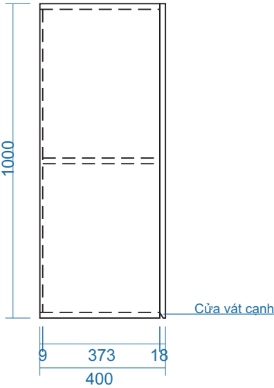
MẶT BÊN
