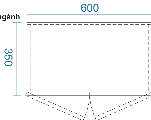
MẶT BẰNG
