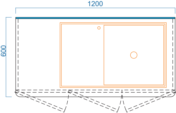
MẶT BẰNG
