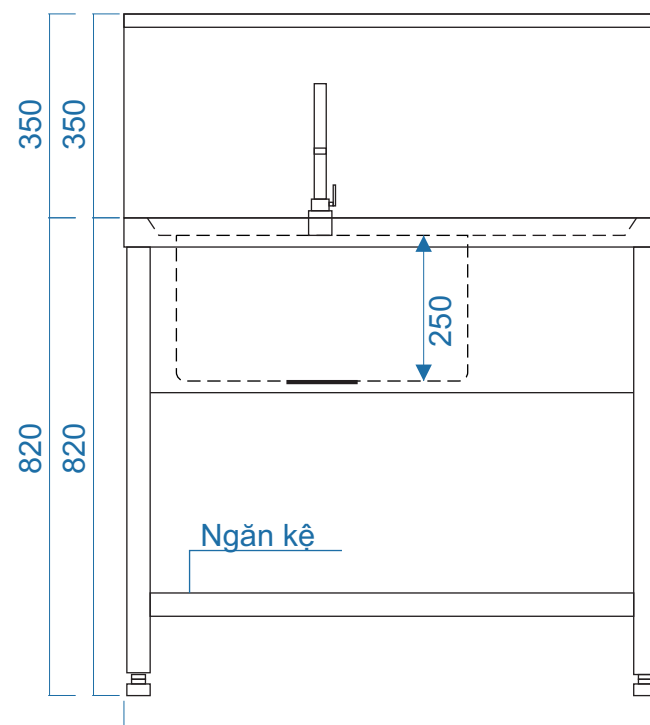
MẶT ĐỨNG
