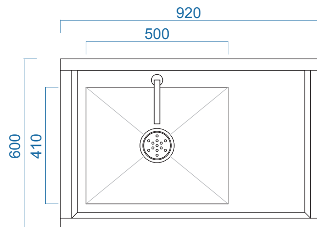
MẶT BẰNG
