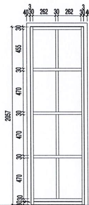
KHUNG CÁNҺ CỬA
