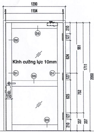
MẶT ĐÚNG NGOÀI
