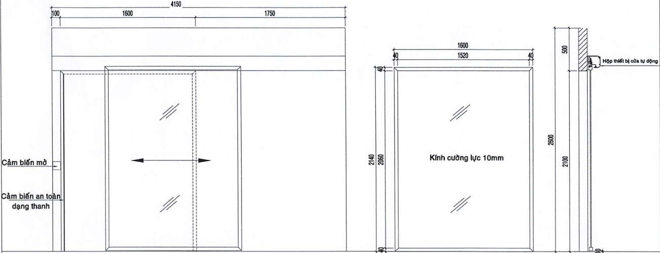
MẶT ĐÚNG CỬA TỰ ĐỘNG
