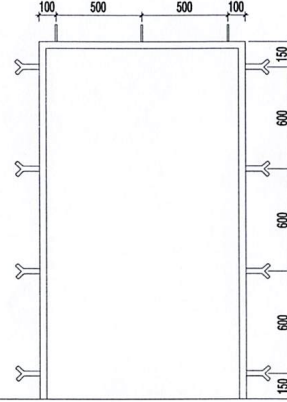
CHI TIẾT NEO KHUNG CỬA
