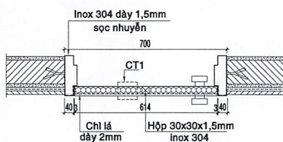
MẶT BẰNG CỬA
