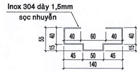
CHI TIẾT KHUNG CỬA
