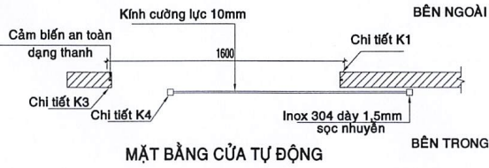
MẶT BẰNG CỬA TỰ ĐỘNG
