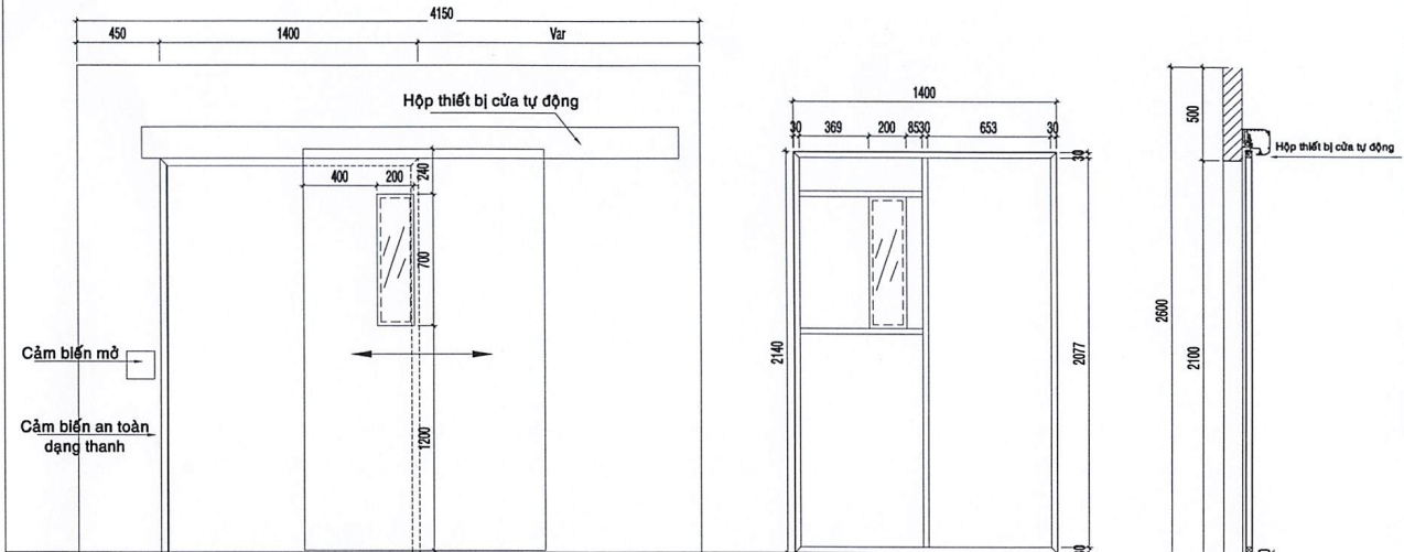
MẶT ĐÚNG CỬA TỰ ĐỘNG
