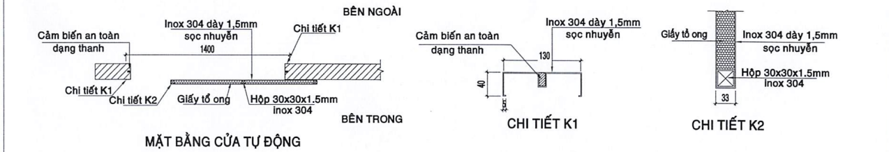
MẶT BẰNG CỬA TỰ ĐỘNG
