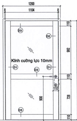
MẶT ĐÚNG TRONG
