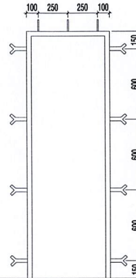
CHI TIẾT NEO KHUNG CỬA
