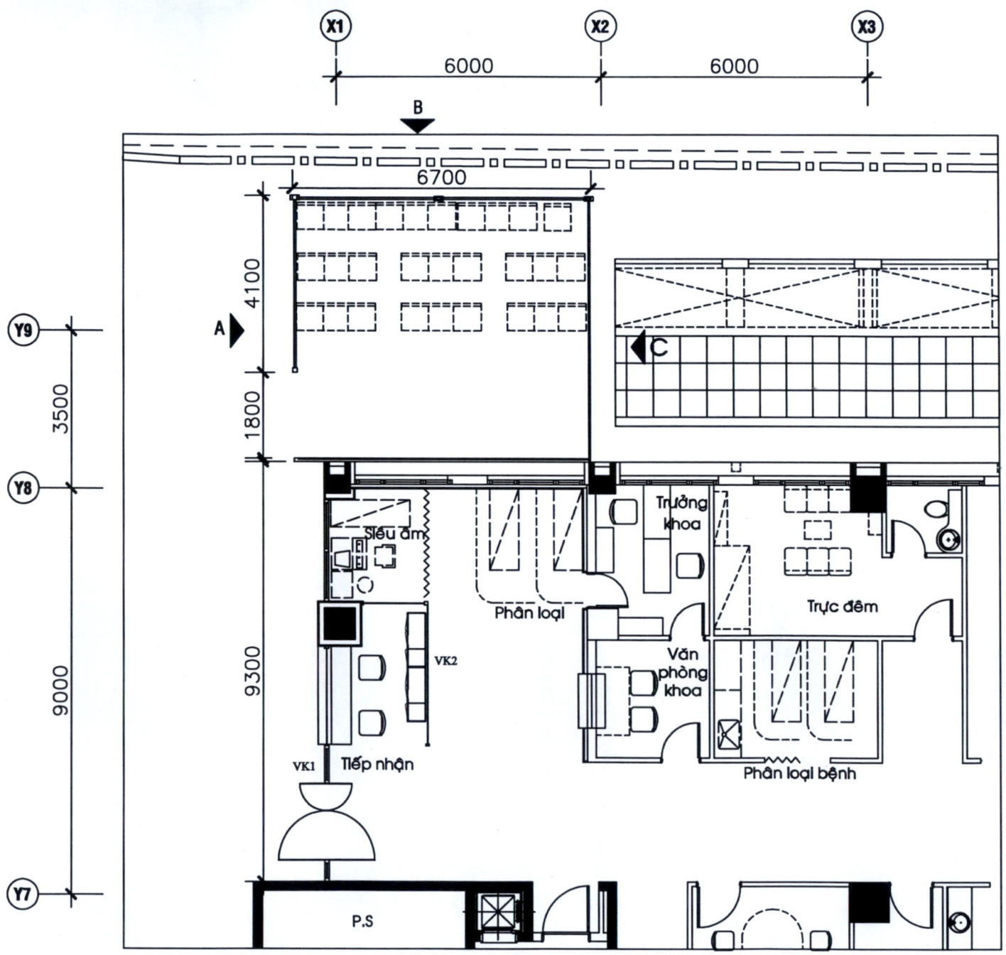
MẶT BẰNG KHU VỰC NGỒI CHỜ VÀ TIẾP NHẬN KHOA CẤP CỨU SAU CẢI TẠO
