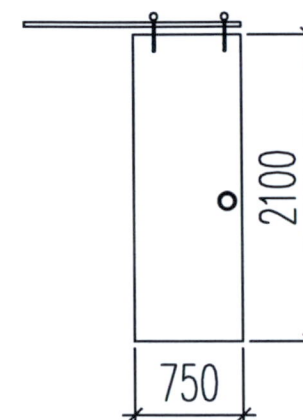
CHI TIẾT CỬA LÙA
