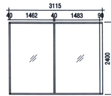
MẶT CHIỀU ĐỨNG HƯỚNG NHÌN 2 VÁCH VK2
