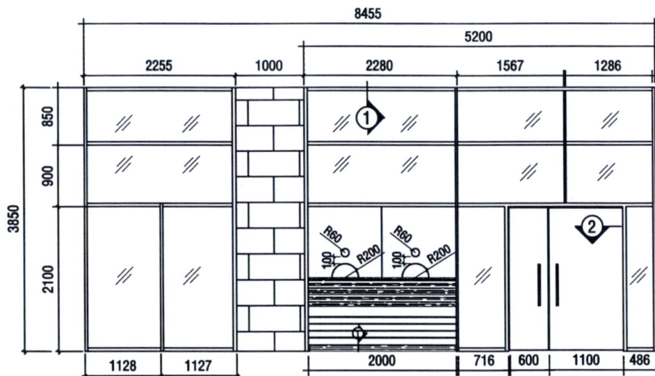
MẶT ĐỨNG KHUNG INOX VÁCH KÍNH VK1
