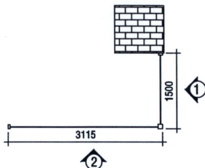
MẶT BẰNG KHUNG INOX VÁCH KÍNH VK2
