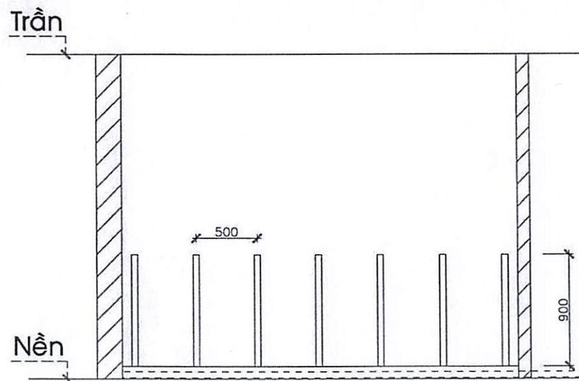
CHI TIẾT BỐ TRÍ KHUNG XƯƠNG
