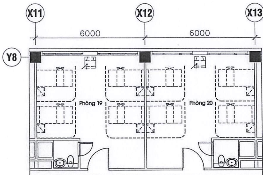
MẶT BẰNG LẦU 7 TRƯỚC KHI CẢI TẠO
