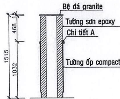
CHI TIẾT TƯỜNG LỮNG
