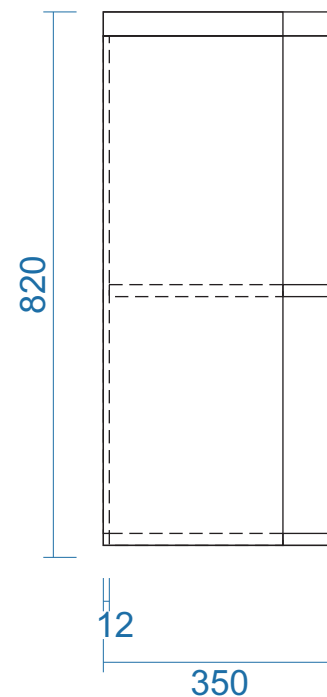
MẶT BÊN
