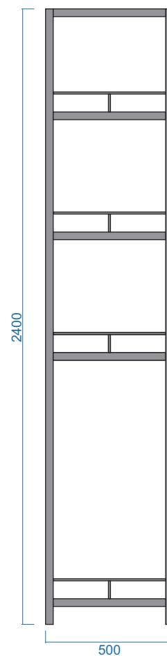
MẶT BÊN
