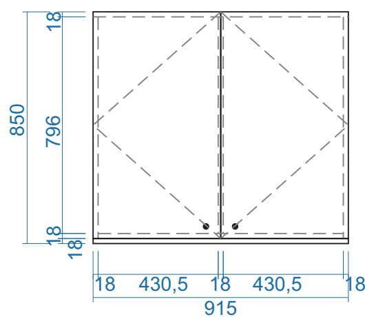
MẶT ĐỨNG
