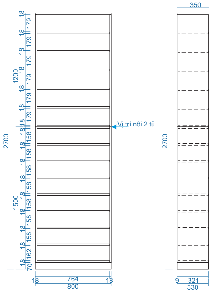
MẶT ĐỨNG
