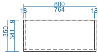
MẶT BẰNG
