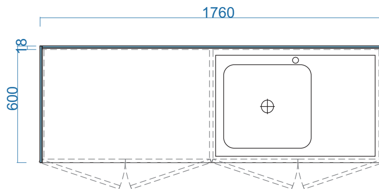
MẶT BẰNG
