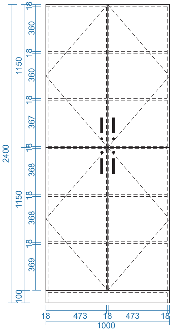
MẶT ĐỨNG
