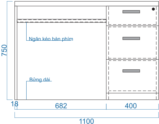
MẶT ĐỨNG
