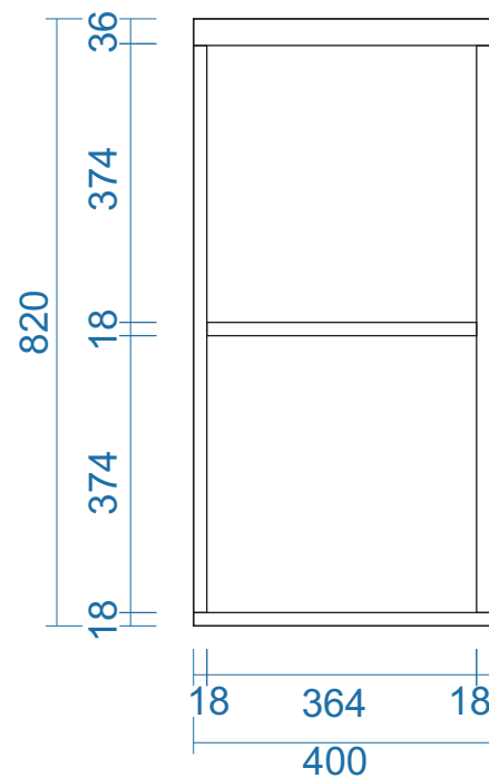
MẶT ĐỨNG
