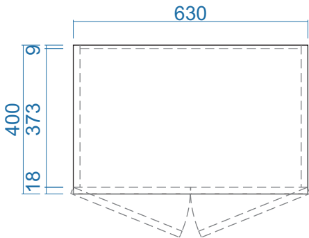
MẶT BẰNG
