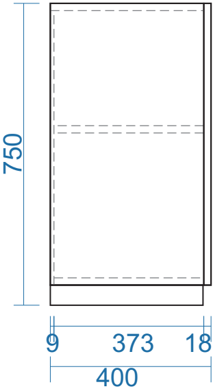
MẶT BÊN
