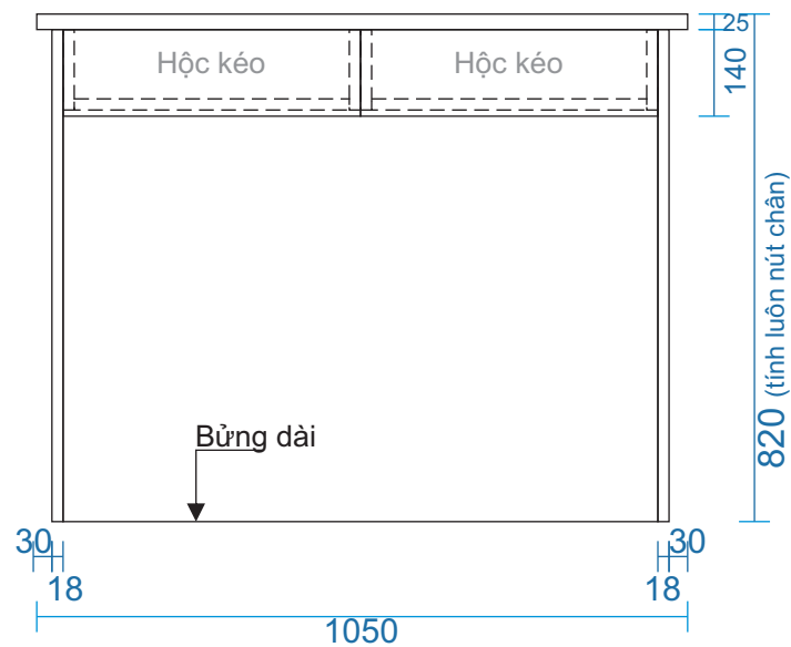
MẶT ĐỨNG
