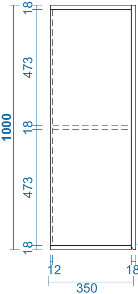
MẶT BÊN
