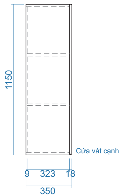
MẶT BÊN
