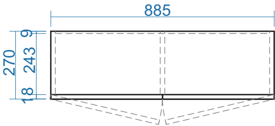
MẶT BẰNG
