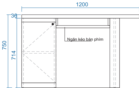
MẶT ĐỨNG
