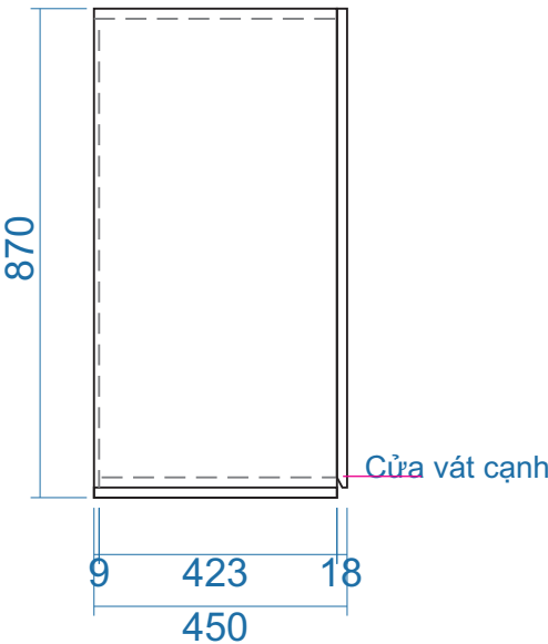
MẶT BÊN
