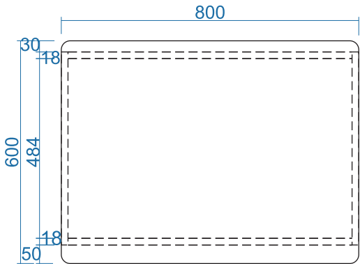
MẶT BẰNG
