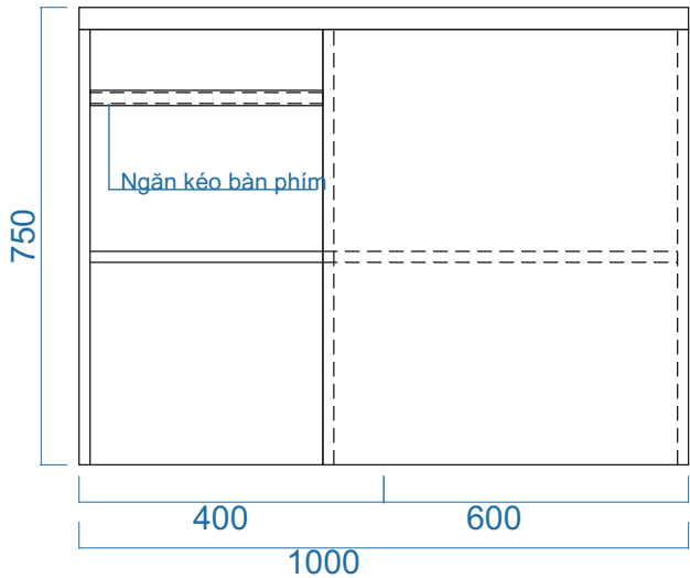
MẶT ĐỨNG
