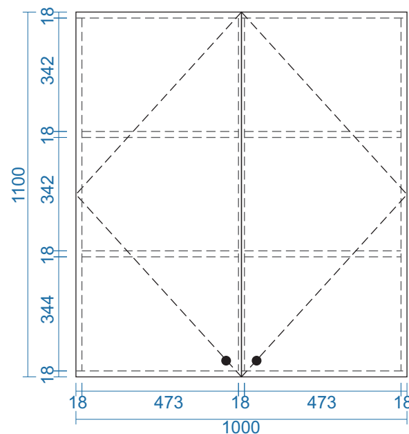
MẶT ĐỨNG
