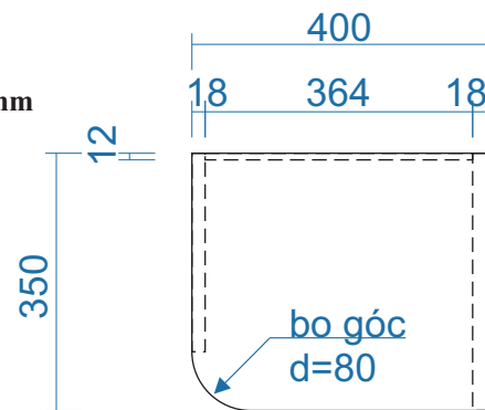
MẶT BỀ
