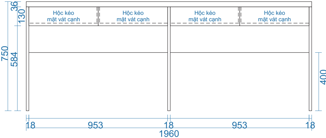
MẶT ĐỨNG
