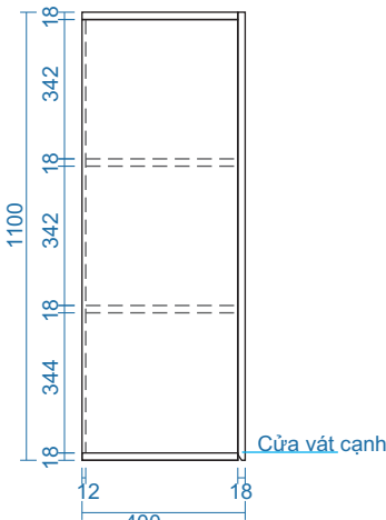
MẶT BÊN
