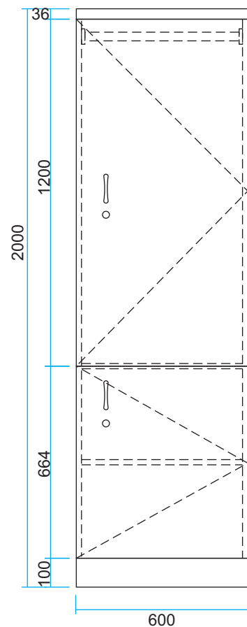
MẶT ĐỨNG
