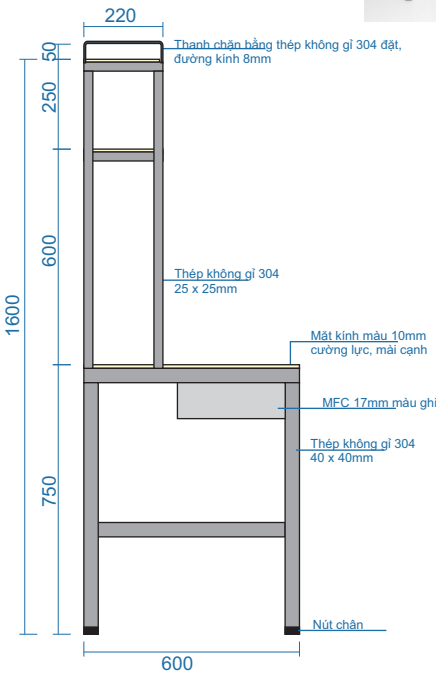
MẶT BÊN
