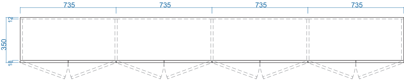
MẶT BẰNG
