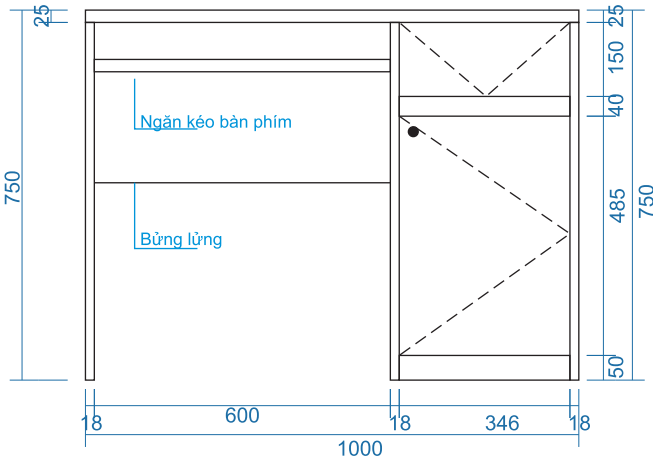
MẶT ĐỨNG
