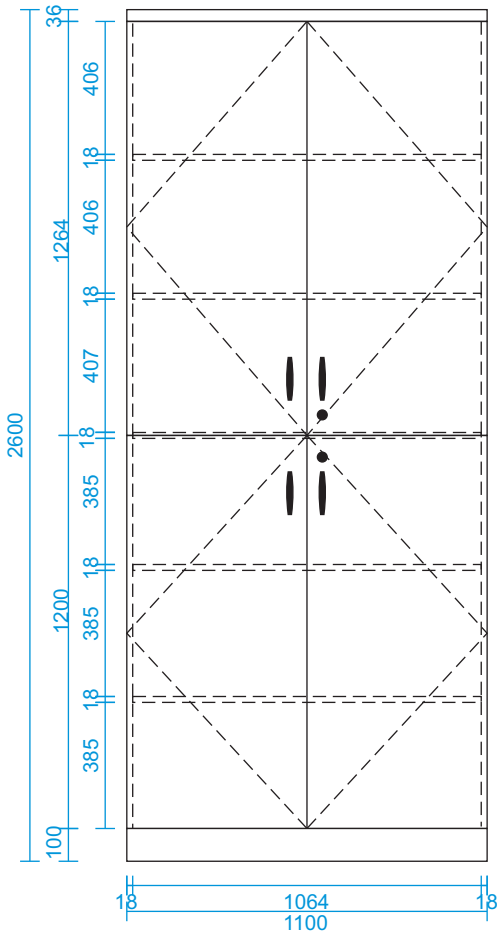
MẶT ĐỨNG
