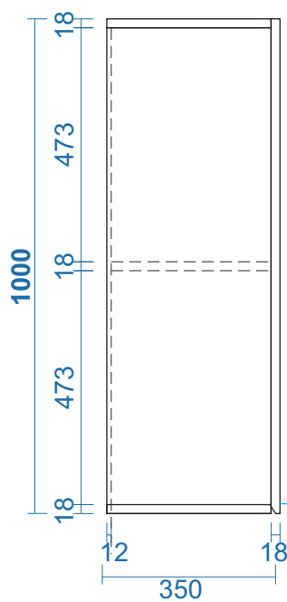
MẶT BÊN
