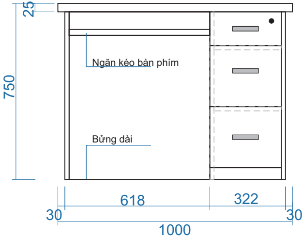
MẶT ĐỨNG
