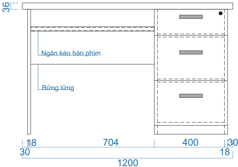
MẶT ĐỨNG
