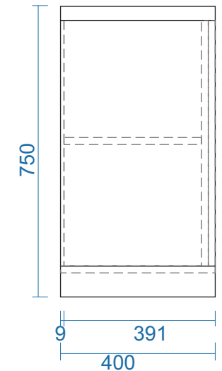
MẶT BÊN
