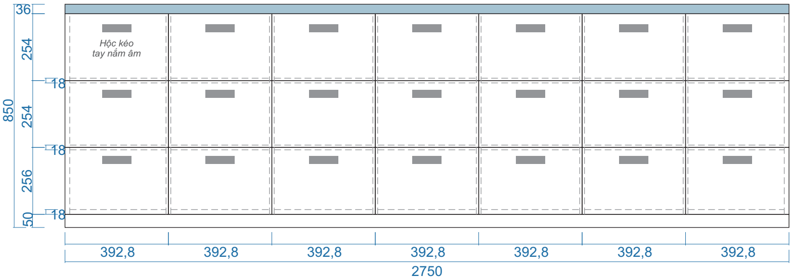
MẶT ĐỨNG
