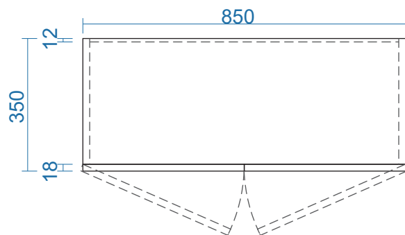
MẶT BẰNG
