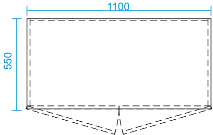
MẶT BẰNG
