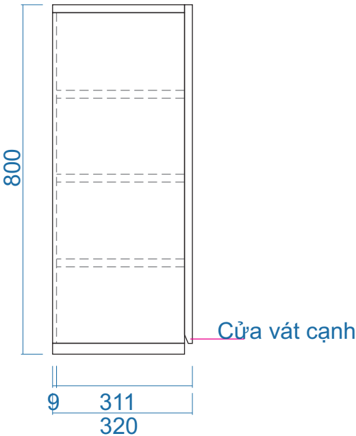
MẶT BÊN
