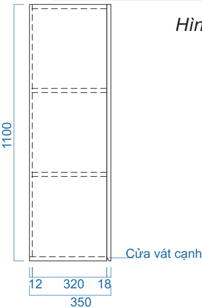
MẶT BÊN
