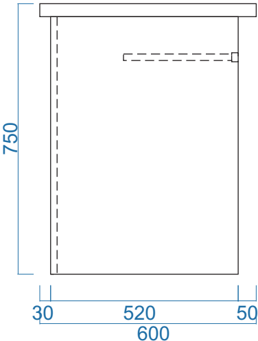
MẶT BÊN
