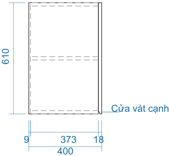
MẶT BÊN
