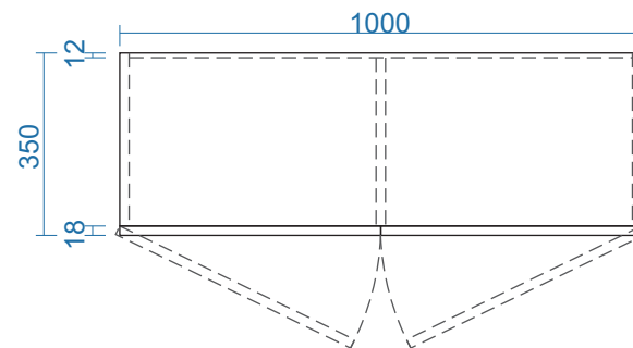
MẶT BẰNG
