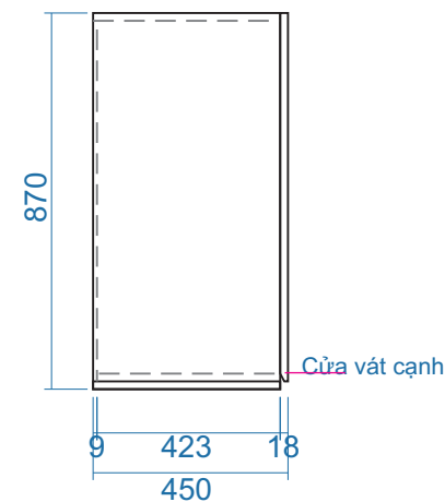
MẶT BÊN
