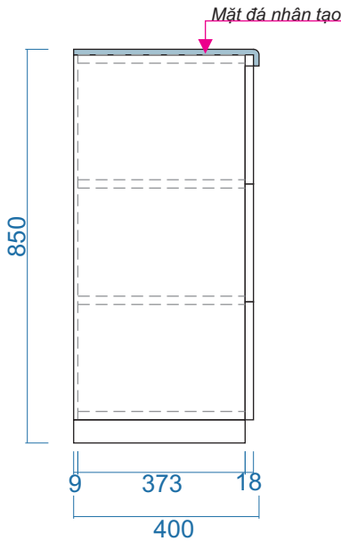
MẶT BÊN
