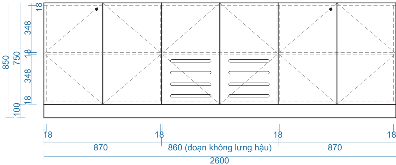
MẶT ĐỨNG
