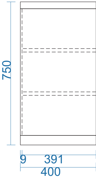
MẶT BÊN
