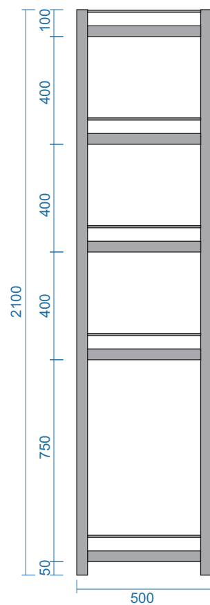
MẶT ĐỨNG
