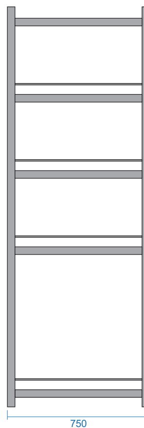
MẶT BÊN
