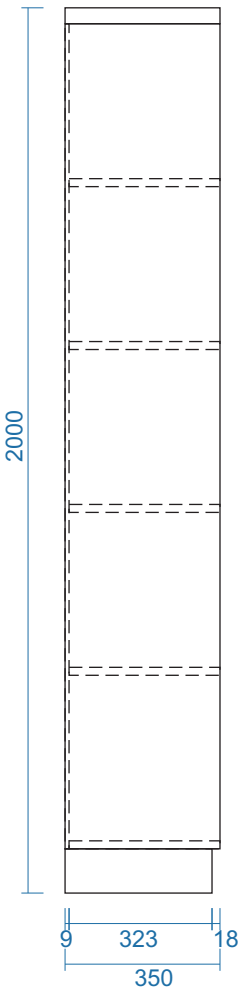
MẶT BÊN
