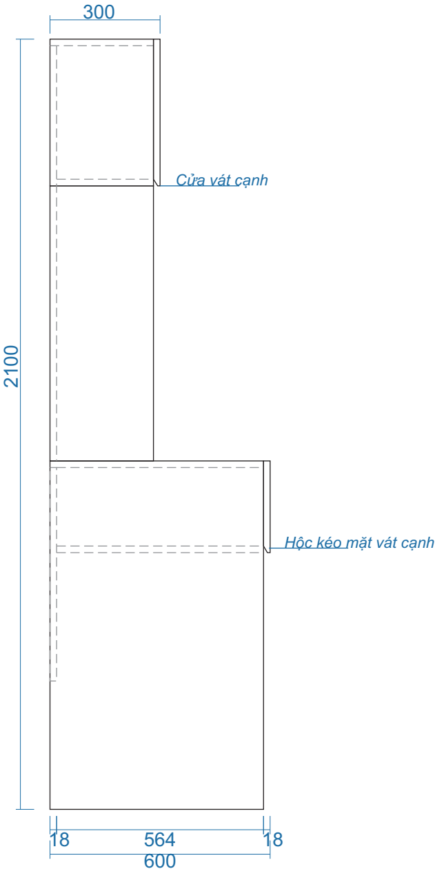
MẶT BÊN
