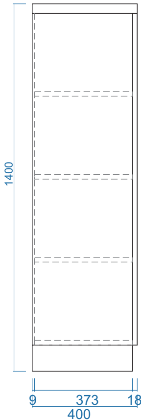
MẶT BÊN
