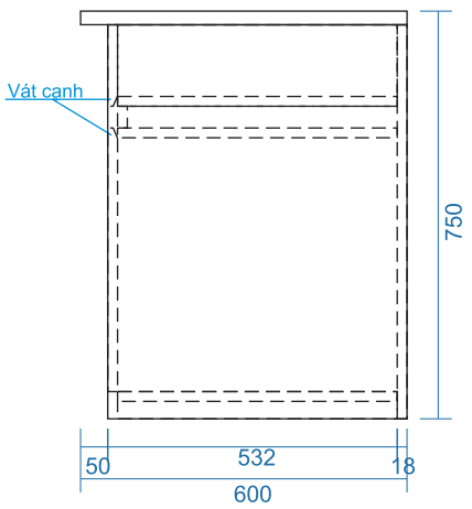
MẶT BÊN
