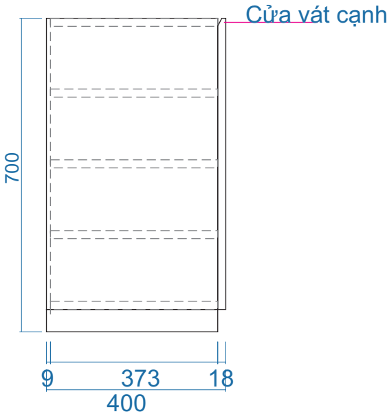
MẶT BÊN
