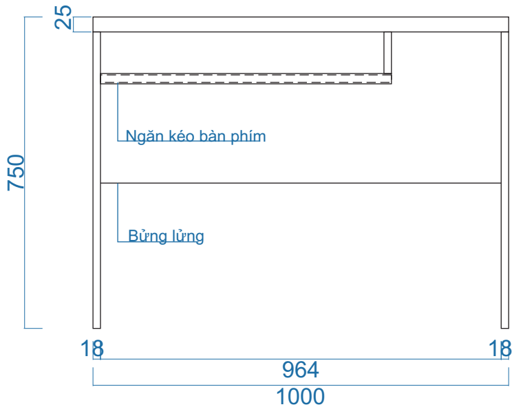
MẶT ĐỨNG
