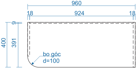
MẶT BẰNG
