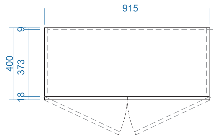
MẶT BẰNG
