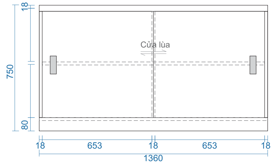
MẶT ĐỨNG
