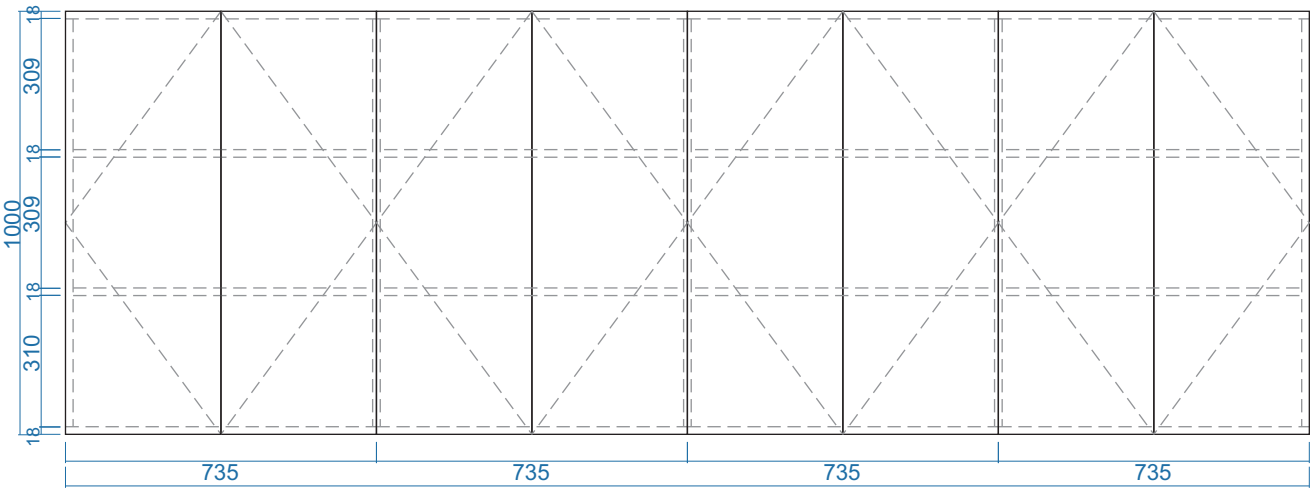
MẶT ĐỨNG
