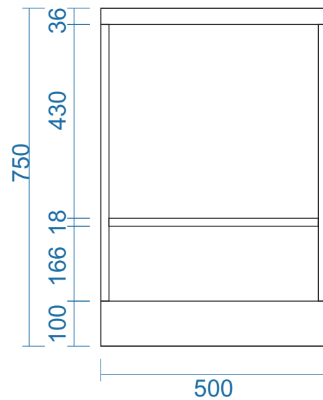
MẶT ĐỨNG
