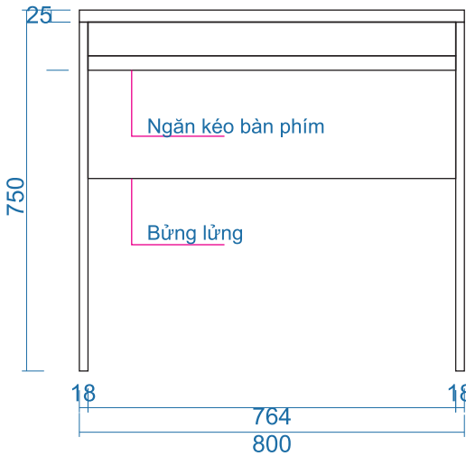
MẶT ĐỨNG
