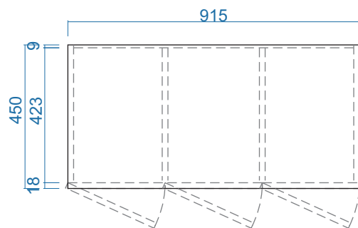
MẶT BẰNG
