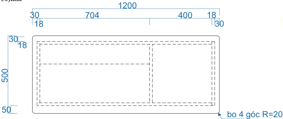
MẶT BẰNG
