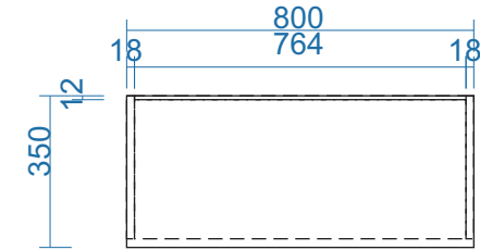
MẶT BẰNG
