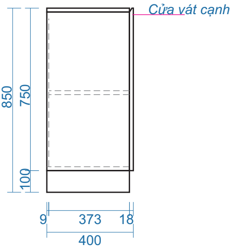
MẶT BÊN
