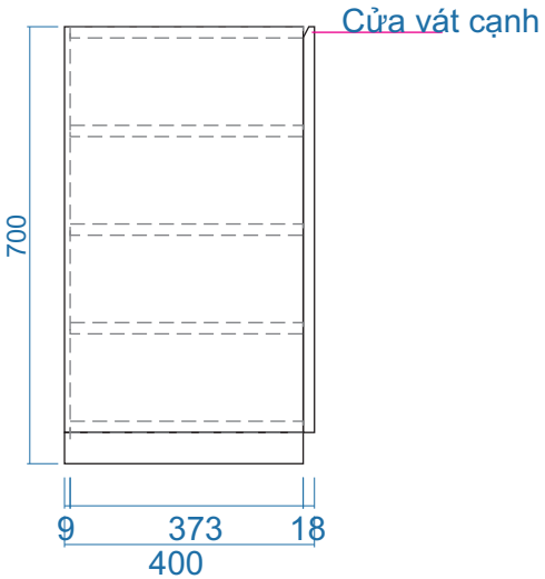
MẶT BÊN
