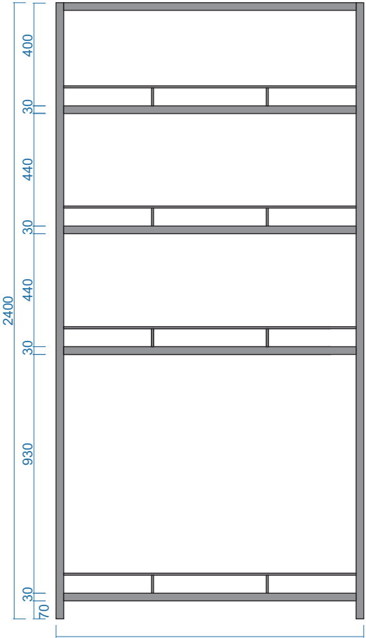
MẶT ĐỨNG
