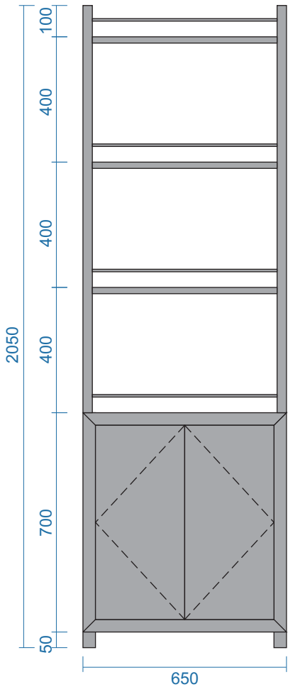
MẶT ĐỨNG
