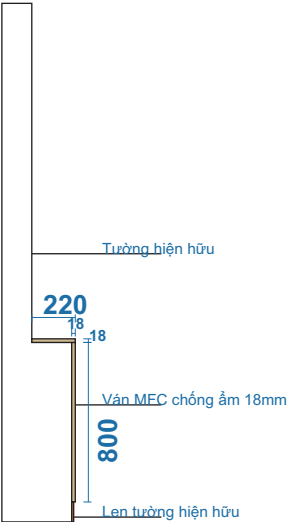
Mặt bên
