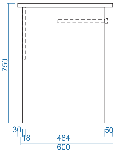
MẶT BÊN
