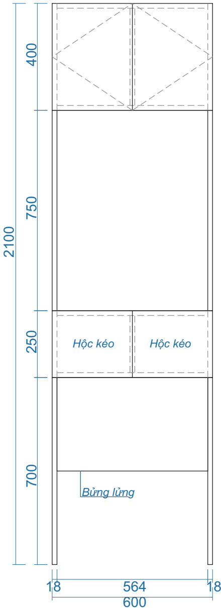
MẶT ĐỨNG
