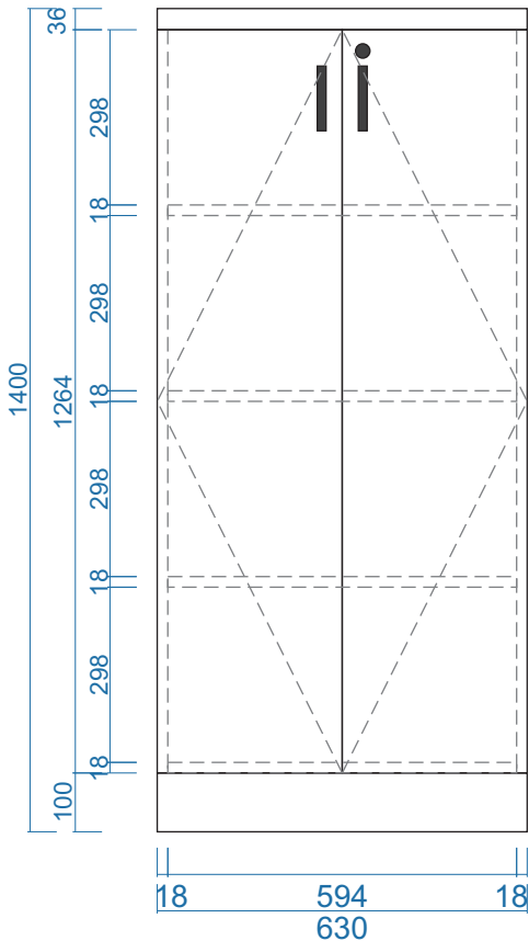
MẶT ĐỨNG
