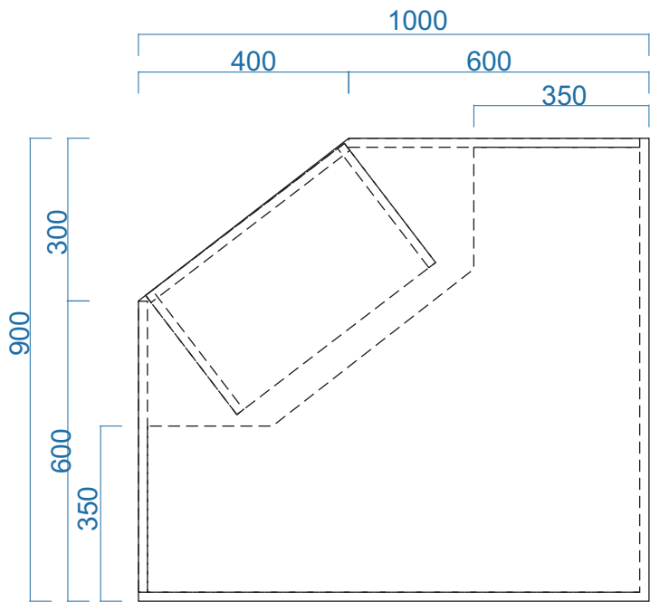
MẶT BẰNG
