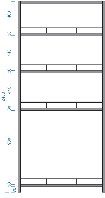
MẶT ĐÚNG
