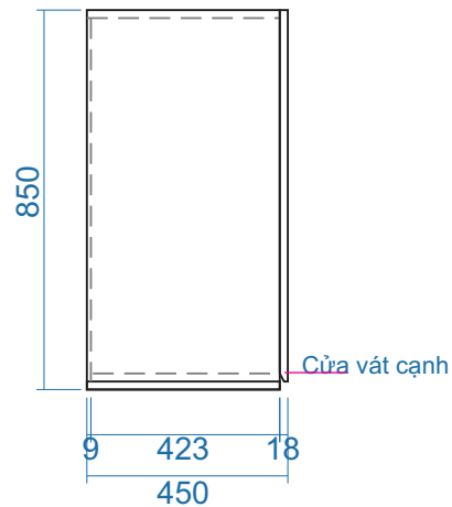
MẶT BÊN
