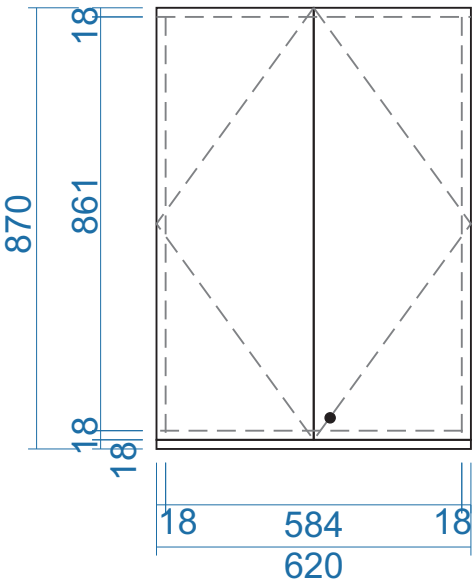
MẶT ĐỨNG
