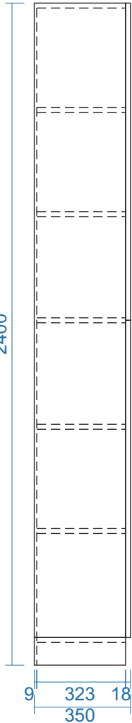
MẶT BÊN
