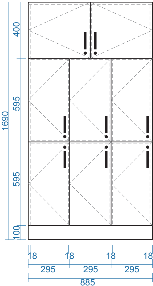
MẶT ĐỨNG
