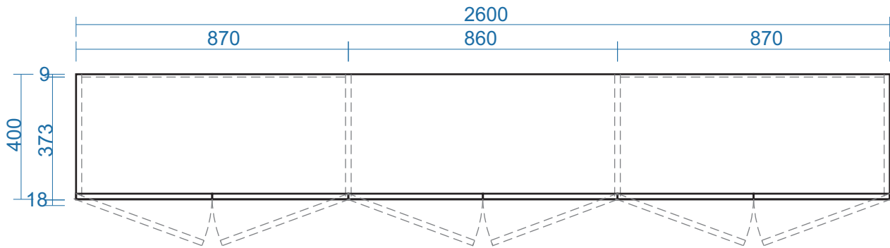
MẶT BẰNG
