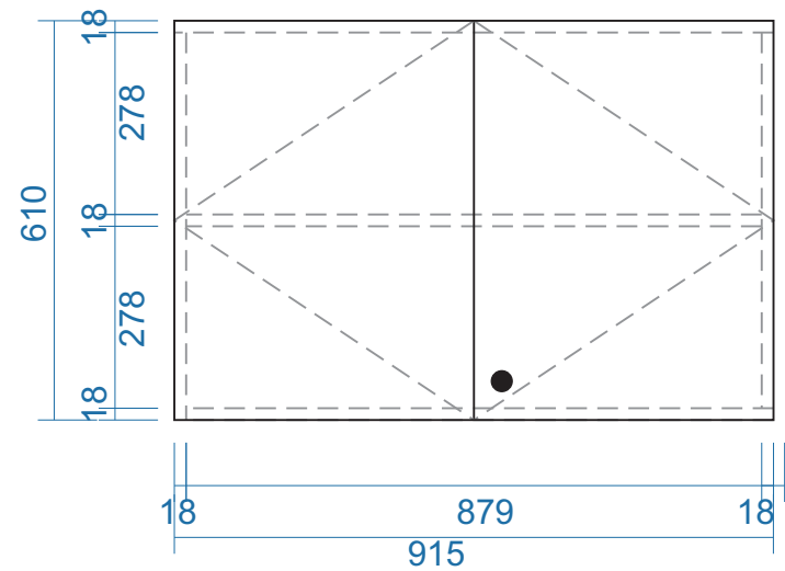
MẶT ĐỨNG
