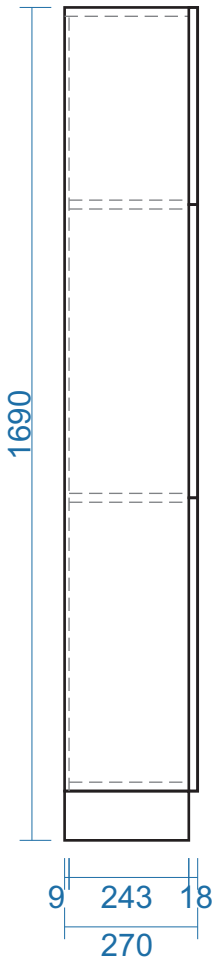
MẶT BÊN
