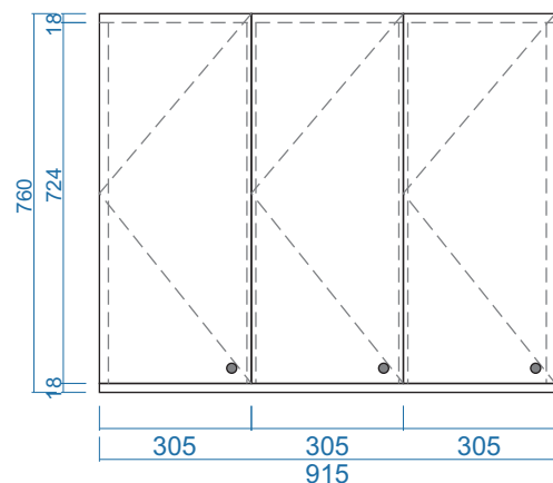
MẶT ĐỨNG
