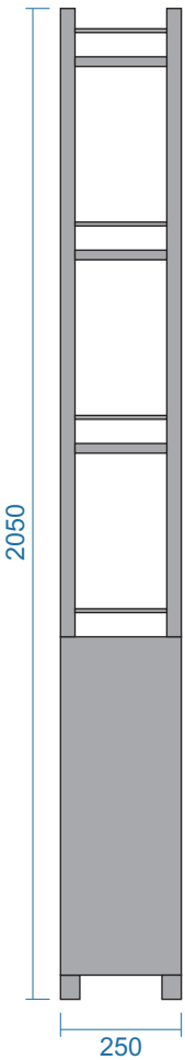
MẶT BÊN
