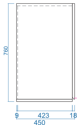
MẶT BÊN
