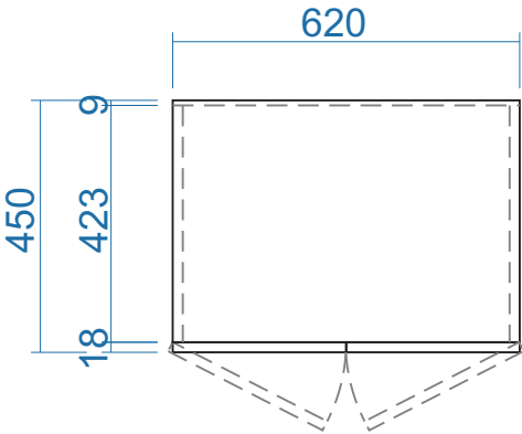
MẶT BẰNG
