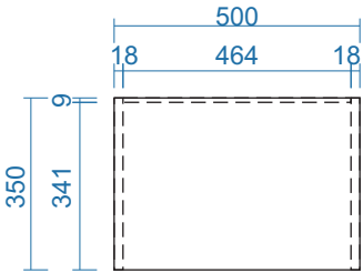
MẶT BẰNG
