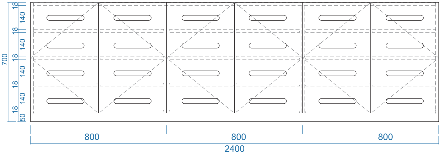
MẶT ĐỨNG
