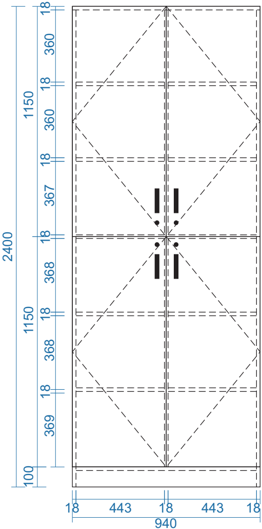
MẶT ĐỨNG
