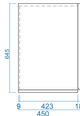
MẶT BÊN
