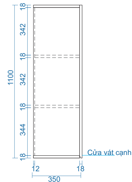
MẶT BÊN
