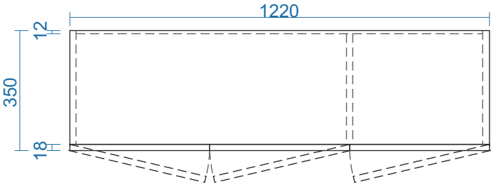
MẶT BẰNG
