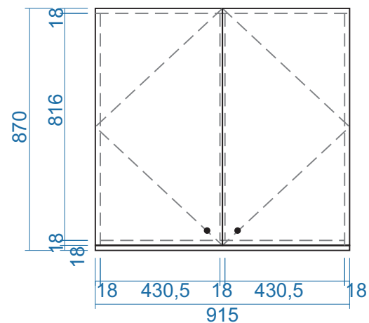
MẶT ĐỨNG
