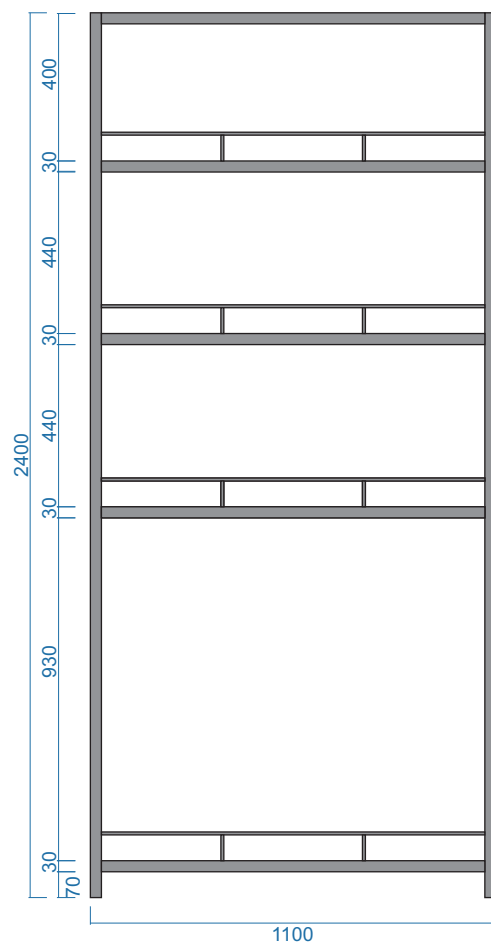
MẶT ĐỨNG
