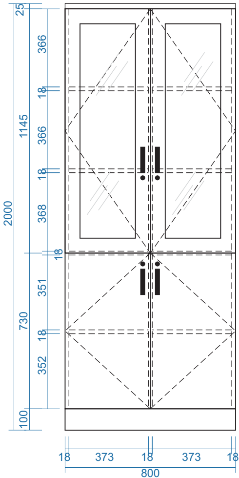
MẶT ĐỨNG
