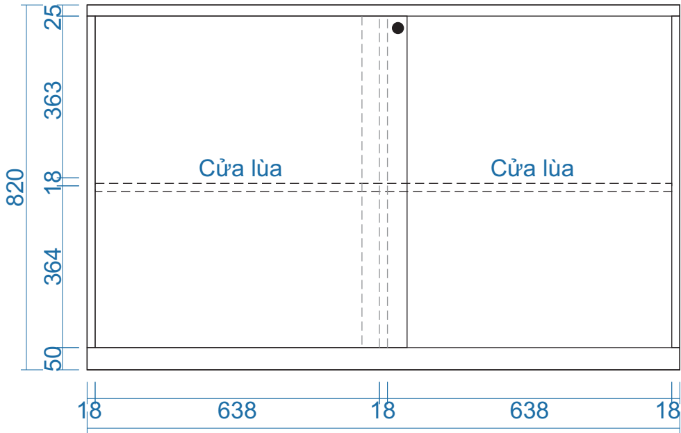
MẶT ĐỨNG
