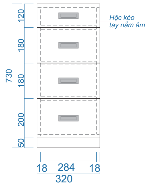
MẶT ĐỨNG
