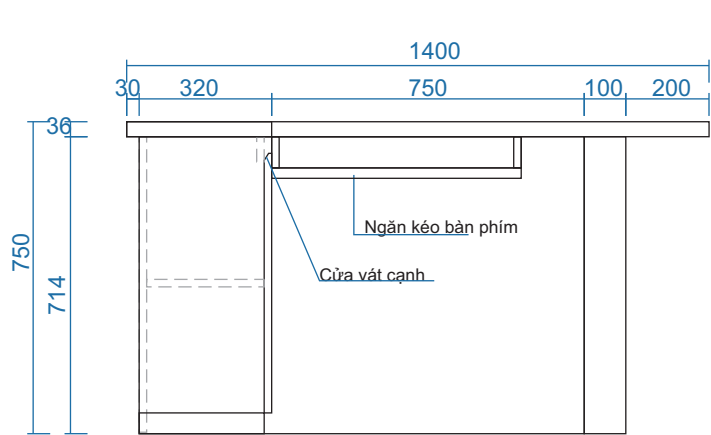
MẶT ĐỨNG
