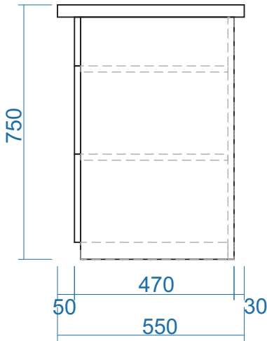
MẶT BÊN
