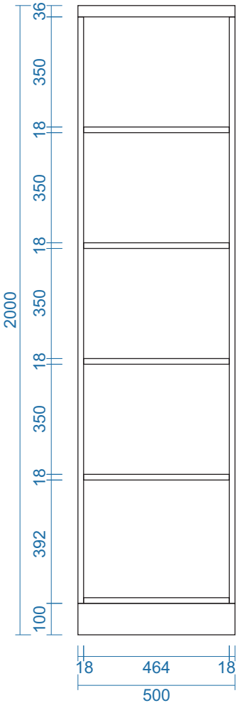
MẶT ĐỨNG
