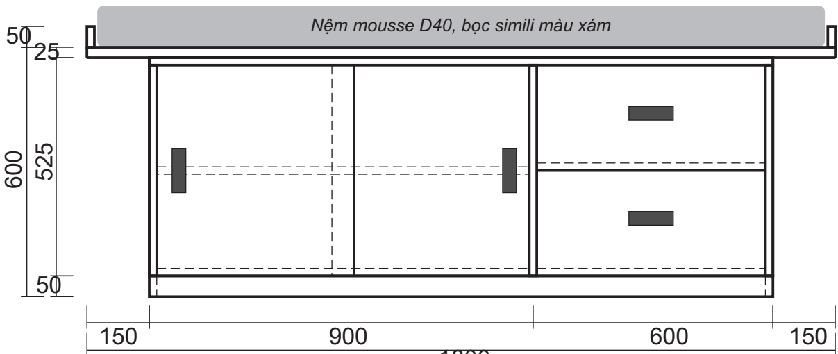
MẶT ĐỨNG
