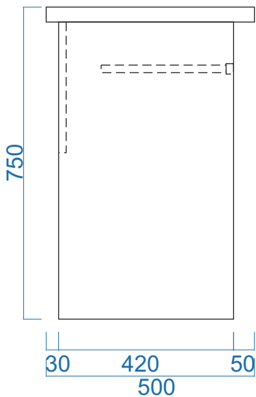
MẶT BÊN
