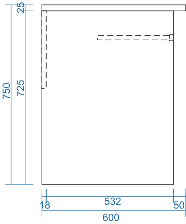
MẶT BÊN
