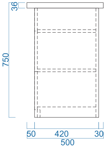
MẶT BÊN
