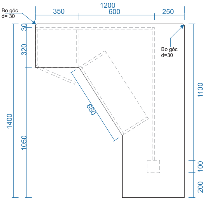
MẶT BẰNG
