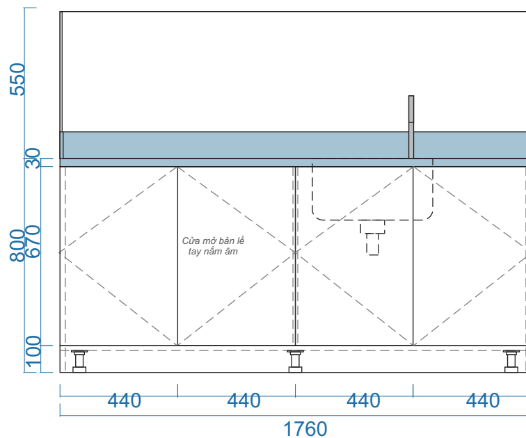
MẶT ĐỨNG
