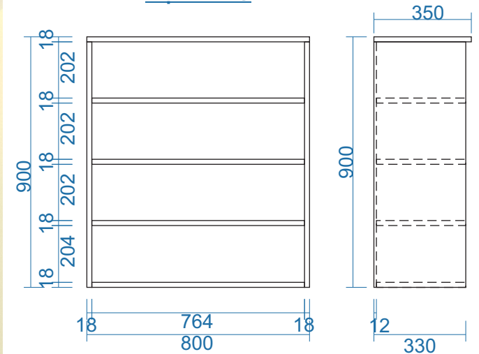
MẶT ĐỨNG
