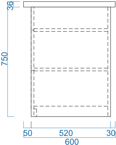
MẶT BÊN
