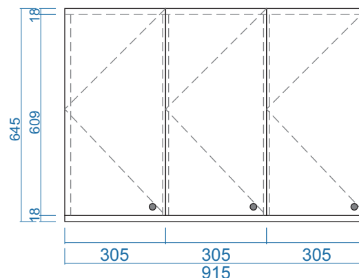
MẶT ĐỨNG
