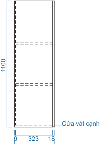
MẶT ĐÚNG
