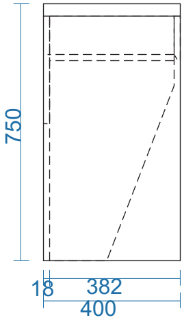
MẶT BÊN
