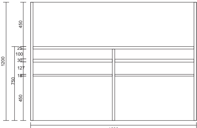
MẶT SAU
