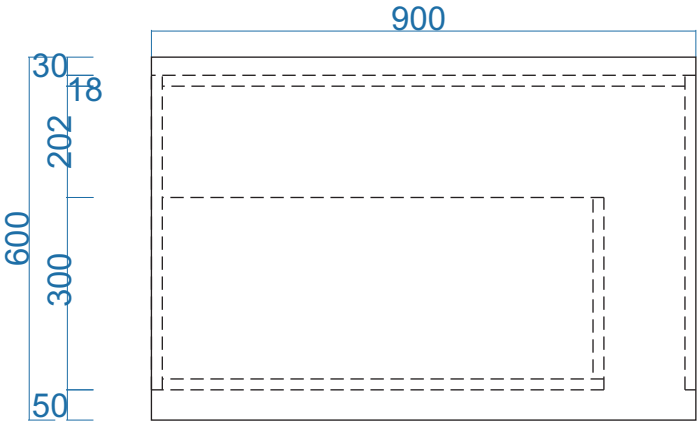
MẶT BẰNG
