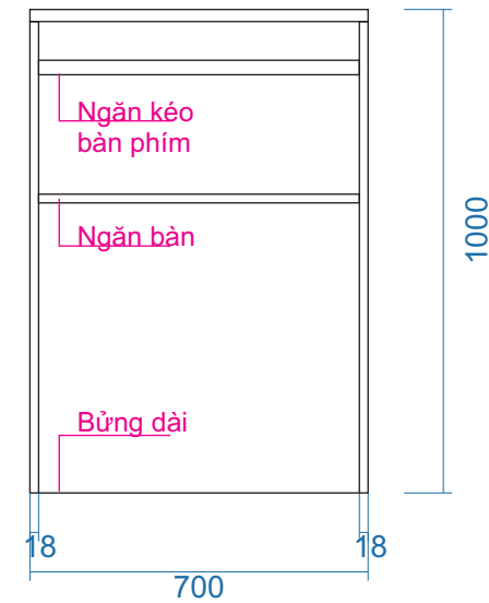
MẶT ĐỨNG
