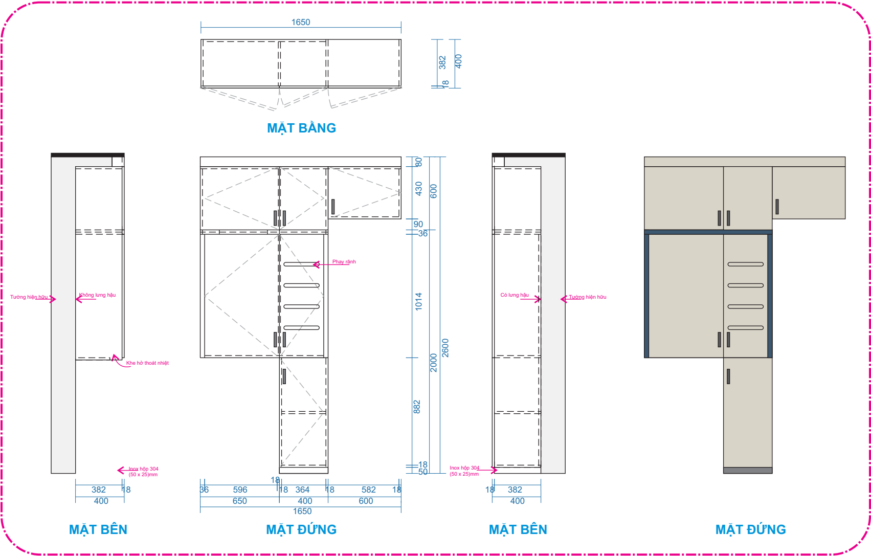
Chi tiết 2
