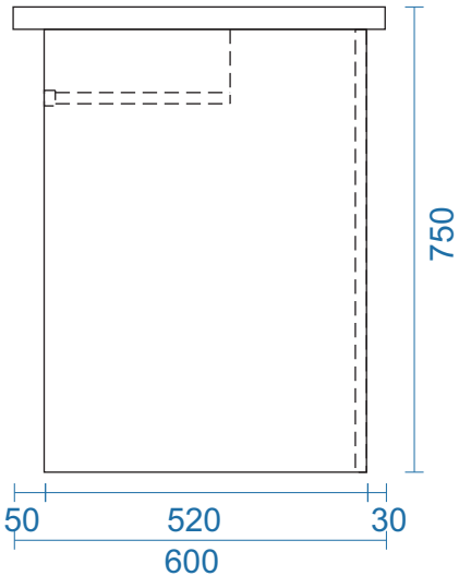
MẶT BÊN
