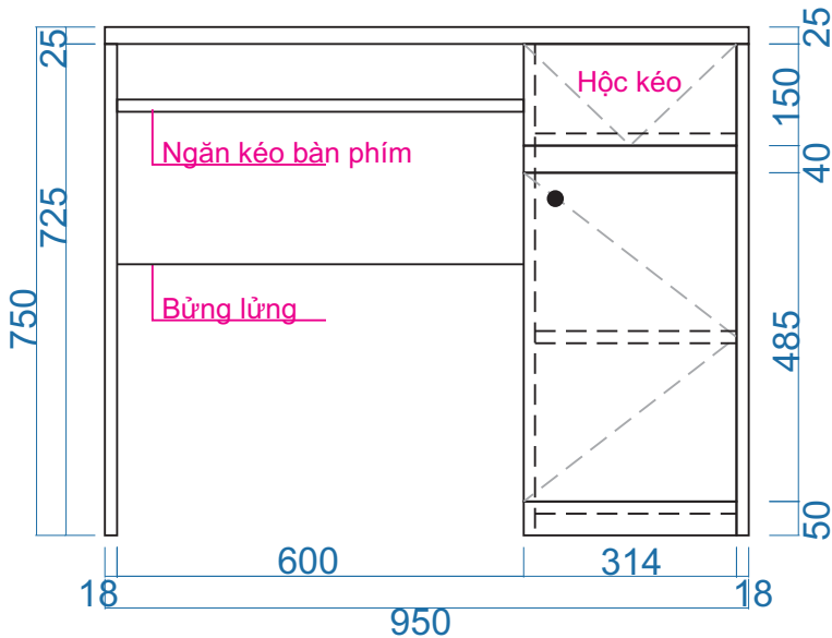
MẶT ĐỨNG
