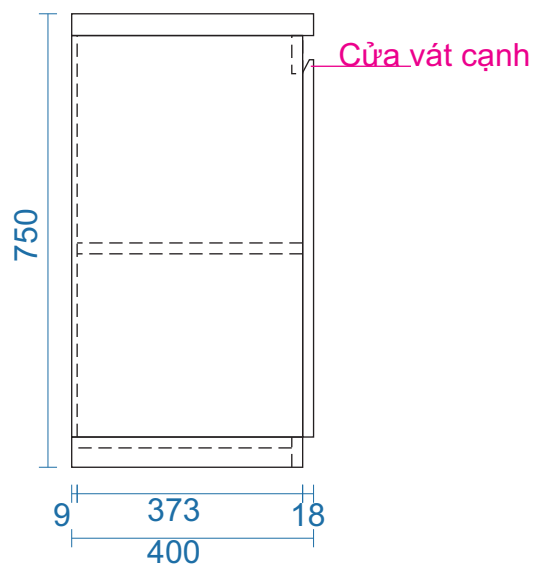
MẶT BÊN
