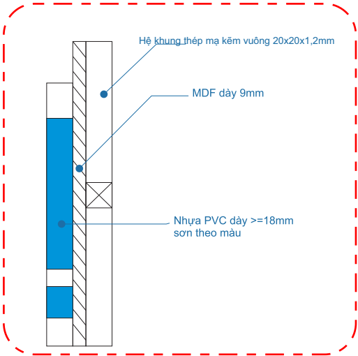
Chi tiết 2
