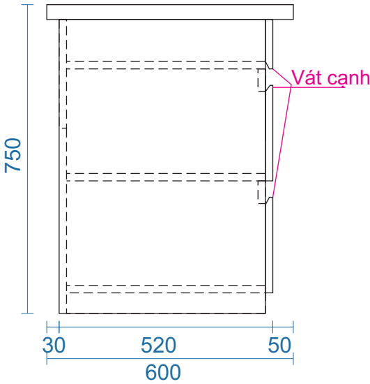
MẶT BÊN
