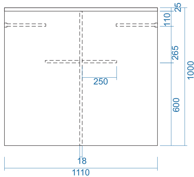
MẶT BÊN
