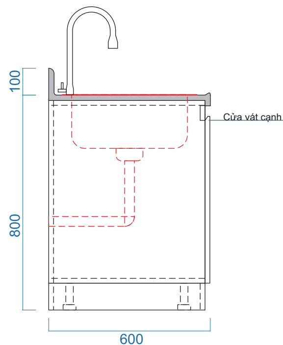
MẶT BÊN
