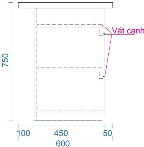
MẶT BÊN
