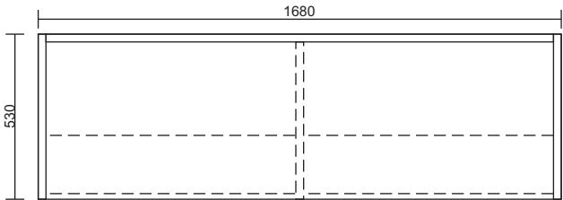
MẶT TRÊN
