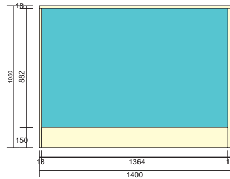
VÁCH 1
