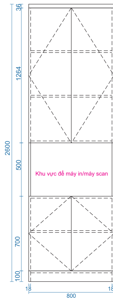
MẶT ĐỨNG
