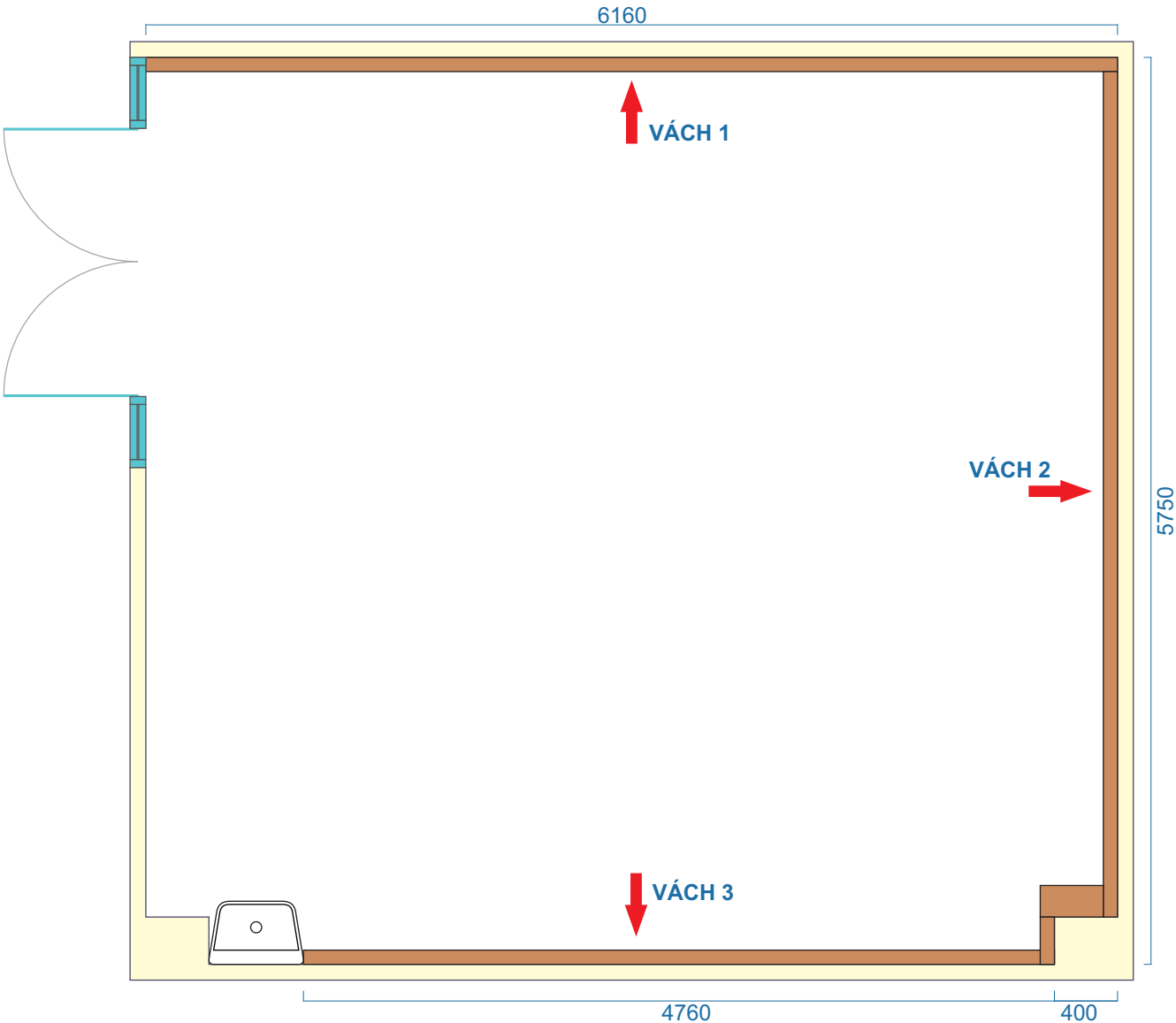
MẶT BẰNG BỐ TRÍ VÁCH ỐP ĐƯỜNG ỐNG R.O KHOA NỘI THẬN - THẬN NHÂN TẠO - PHÒNG HDF - OUTDOOR CÁNH B LẦU 9
