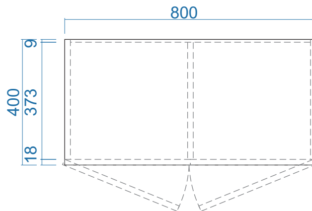
MẶT BẰNG
