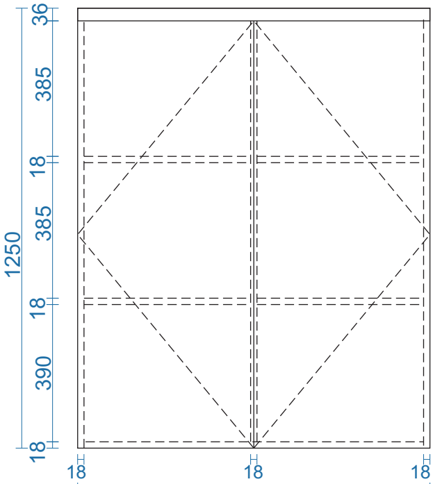
MẶT ĐỨNG
