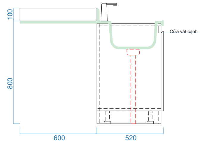
MẶT BÊN
