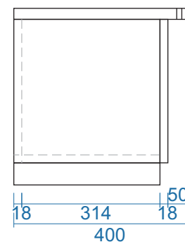
MẶT BÊN
