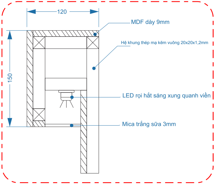
Chi tiết 1
