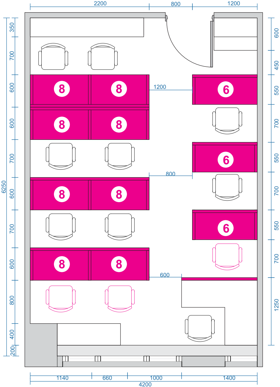
MẶT BẰNG BỐ TRÍ NỘI THẤT PHÒNG QUẢN LÝ CHẤT LƯỢNG BỆNH VIỆN (LẦU 4 KHU A)
