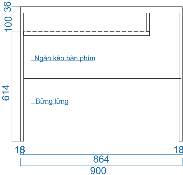
MẶT ĐỨNG
