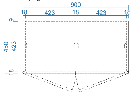
MẶT BẰNG
