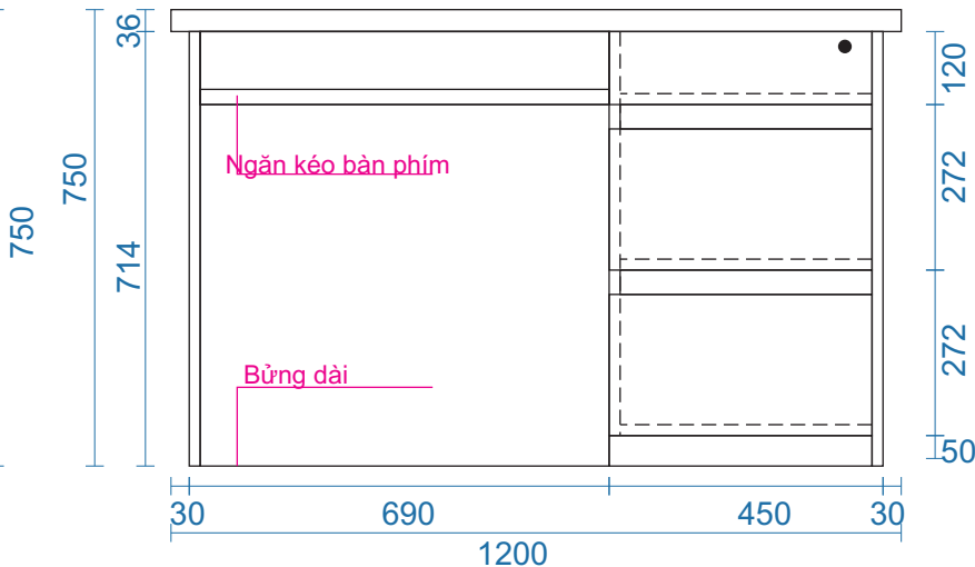
MẶT ĐỨNG
