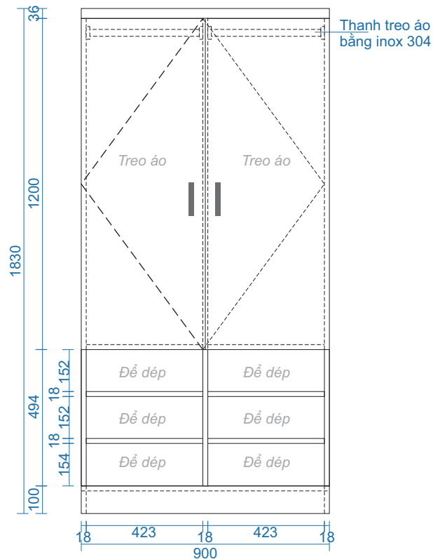
MẶT ĐỨNG
