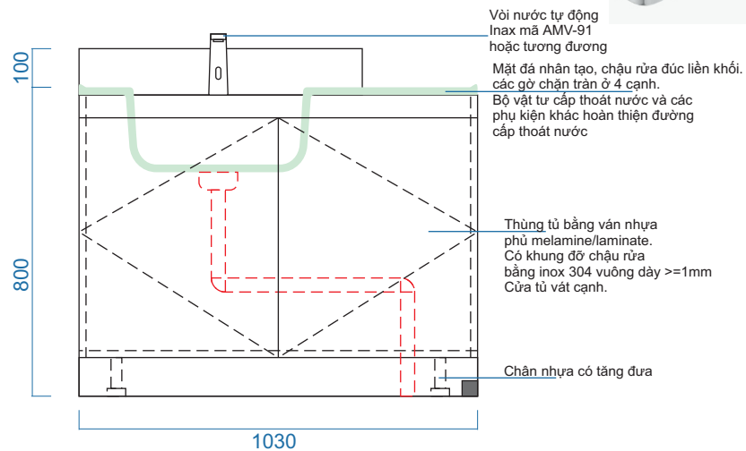
MẶT ĐỨNG
