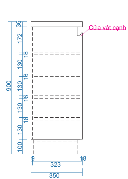
MẶT BÊN
