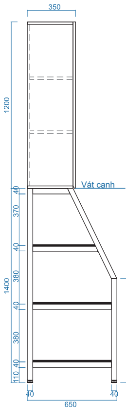
MẶT BÊN
