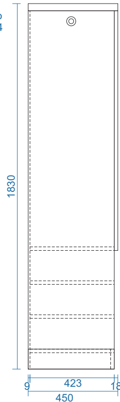
MẶT BÊN
