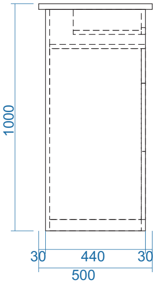
MẶT BÊN
