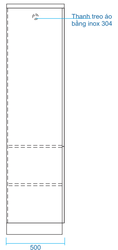
MẶT BÊN
