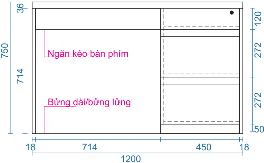
MẶT ĐỨNG
