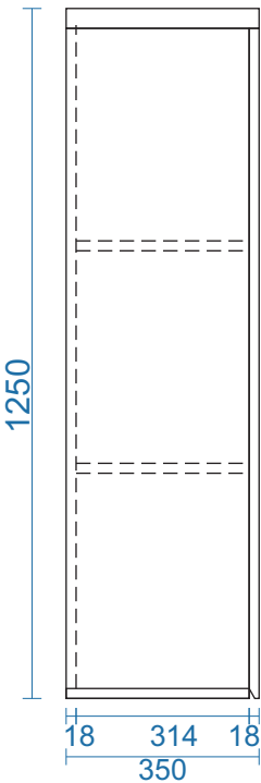
MẶT BÊN
