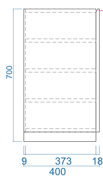
MẶT BÊN
