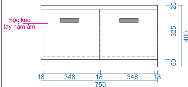
MẶT ĐỨNG
