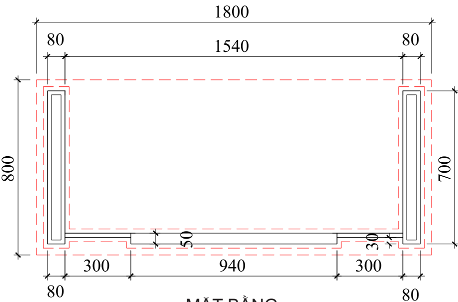
MẶT BẰNG
