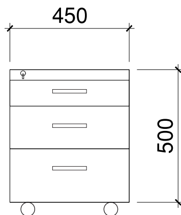
MẶT ĐỨNG
