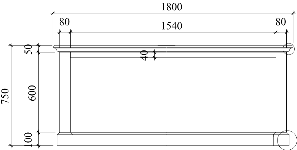
MẶT SAU
