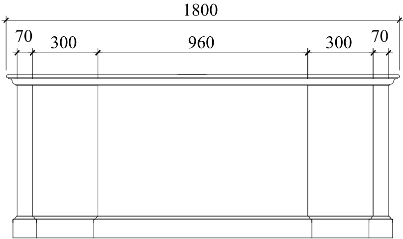
MẶT ĐỨNG
