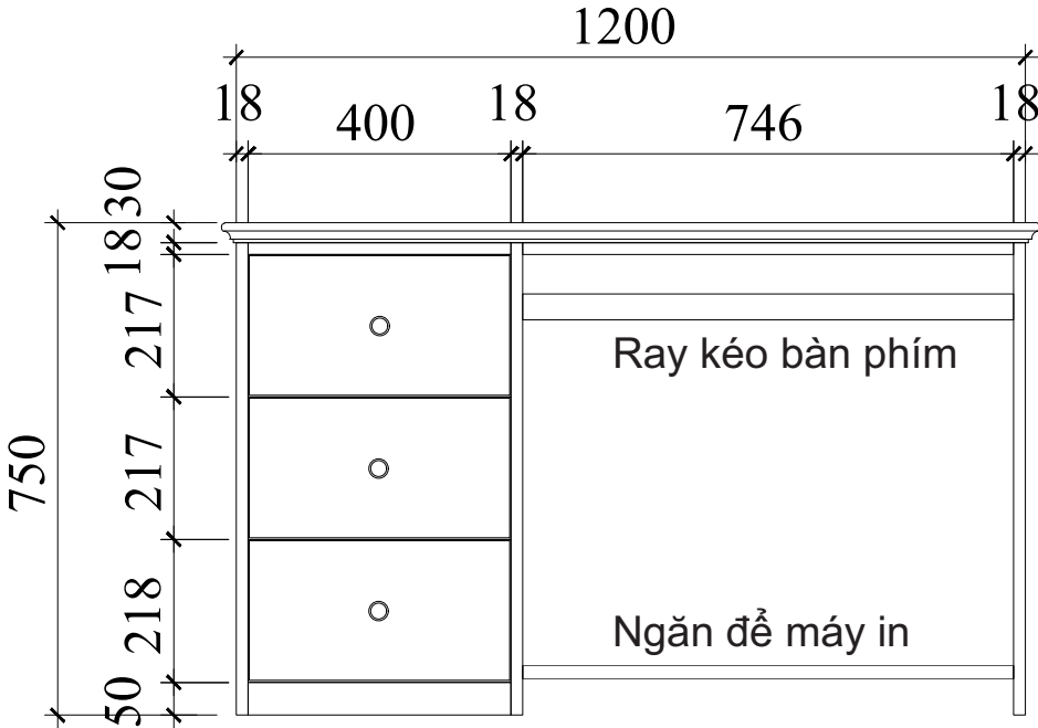
MẶT ĐỨNG
