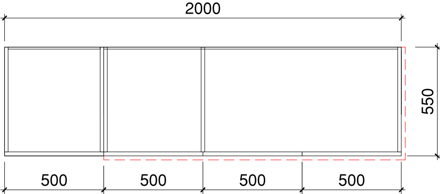
MẶT BẰNG TỦ DƯỚI
