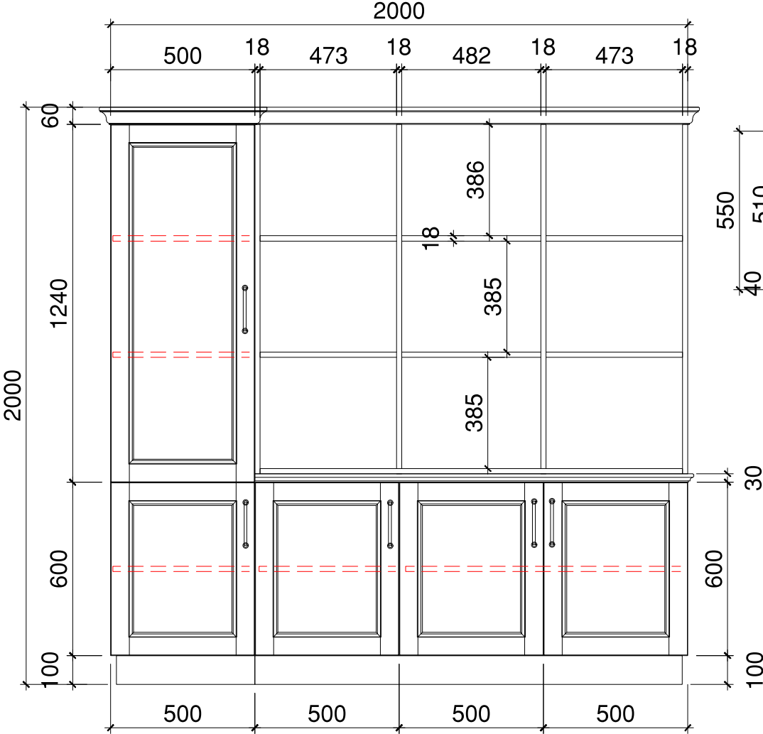
MẶT ĐÚNG TỦ HỒ SƠ
