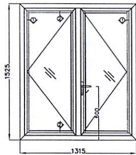
CỬA: WD - 2, SL: 24 BỘ TL 1/80
