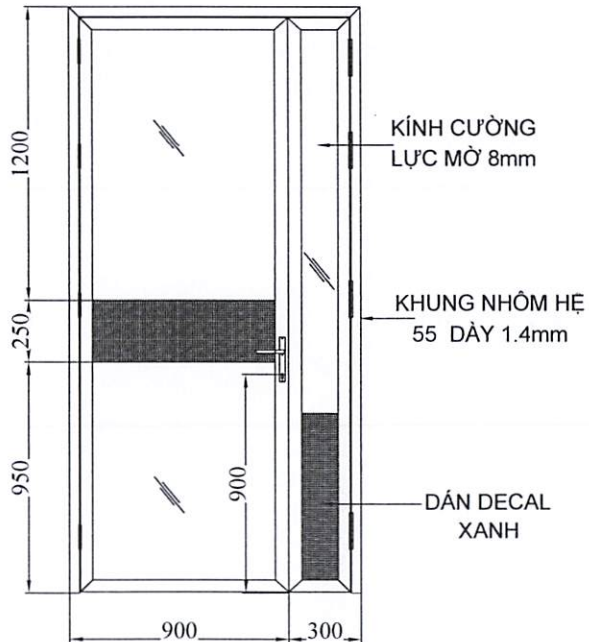
CỬA: MD - 6, SL: 1 BỘ, TL: 1/30
