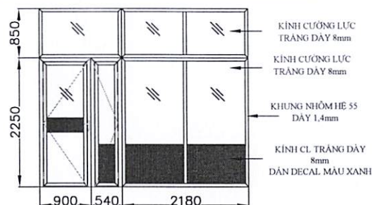
BẢN VẼ MẶT ĐỨNG VÁCH NHÔM THAY MỚI TL 1/90
