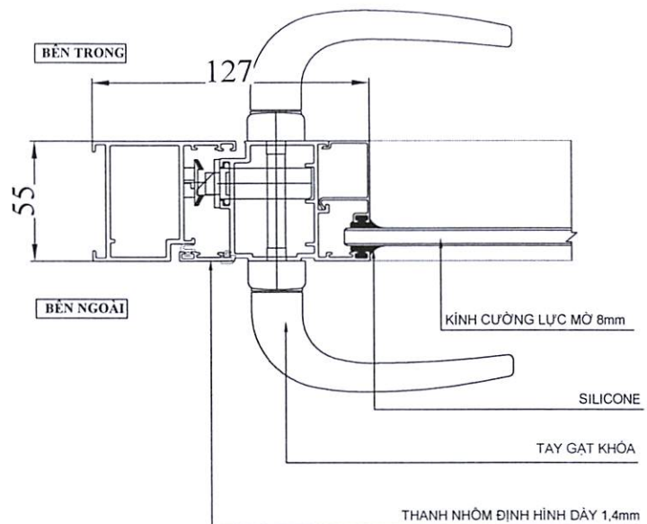
CHI TIẾT 23
