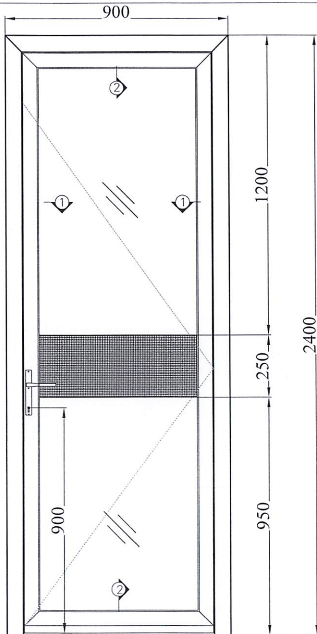
CỬA MD - 10
