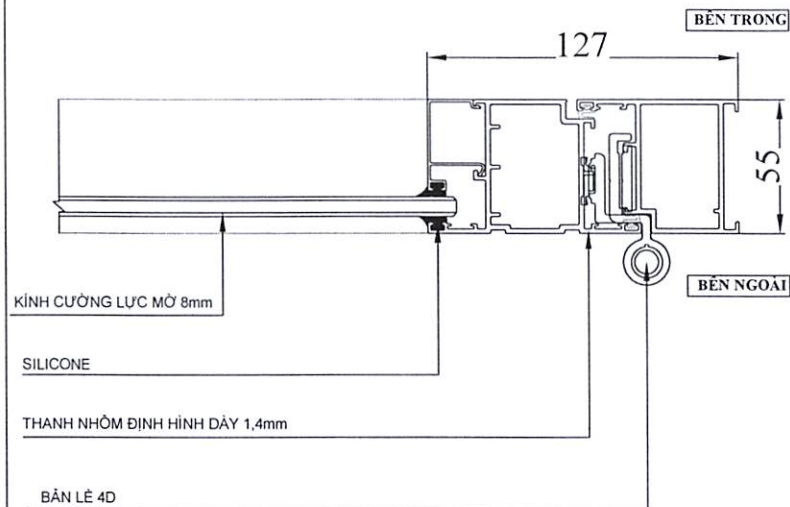
CHI TIẾT 16
