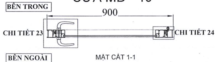
CỬA MD - 10
