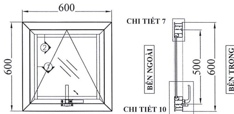
CỬA WD - 5
