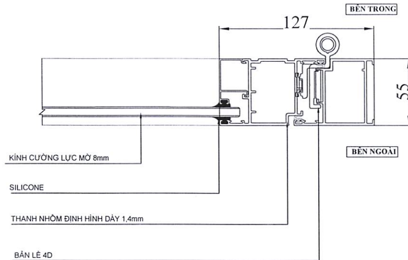
CHI TIẾT 24
