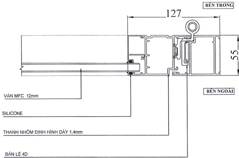
CHI TIẾT 27
