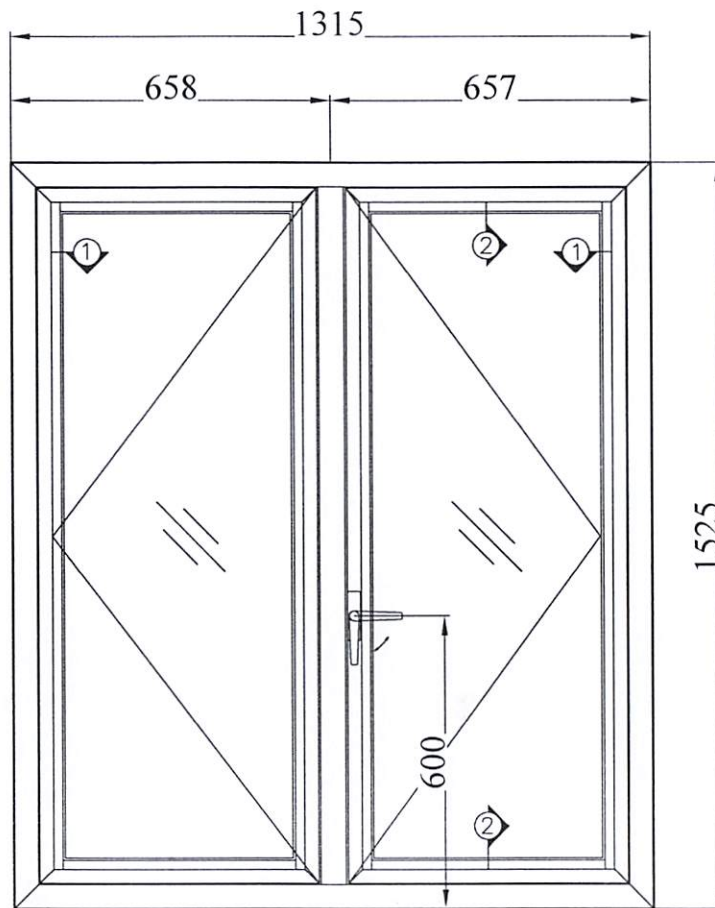
CỬA WD - 2
