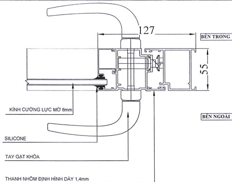
CHI TIẾT 12
