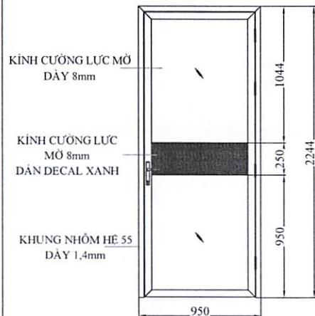
CỬA MD - 9, SL : 1 BỘ, TL: 1/40
