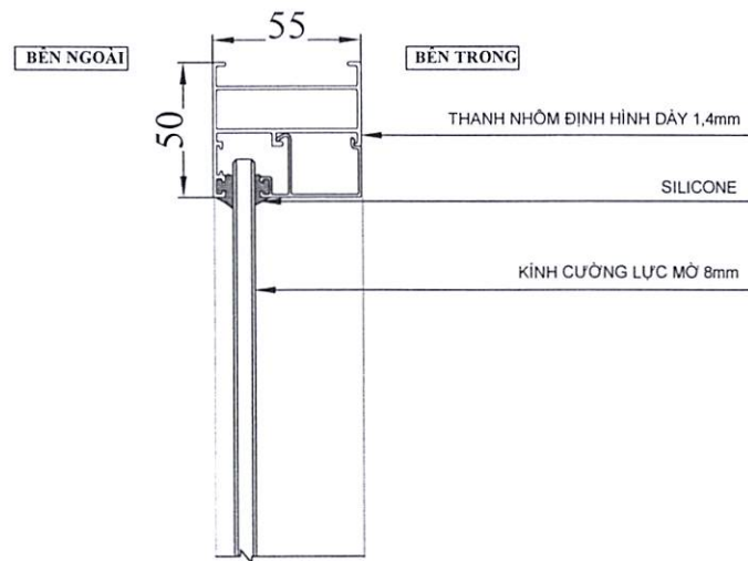
CHI TIẾT 8
