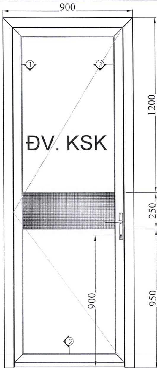
CỬA MD - 18
