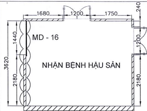
BẢN VẼ MẶT BẰNG NHẬN BỆNH HẬU SẢN TL 1/90
