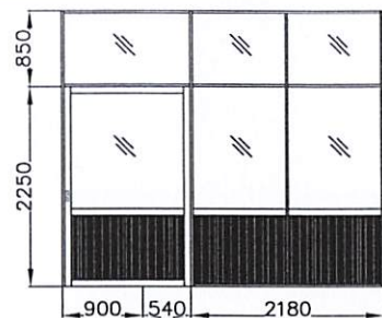
BẢN VẼ MẶT ĐỨNG VÁCH NHÔM 25x76 HIỆN TRANG TL 1/90
