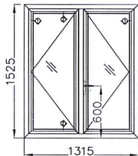
CỬA WD - 2, SL: 02 BỘ TL 1/30
