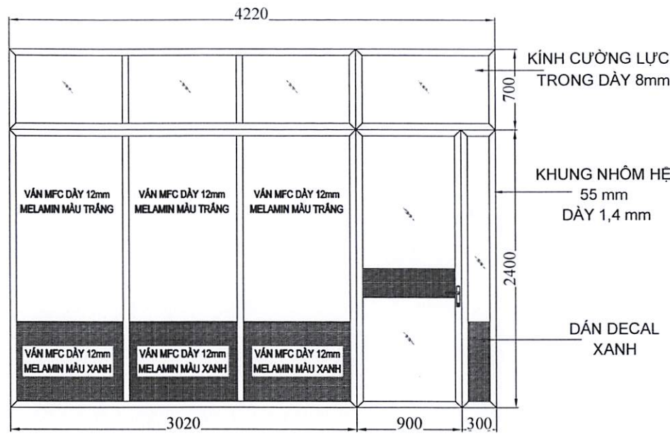
CỬA MD - 6
