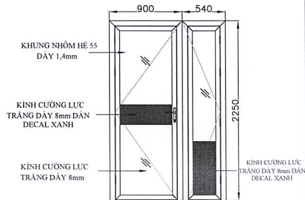
BẢN VẼ CỬA: MD - 16, TL 1/45, SL: 01 BỘ
