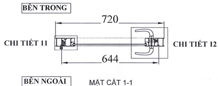
CỬA TD - 20
