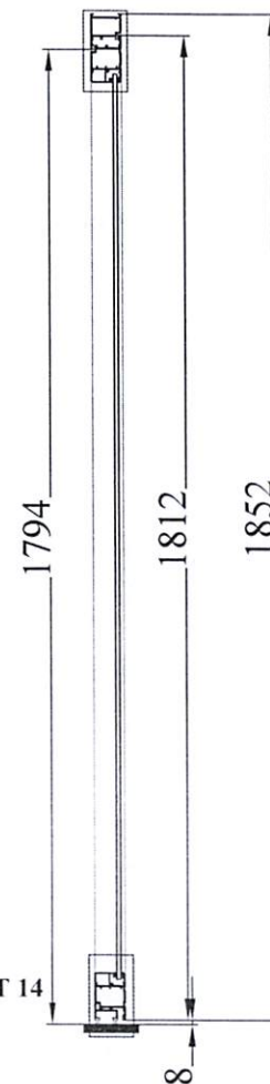
MẶT CẮT 2-2
