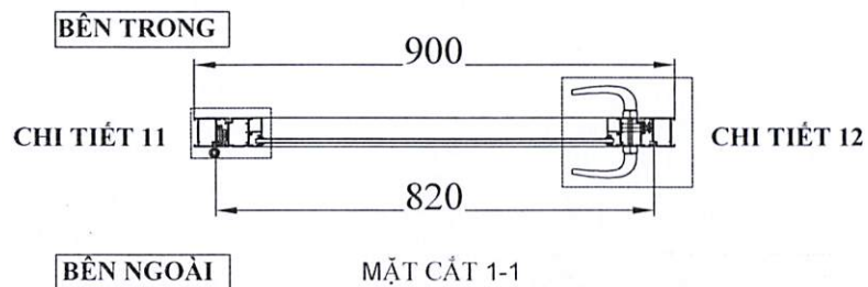
CỬA MD - 7
