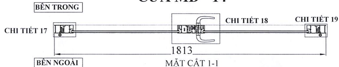
CỬA MD - 14
