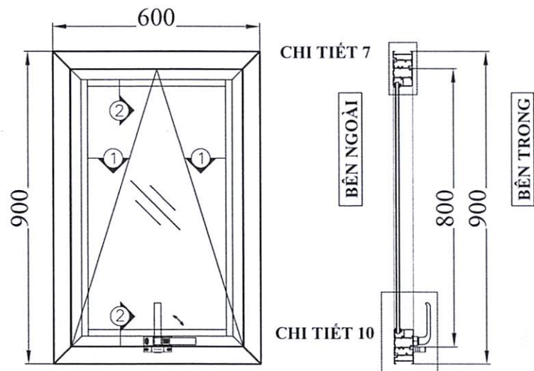
CỬA WD - 4
