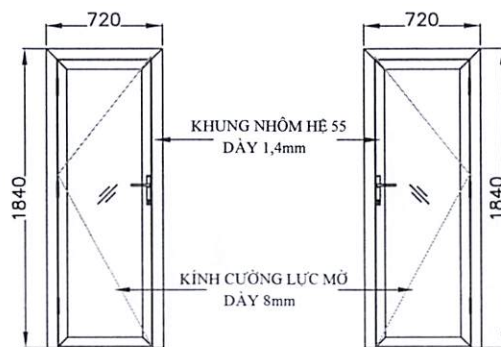
BẢN VẼ CỬA: TD - 20, TL: 1/45, SL: 03 BỘ
