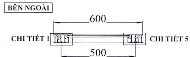
MẶT CẮT 1 - 1
