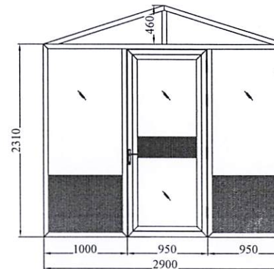
KHUNG NHÔM KÍNH CƯỜNG LỰC 8mm QUẦY BHYT THAY MỚI
