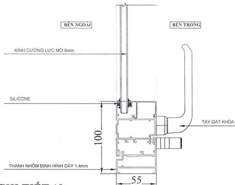
CHI TIẾT 10
