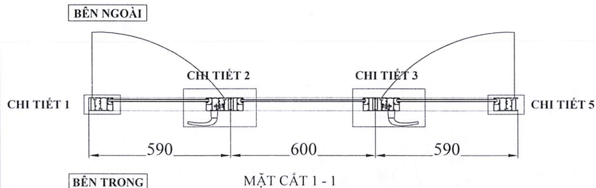
CỬA WD - 1
