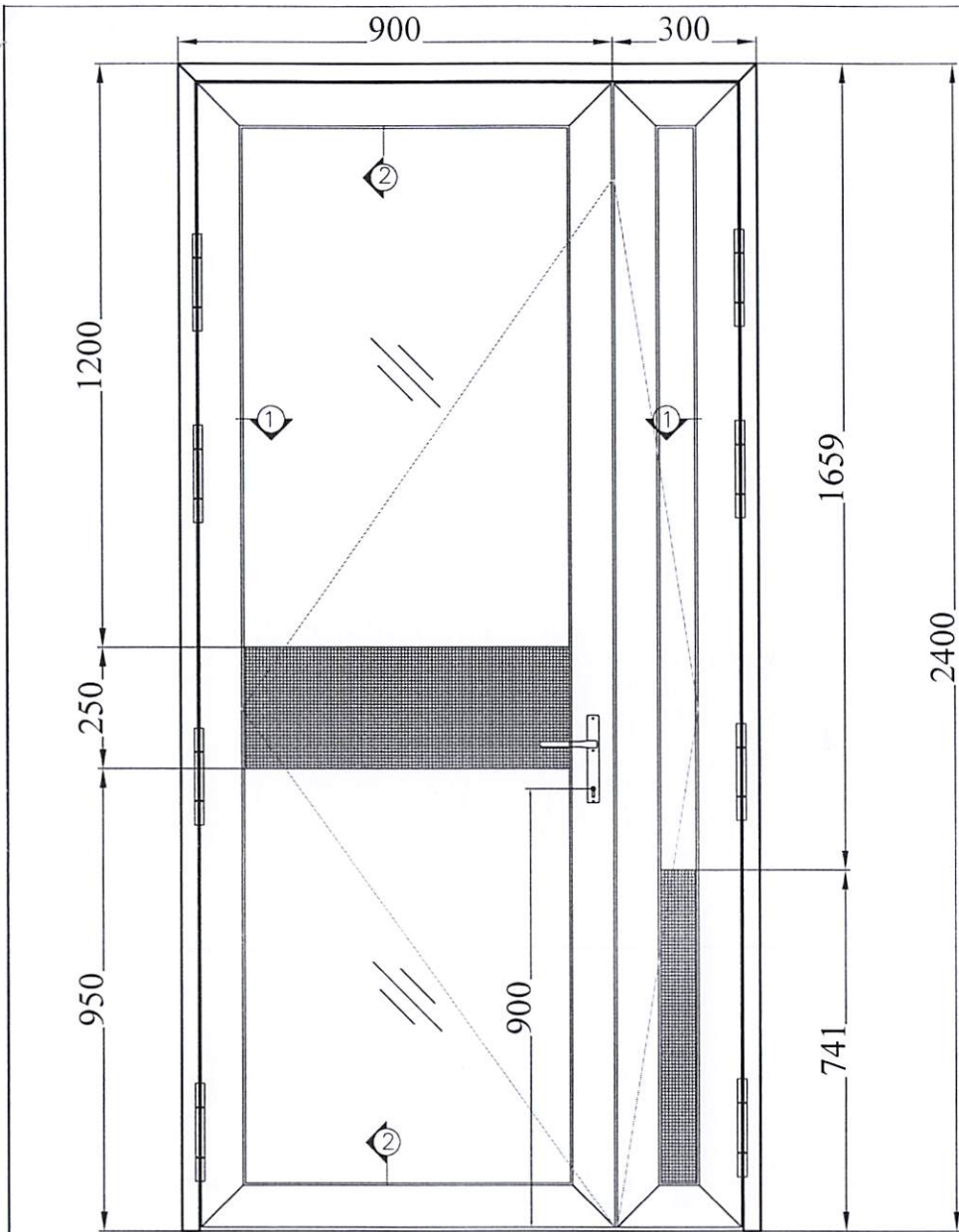
CỬA MD - 6
