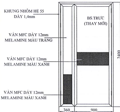
CỬA: MD - 15 TL 1/40 , SL : 01 BỘ
