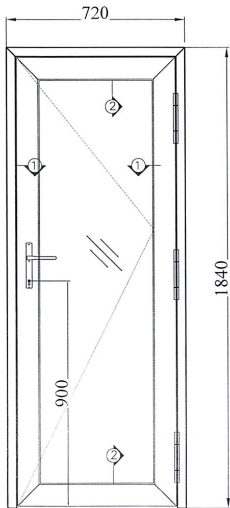
CỬA TD - 22
