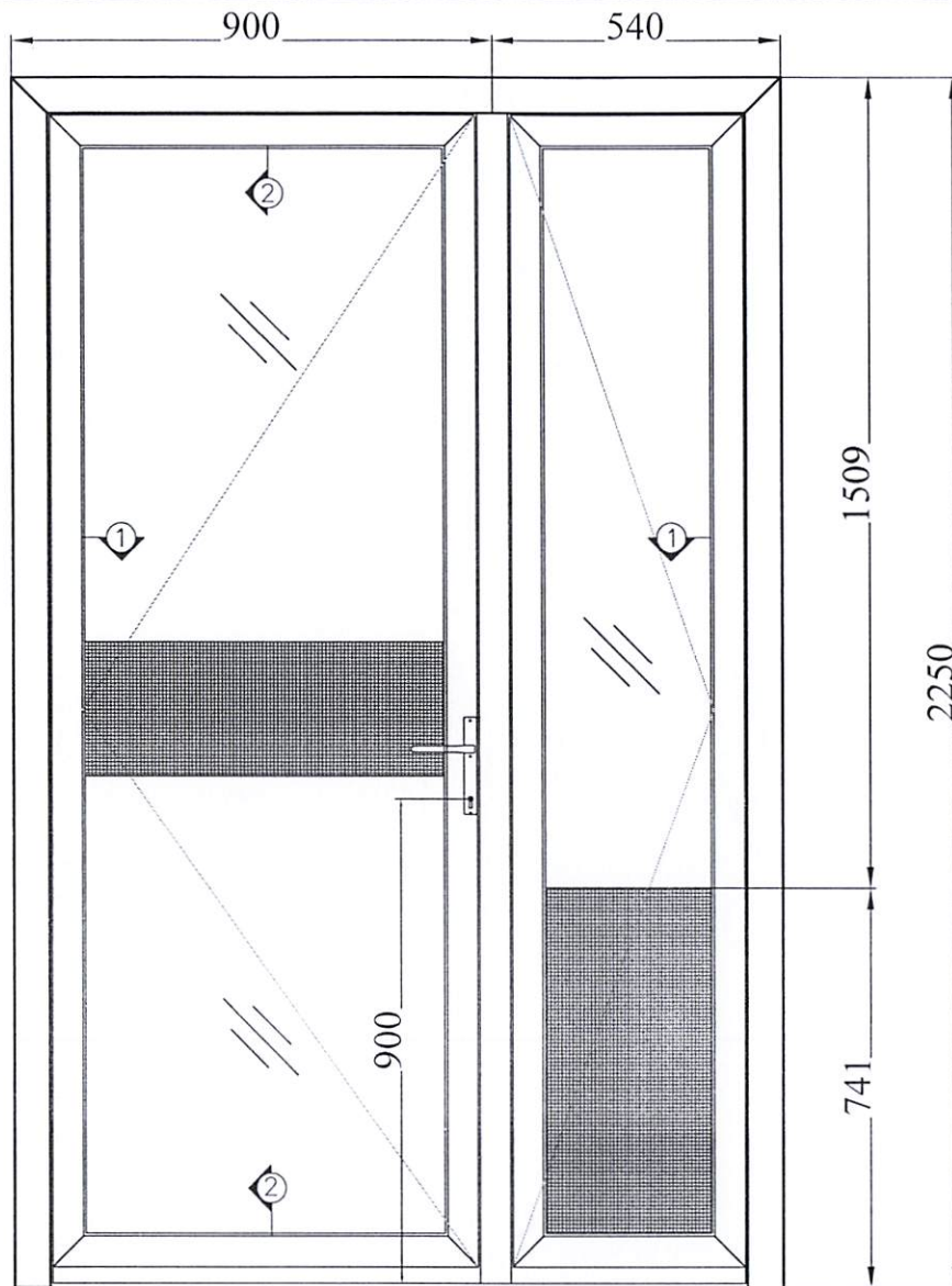
CỬA MD - 16
