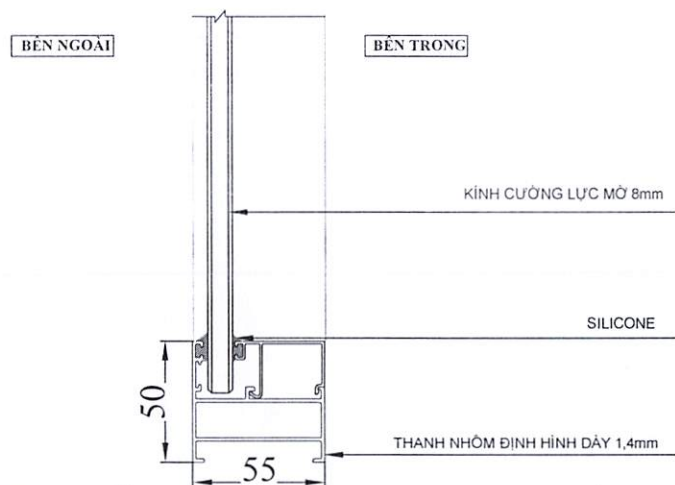
CHI TIẾT 9
