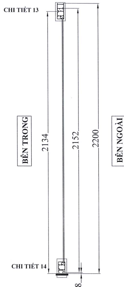
MẶT CẮT 2-2
