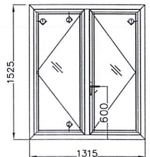
CỬA WD - 2, SL: 10 BỘ TL 1/40
