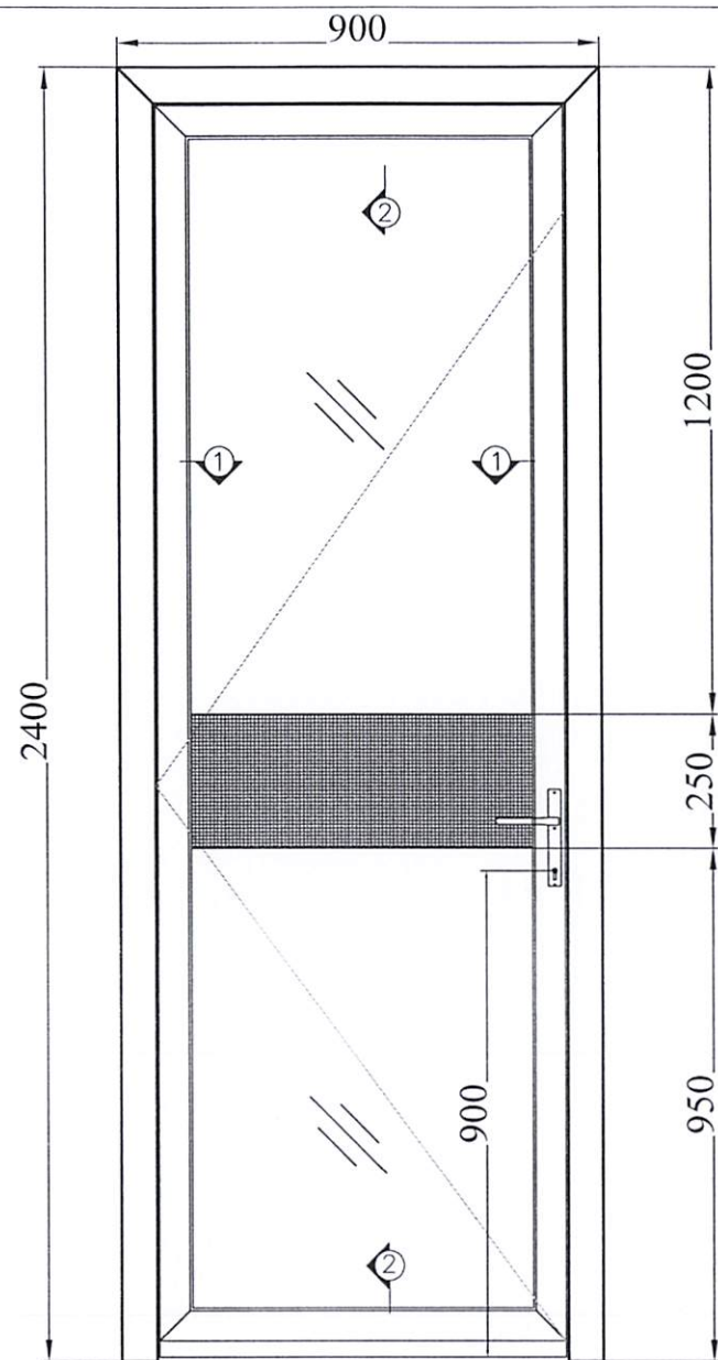
CỬA MD - 11
