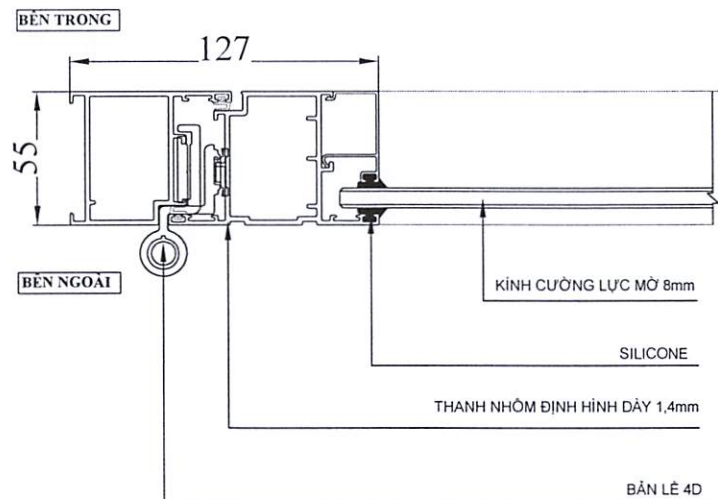
CHI TIẾT 11
