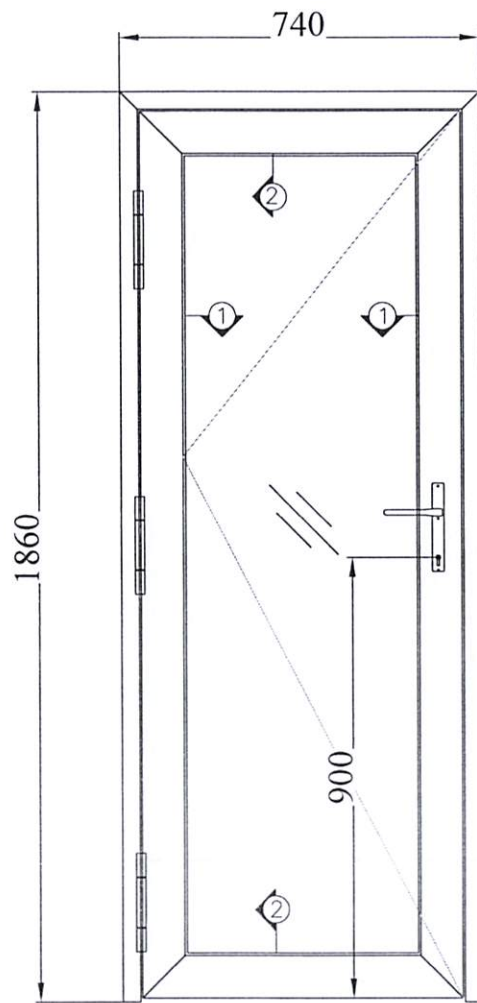
CỬA TD - 19
