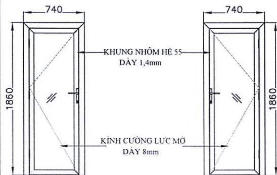
BẢN VẼ CỬA: TD - 19, TL: 1/45, SL: 02 BỘ
