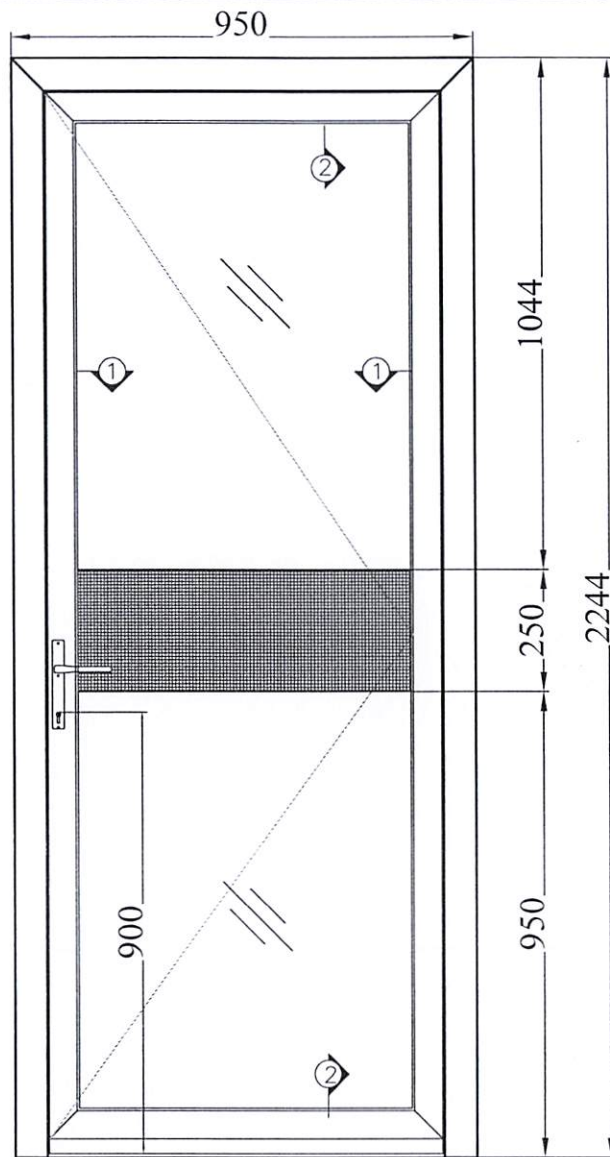
CỬA MD - 9
