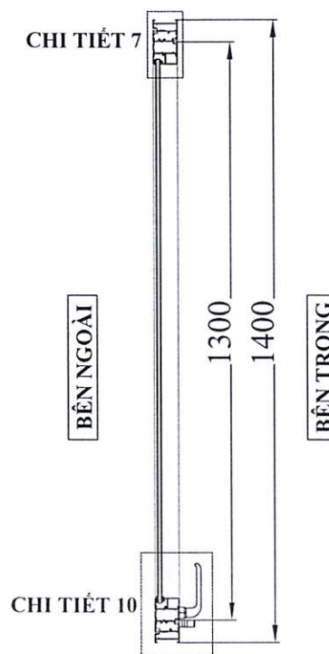
MẶT CẮT 2-2
