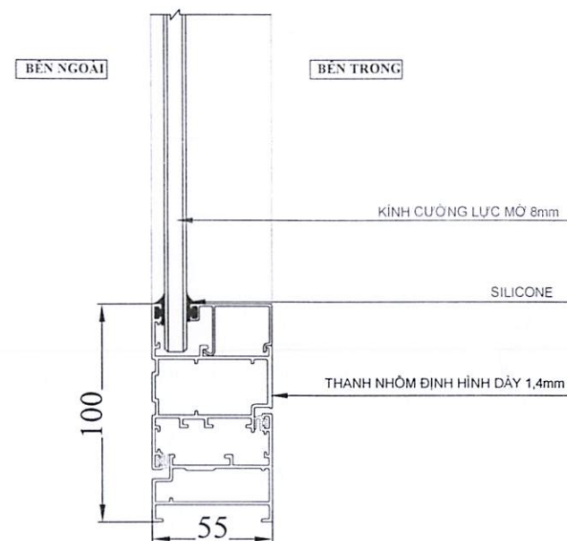
CHI TIẾT 6
