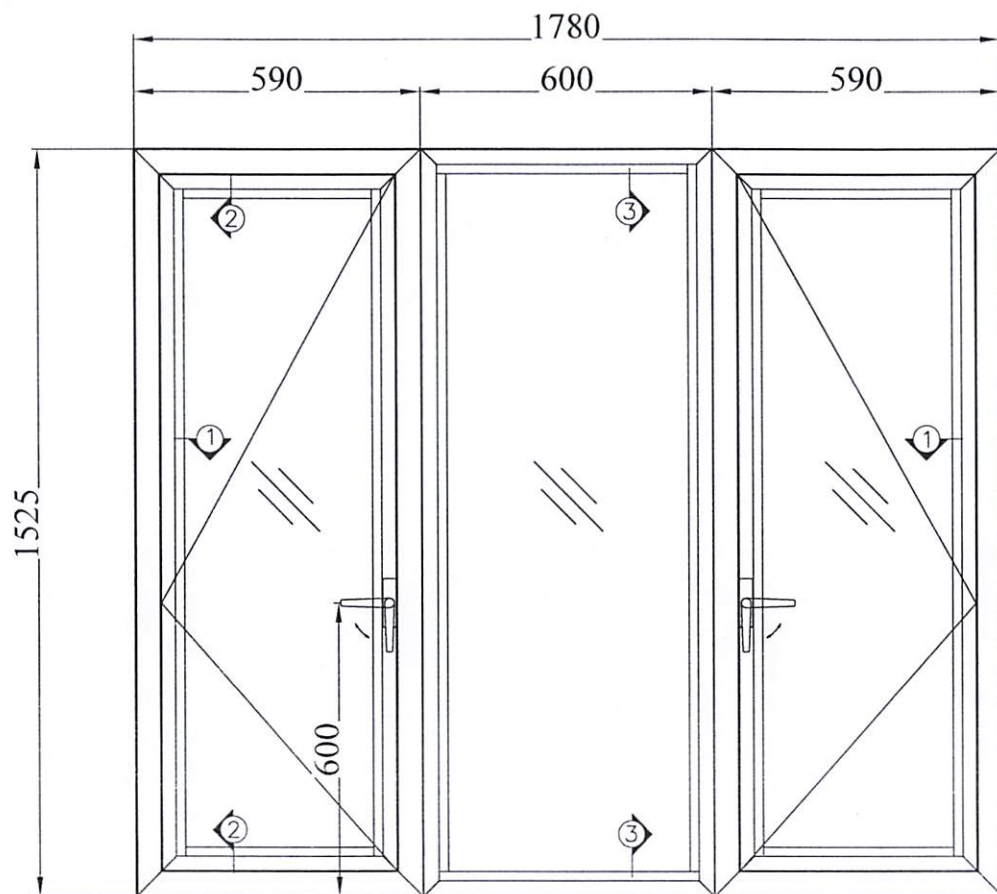
CỬA WD - 1
