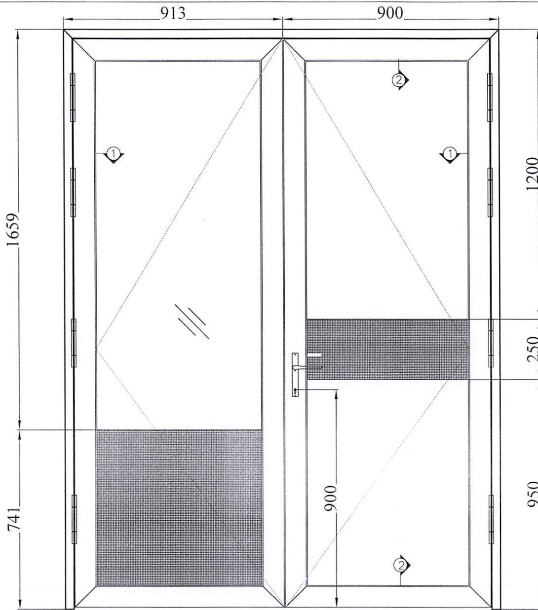
CỬA MD - 14
