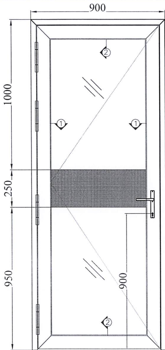
CỬA MD - 7
