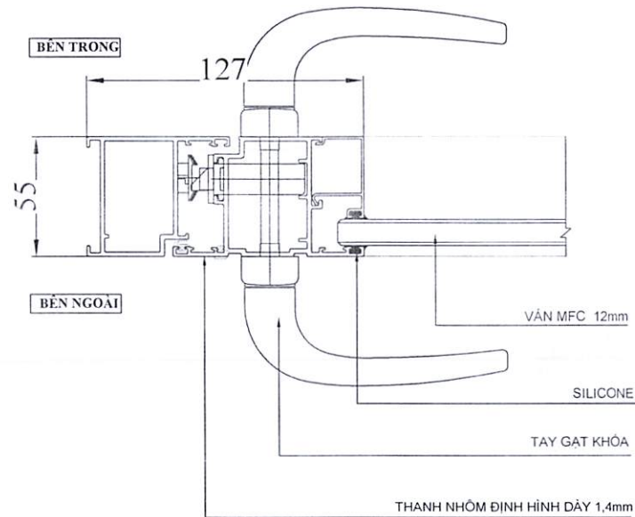
CHI TIẾT 26
