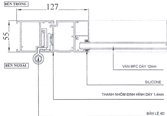
CHI TIẾT 17
