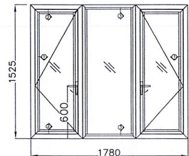
CỬA WD - 1, SL: 08 BỘ TL 1/40
