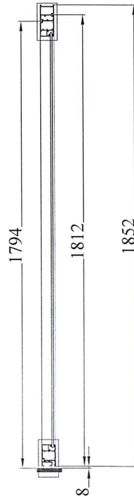
MẶT CẮT 2-2
