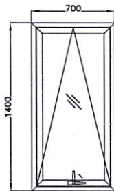
CỬA: WD - 3, SL: 03 BỘ TL 1/80
