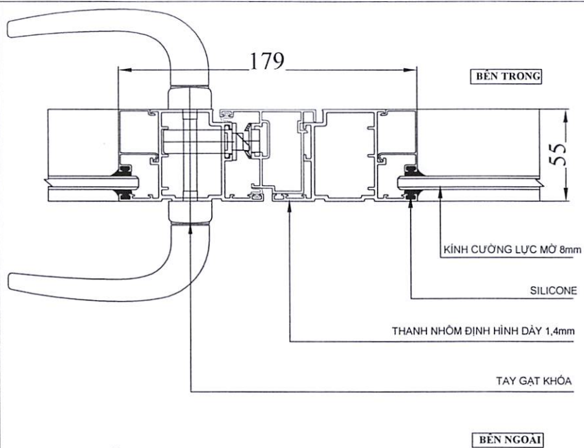
CHI TIẾT 15
