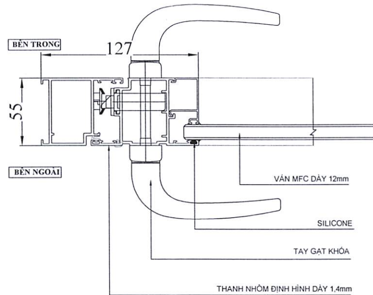
CHI TIẾT 20
