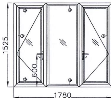
CỬA WD - 1, SL: 08 BỘ TL 1/30
