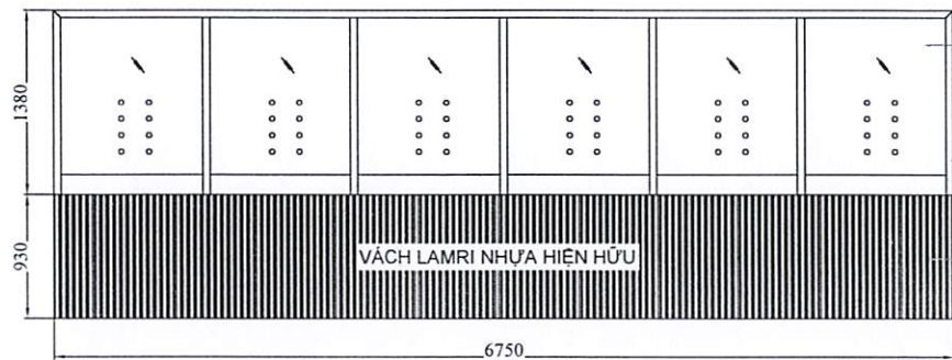
KHUNG NHÔM KÍNH CL TRONG 8MM QUẦY BHYT THAY MỚI
