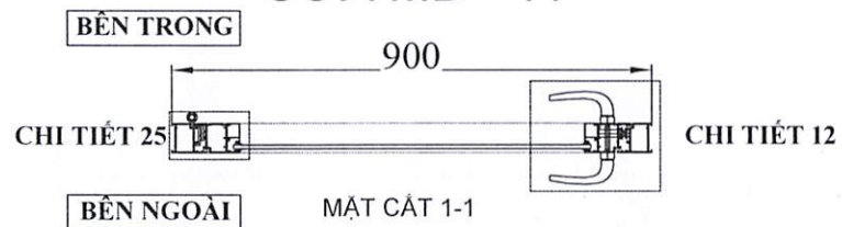
CỬA MD - 11
