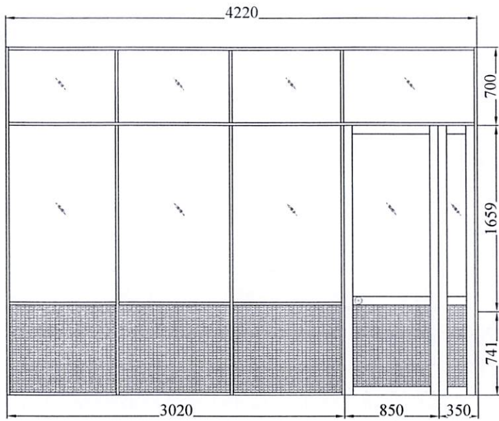
MẶT ĐỨNG VÁCH, CỬA HIỆN TRẠNG KHOA XÉT NGHIỆM
