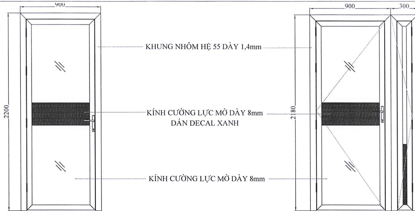
CỬA MD - 7, SL: 01 BỘ TL 1/25
