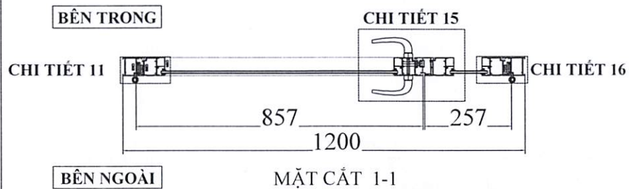
CỬA MD - 8
