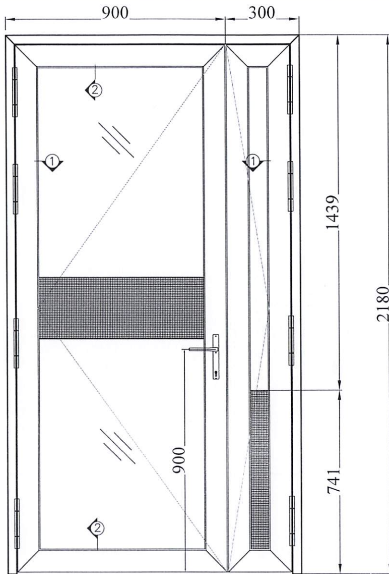
CỬA MD - 8
