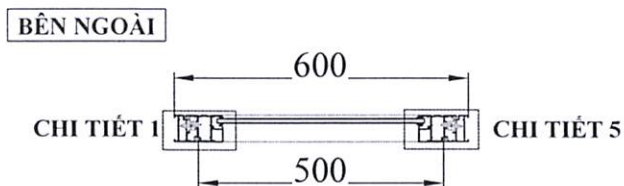
BÊN TRONG MẶT CẮT 1-1
