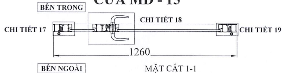
CỬA MD - 15
