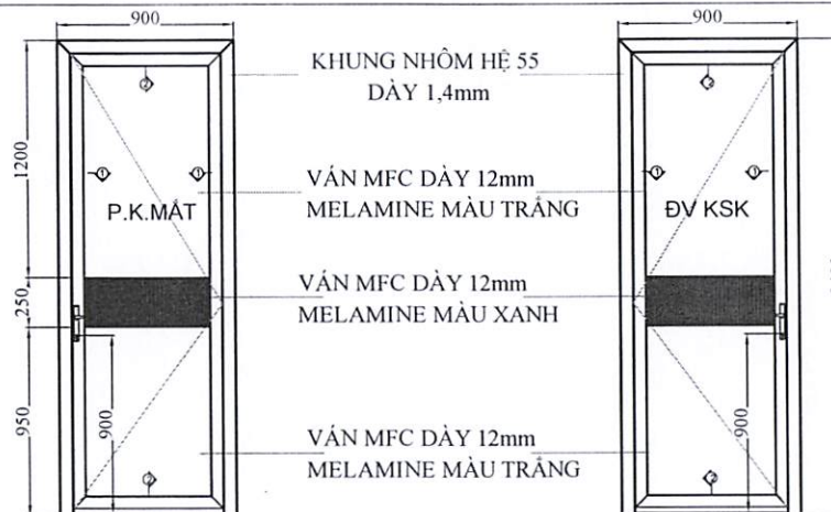
CỬA MD - 17
