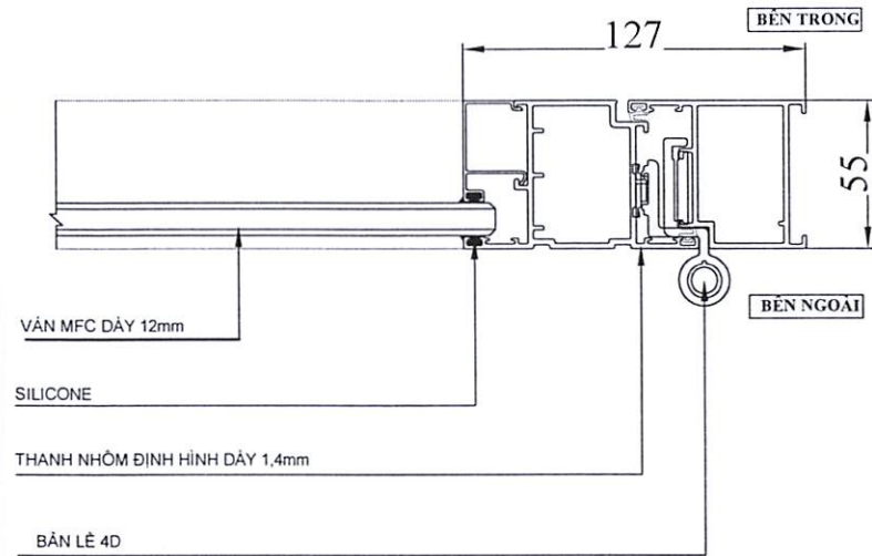
CHI TIẾT 19
