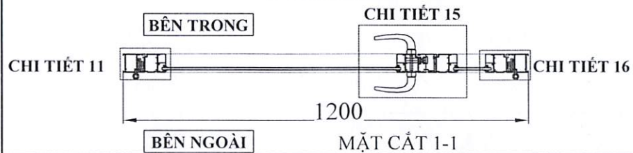
CỬA MD - 6
