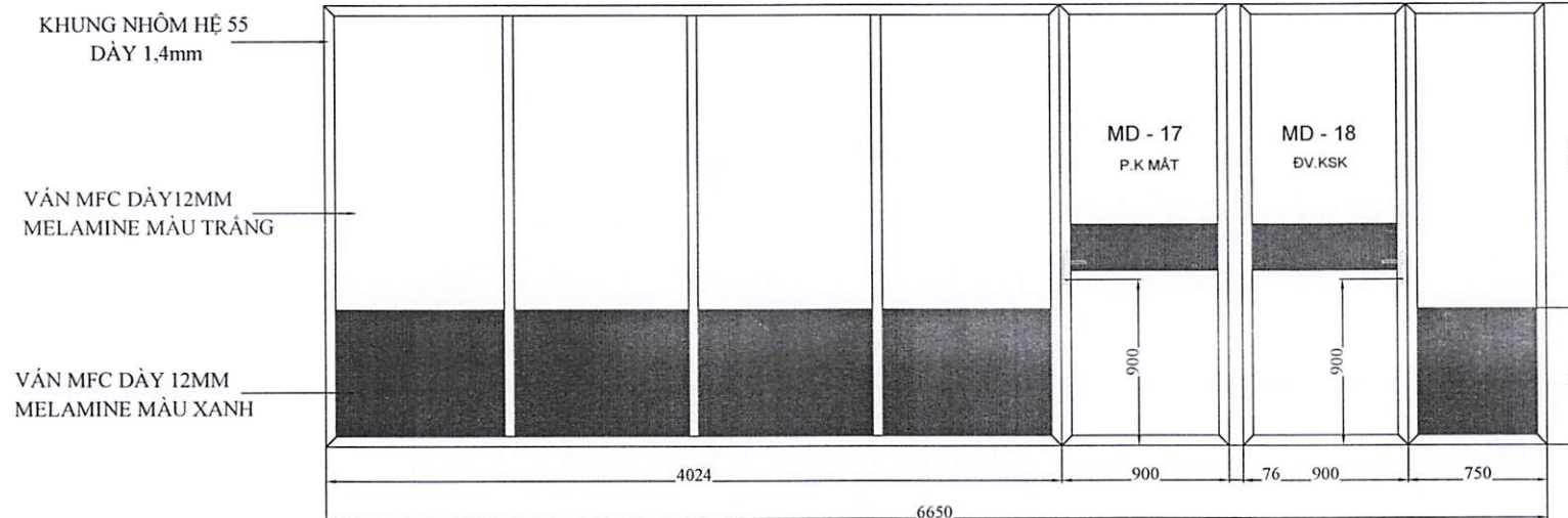
MẶT ĐỪNG VÁCH NHÔM ĐƠN VỊ KHÁM SỨC KHỎE, PHÒNG KHÁM MẮT
