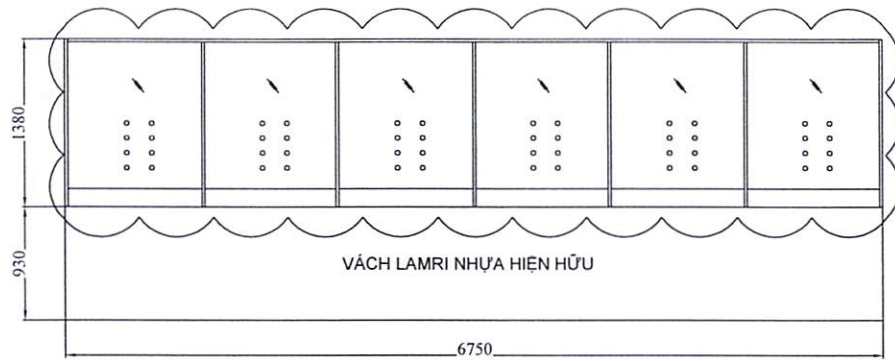
VÁCH NHÔM KÍNH HỆ 25x76 QUẦY BHYT XUỐNG CẤP TL 1/60
