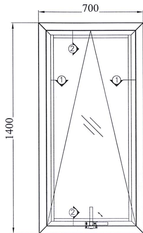
CỬA WD - 3
