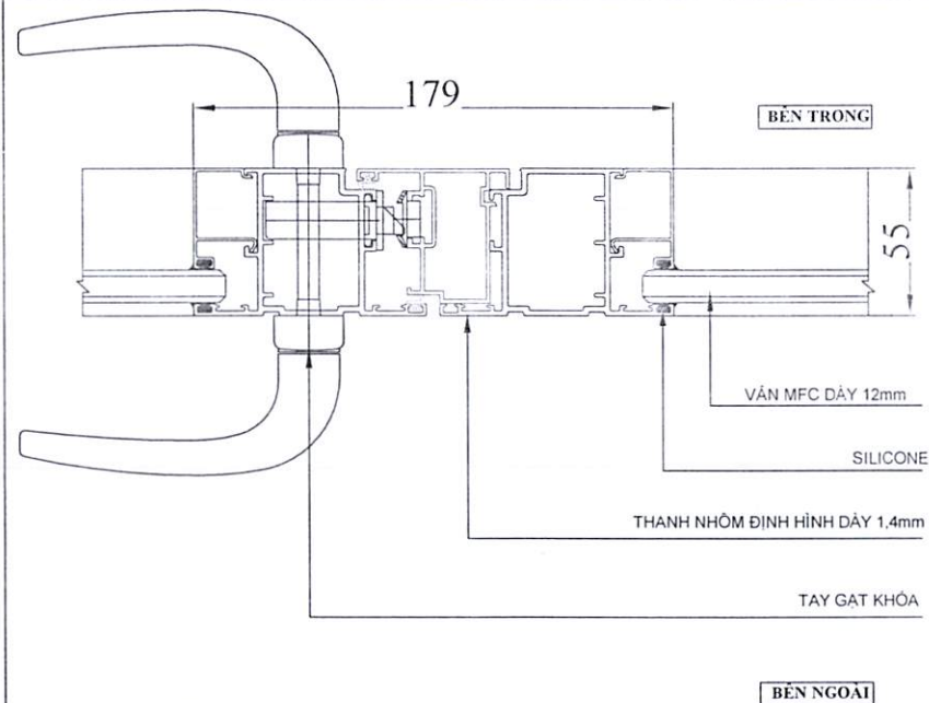
CHI TIẾT 18
