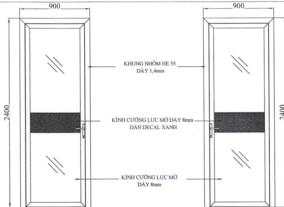
CỬA MD - 11, TL 1/15 , SL: 01 BỘ
