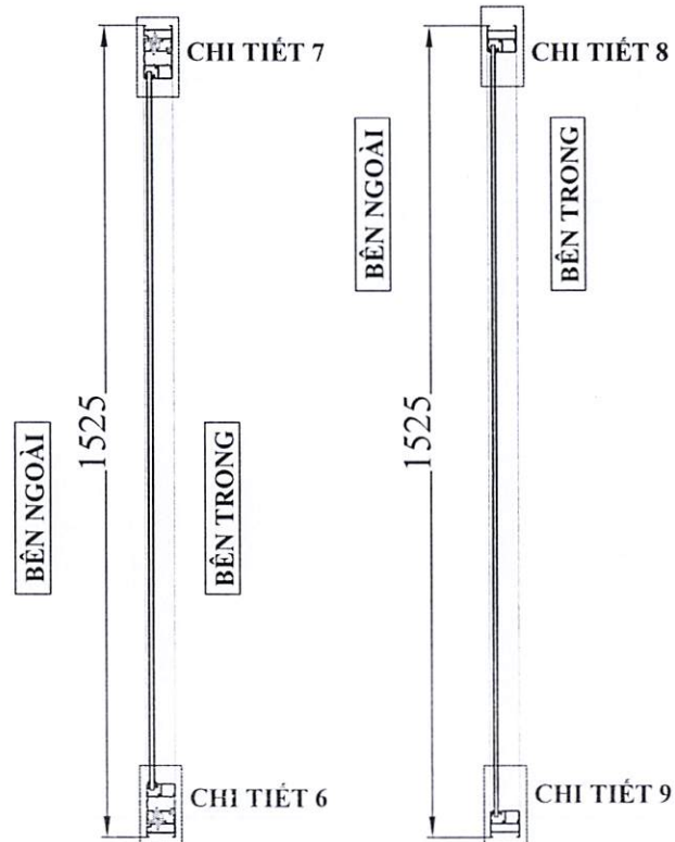
MẶT CẮT 2 - 2
