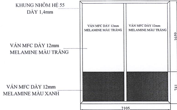
VÁCH NGĂN P. MẮT, ĐV KSK
