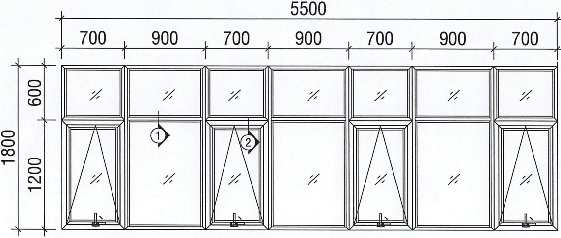
MẶT ĐỨNG CỬA SỔ VK3 TRONG NHÌN CỬA BẬT RA NGOÀI
