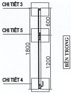
Mặt cắt 2-2
