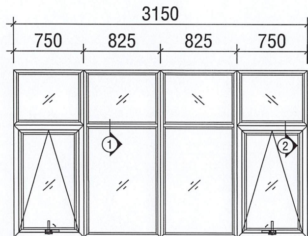
MẶT ĐÚNG CỬA SỔ VK1 TRONG NHÌN CỬA BẬT RA NGOÀI
