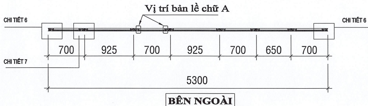
MẶT BẰNG CỬA SỔ VK2
