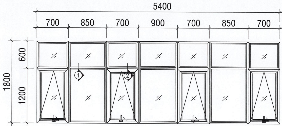
MẶT ĐỨNG CỬA SỔ VK4 TRONG NHÌN CỬA BẬT RA NGOÀI
