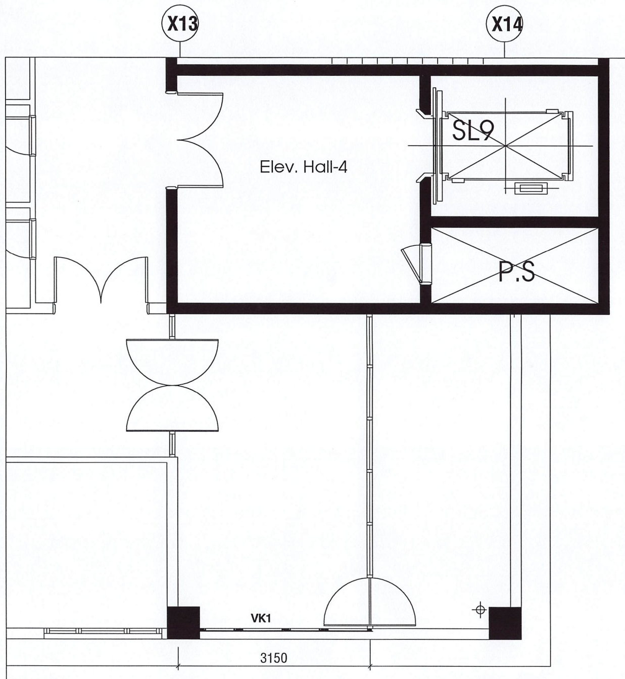
MẶT BẰNG CỬA SỔ NHÔM KÍNH LẦU 7 BLOCK B
