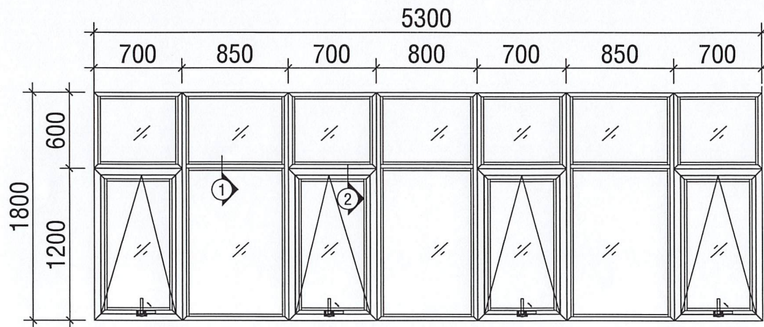
MẶT ĐÚNG CỬA SỔ VK2 TRONG NHÌN CỬA BẬT RA NGOÀI
