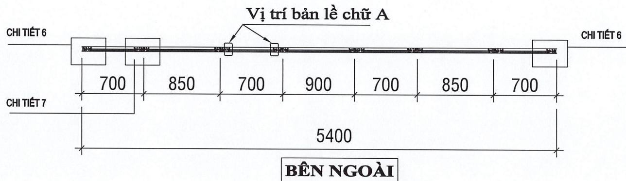
MẶT BẰNG CỬA SỔ VK4
