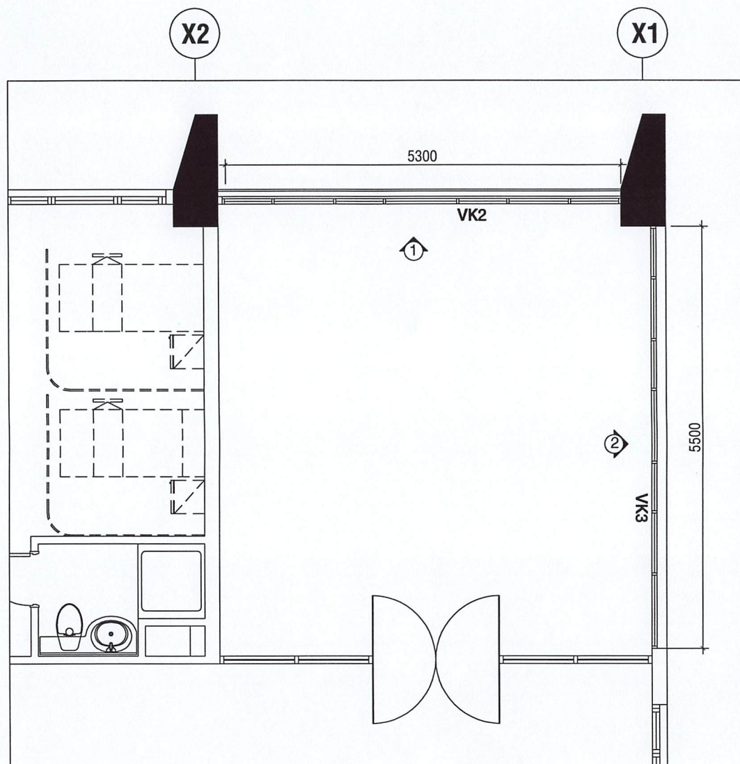
MẶT BẰNG CỬA SỔ NHÔM KÍNH LẦU 7, 10, 11, 12, 13, 14 BLOCK A
