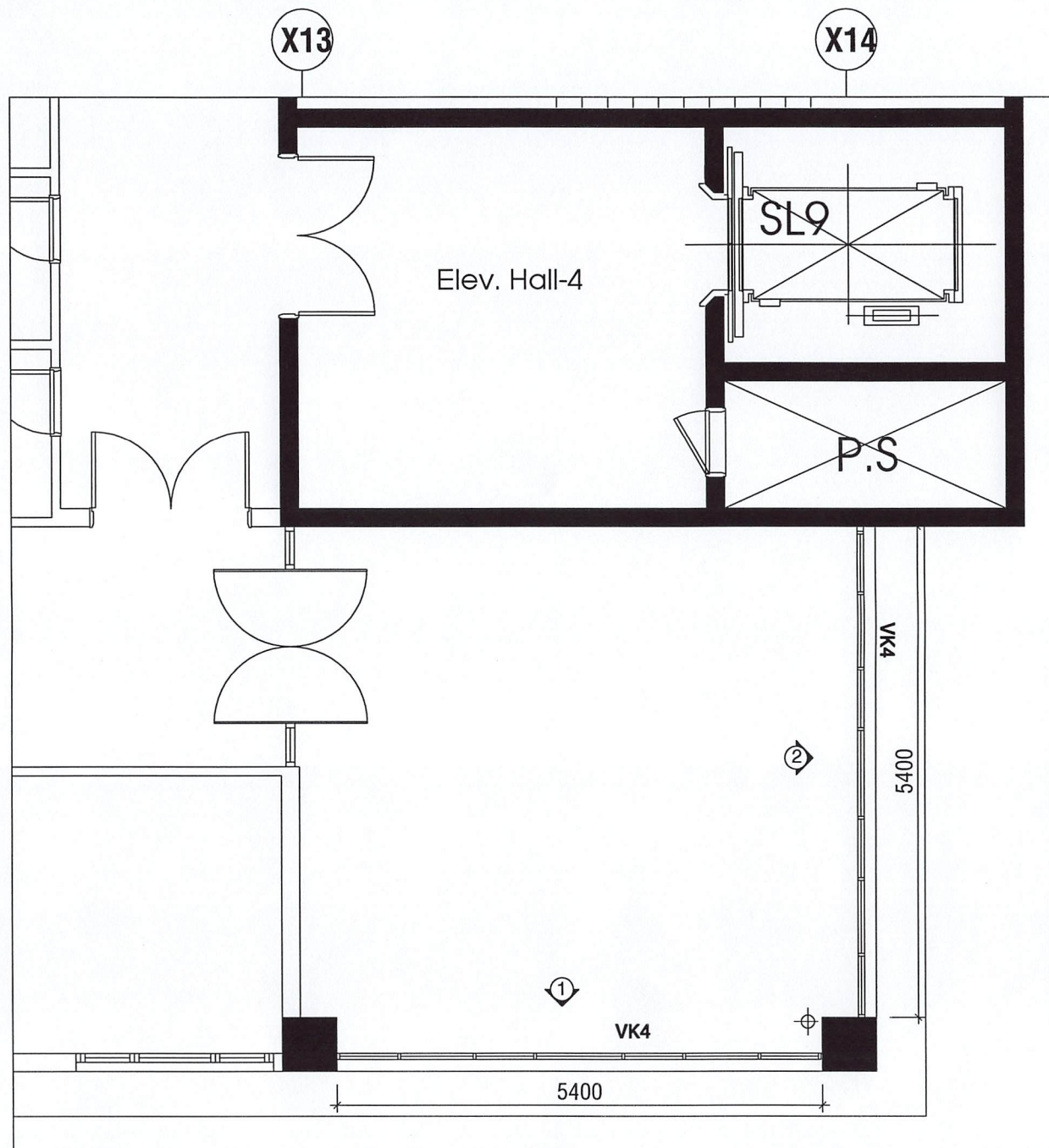
MẶT BẰNG CỬA SỔ NHÔM KÍNH LẦU 8, 11, 12, 13 BLOCK B
