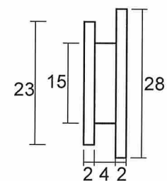
Mặt bên
