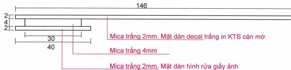
Mặt bằng
