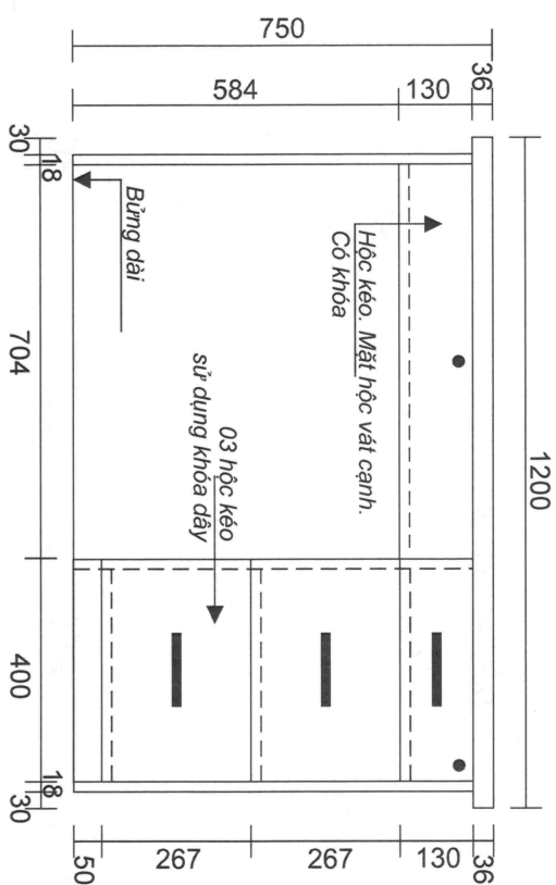
MẶT ĐÚNG
