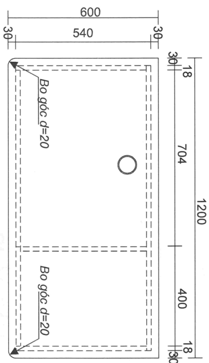
MẶT BẰNG
