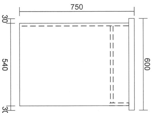
MẶT BÊN
