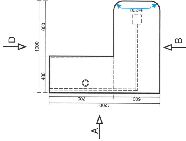
MẶT BẰNG
