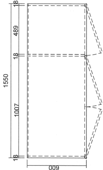
MẶT BẰNG
