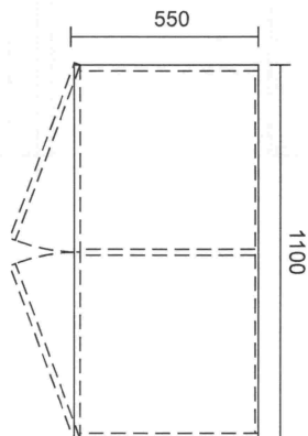
MẶT BẰNG
