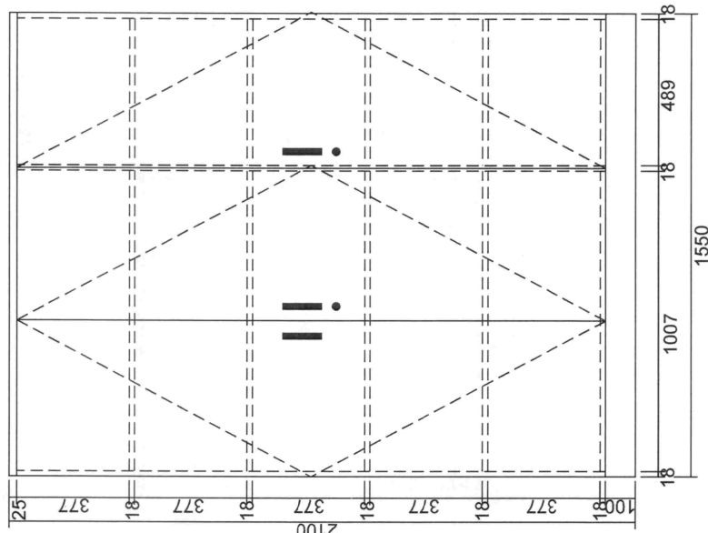
MẶT ĐÚNG
