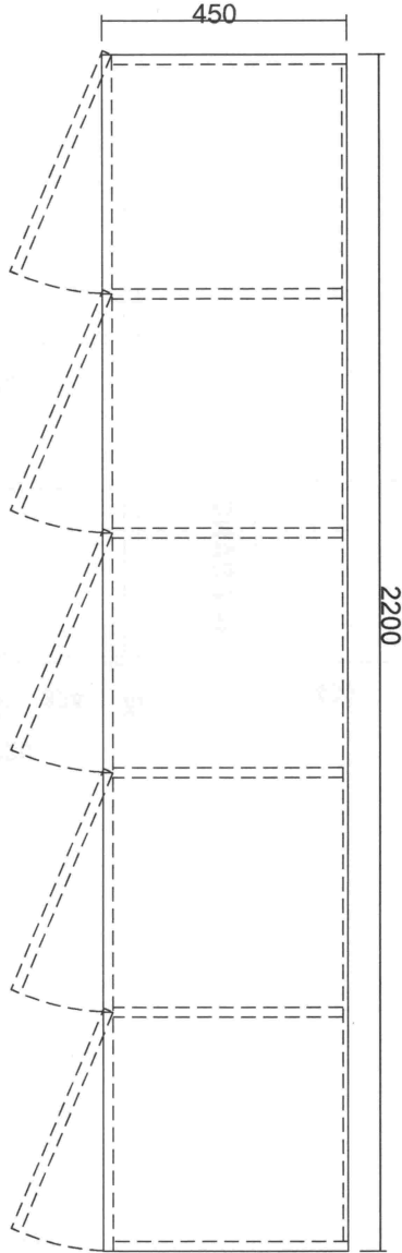
MẶT BẰNG
