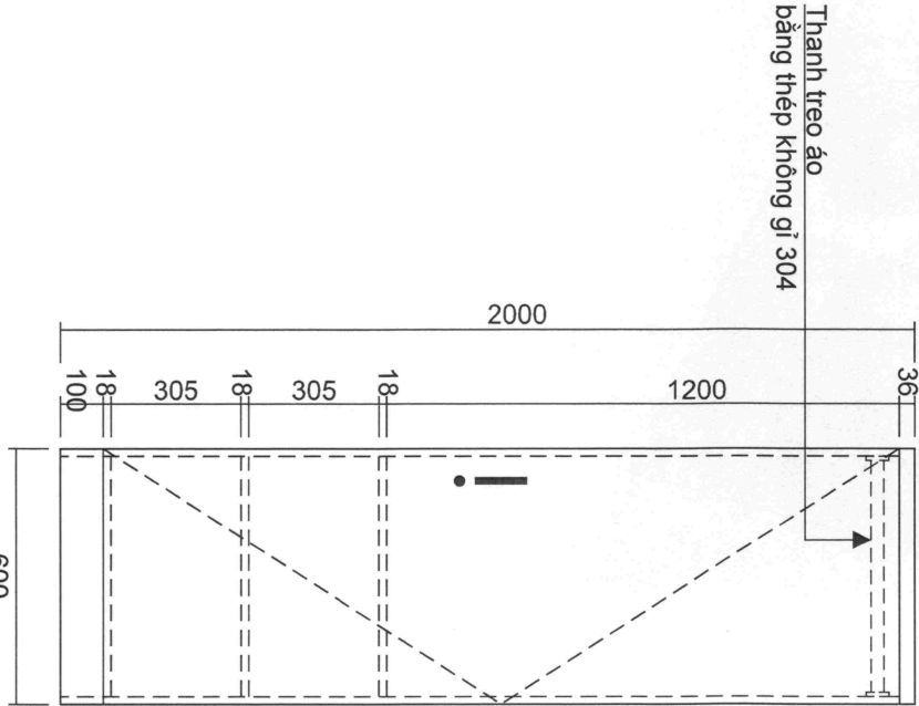
MẶT ĐÚNG
