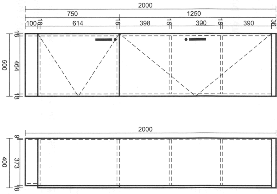
MẶT ĐỨNG
