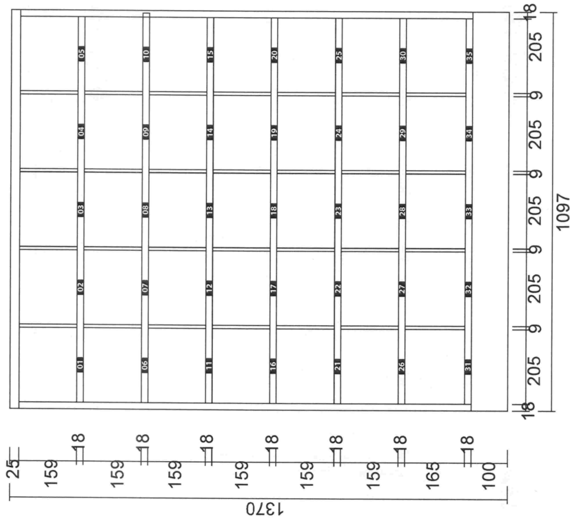
MẶT ĐỨNG
