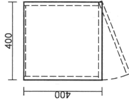
MẶT BẰNG
