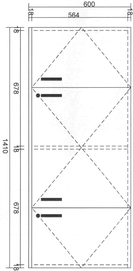
MẶT ĐÚNG
