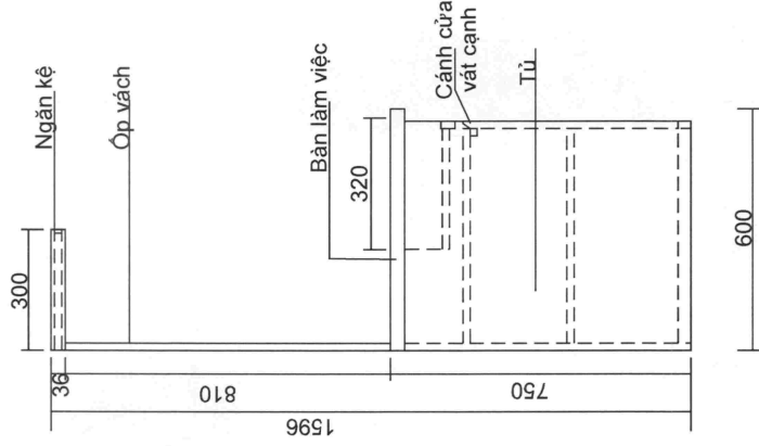
MẶT BÊN
