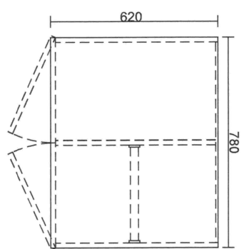
MẶT BẰNG
