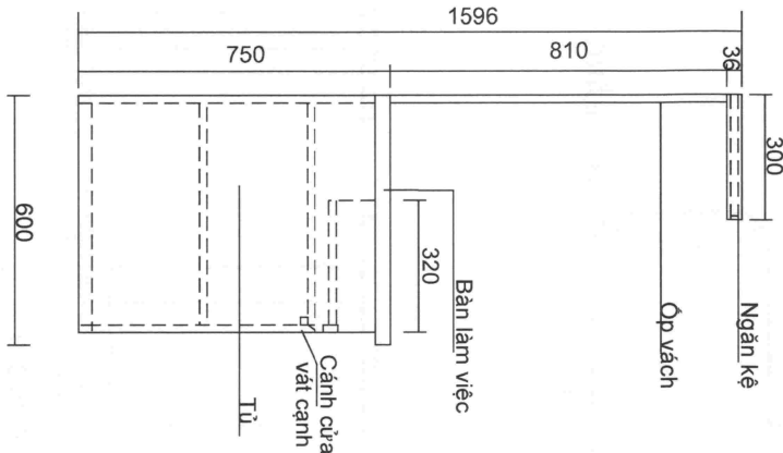
MẶT BÊN
