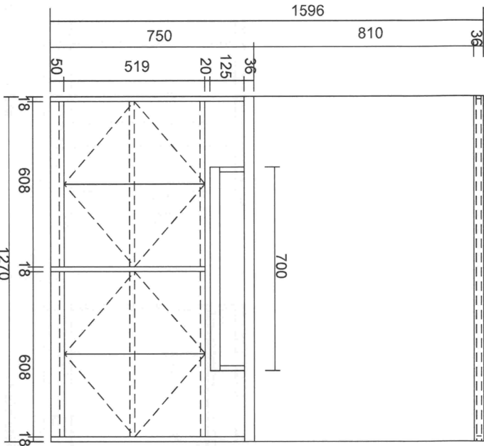
MẶT ĐỨNG
