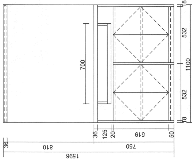
MẶT ĐỨNG
