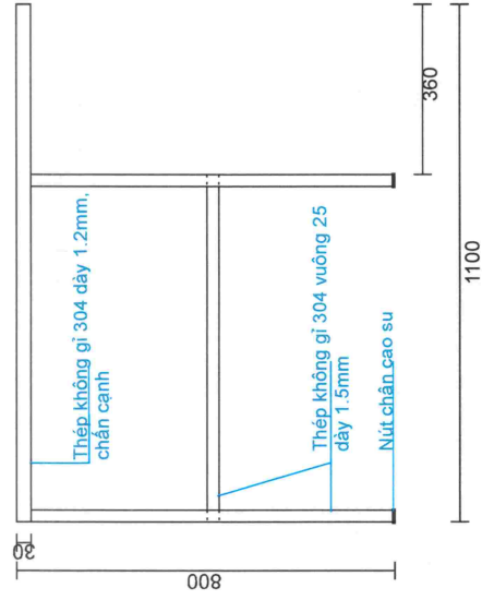
MẶT ĐÚNG
