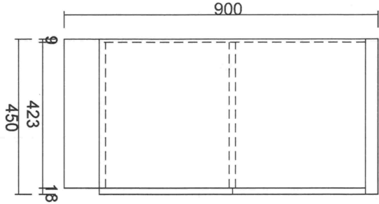
MẶT BÊN
