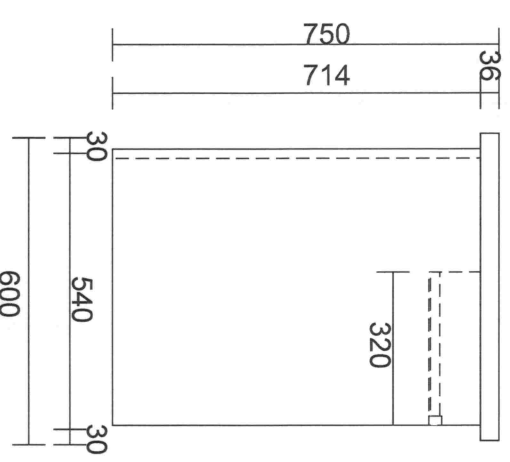
MẶT BÊN
