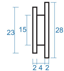
Mặt bên
