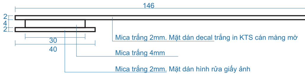
Mặt bằng
