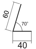
MẶT BÊN
