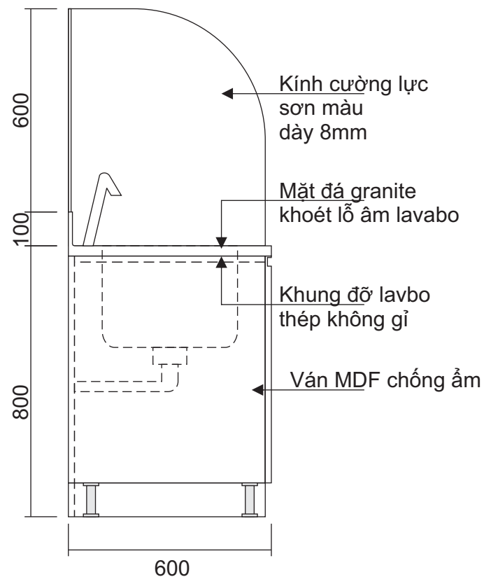
MẶT BÊN
