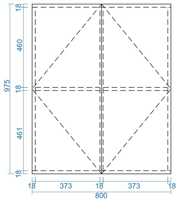
MẶT ĐỨNG
