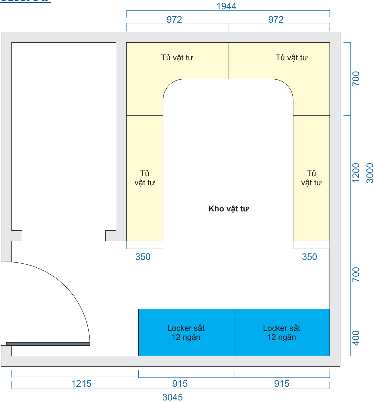
Mặt bằng bố trí nội thất Kho vật tư Khoa PTTM
