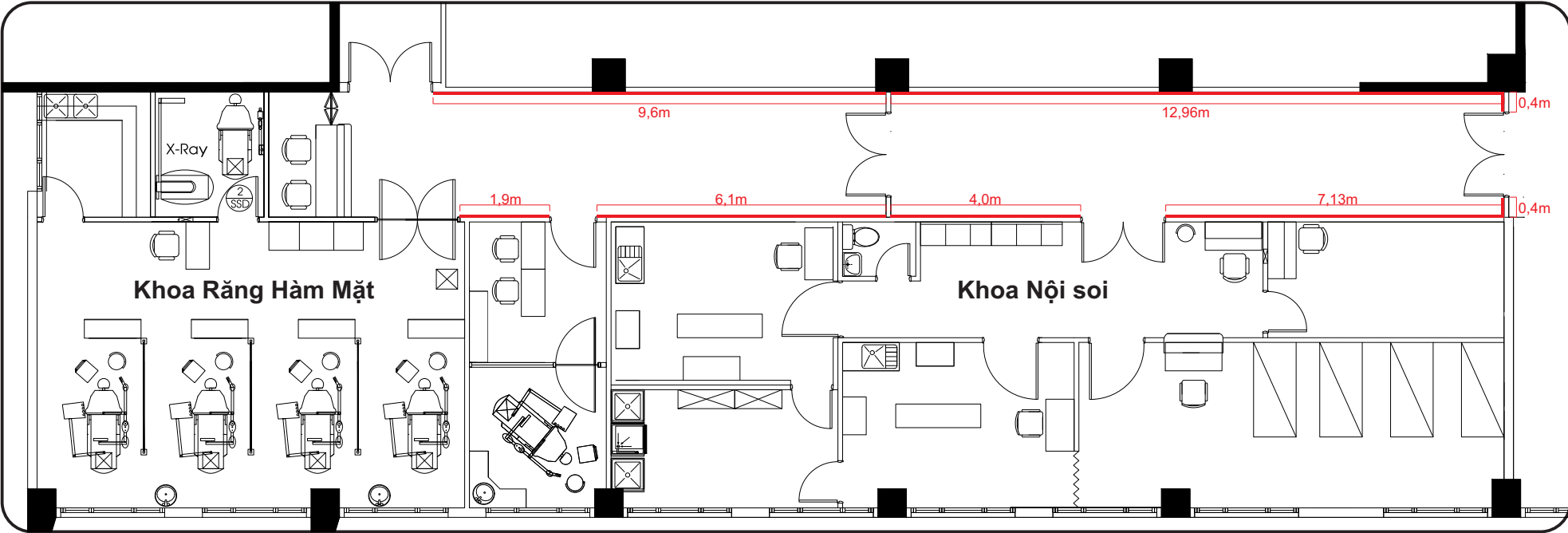
Mặt bằng bố trí ốp len tường
