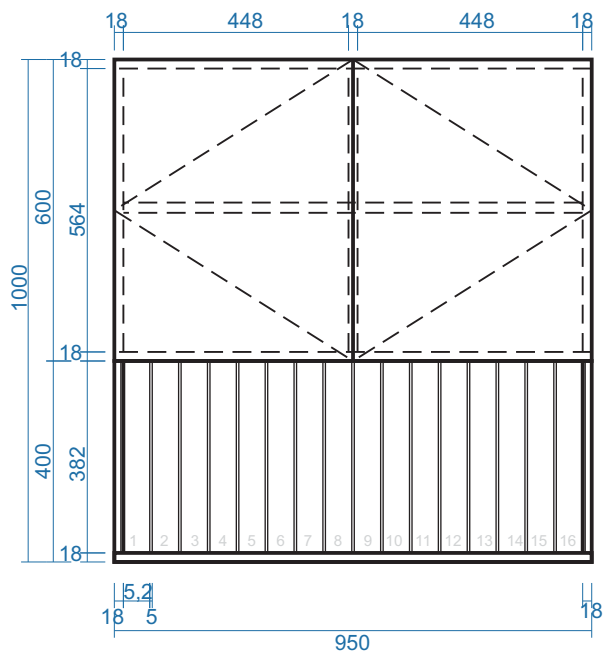
MẶT ĐỨNG
