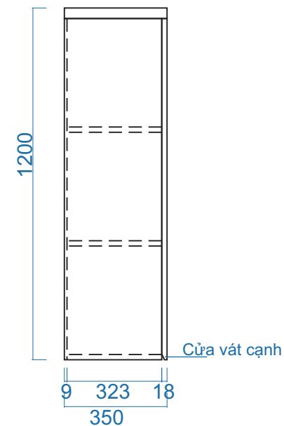
MẶT BÊN
