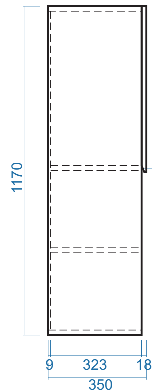
MẶT BÊN
