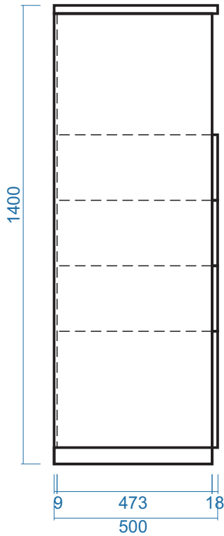
MẶT BÊN
