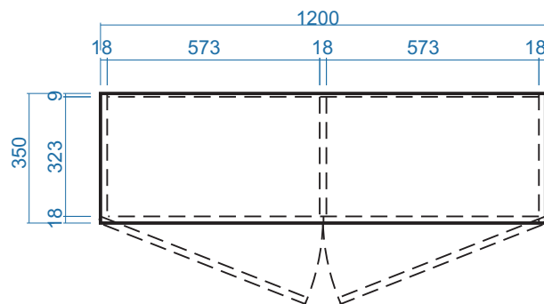
MẶT BÀNG
