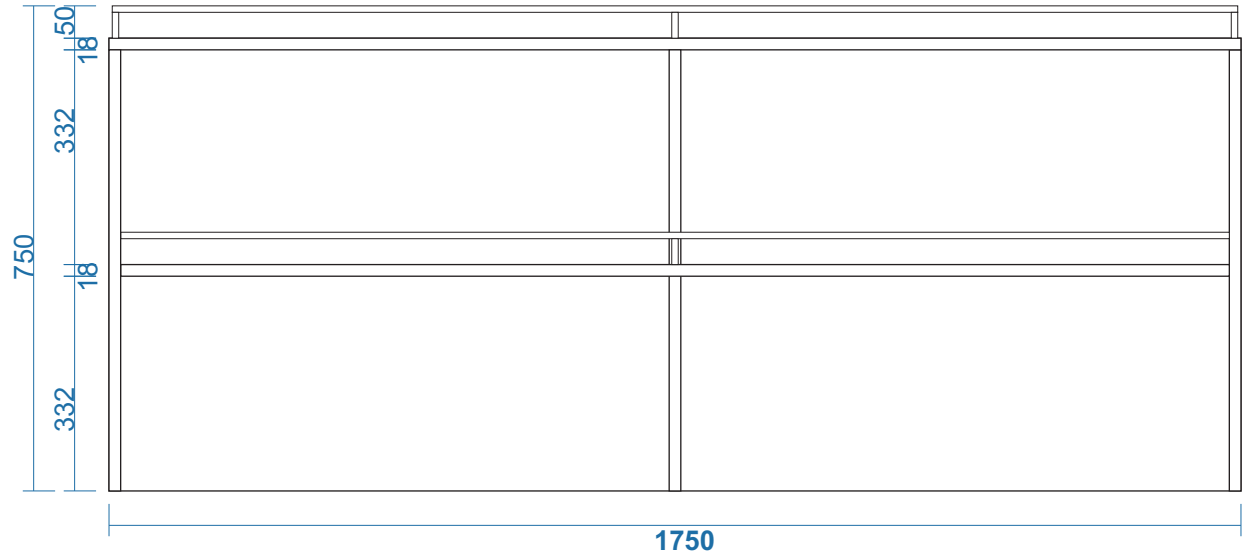
MẶT ĐỨNG
