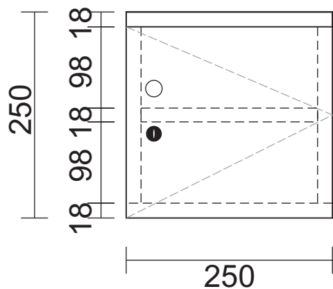
MẶT CHÍNH
