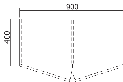
MẶT BẰNG
