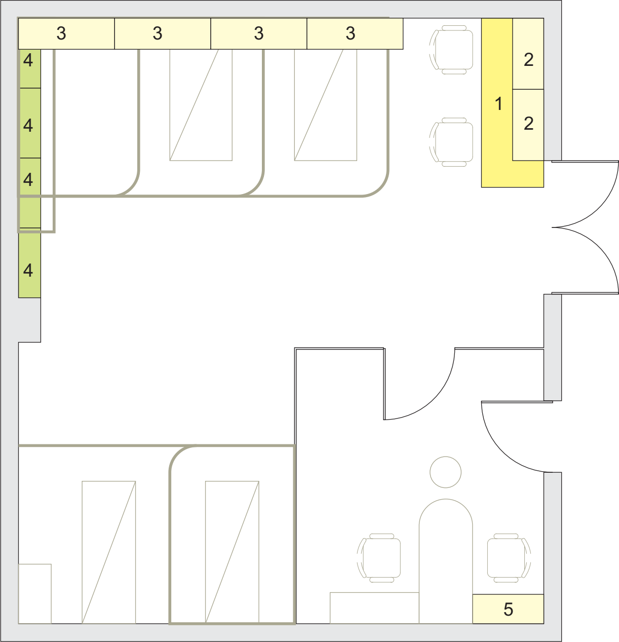
Mặt bằng bố trí nội thất Phòng tập Vật lý trị liệu
