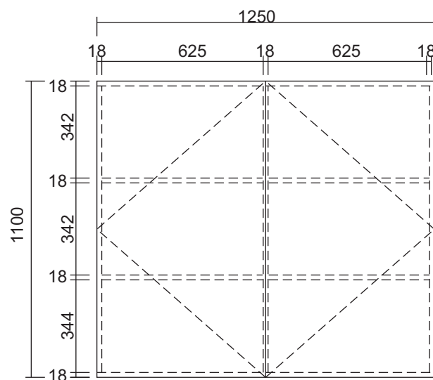
MẶT ĐỨNG
