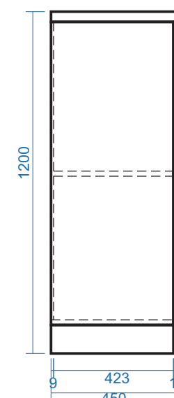
MẶT BÊN
