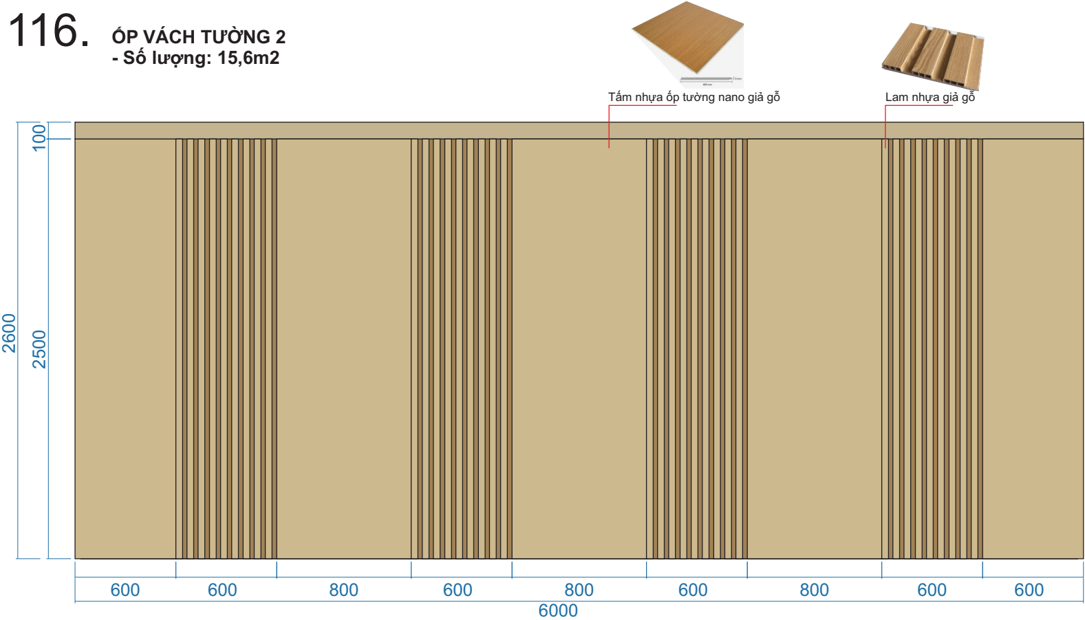
MẶT ĐỨNG
