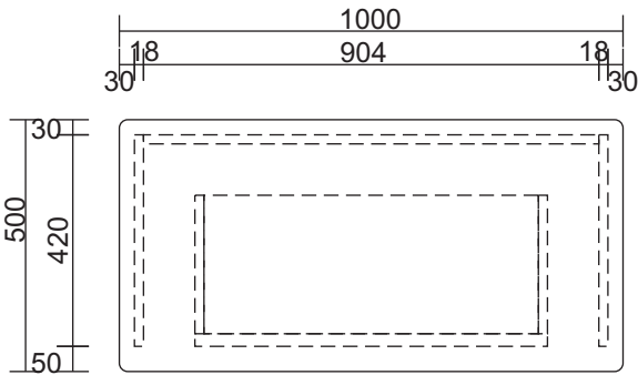
MẶT BẰNG
