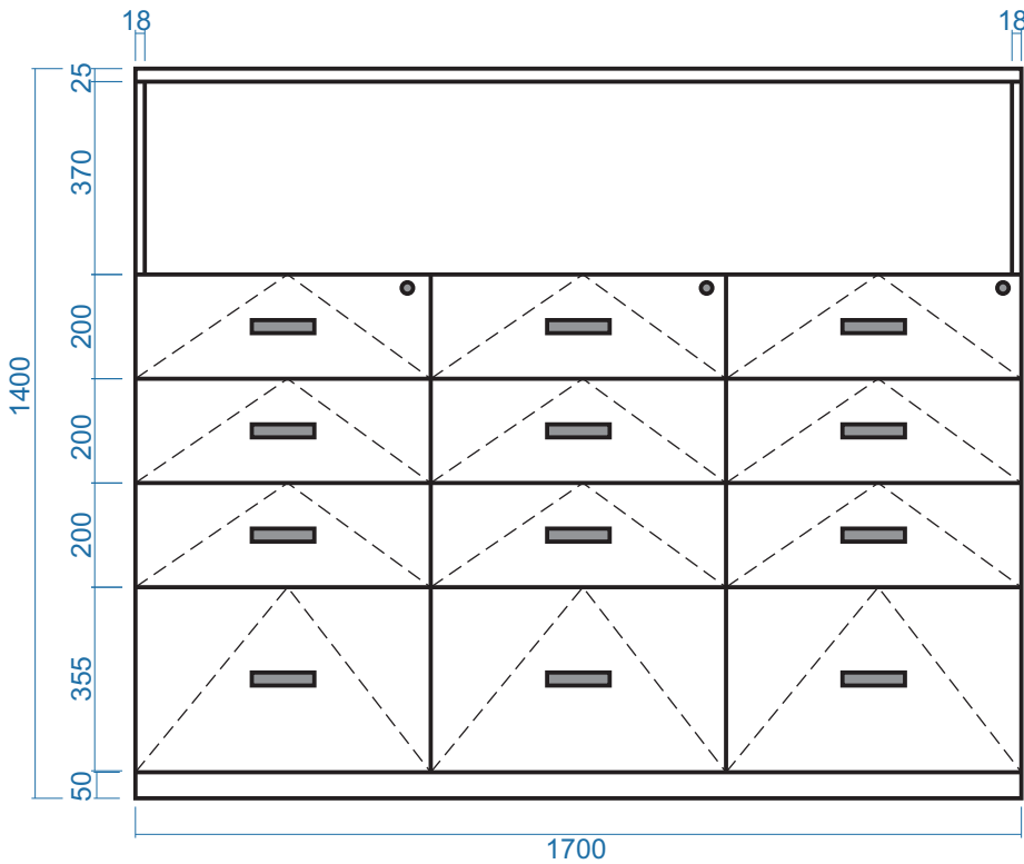
MẶT ĐỨNG
