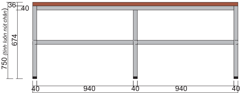
MẶT ĐỨNG
