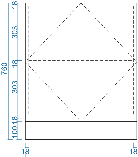
MẶT ĐỨNG
