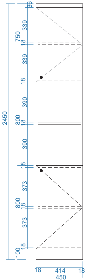
MẶT ĐỨNG
