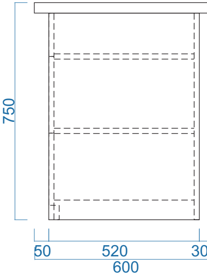
MẶT BÊN
