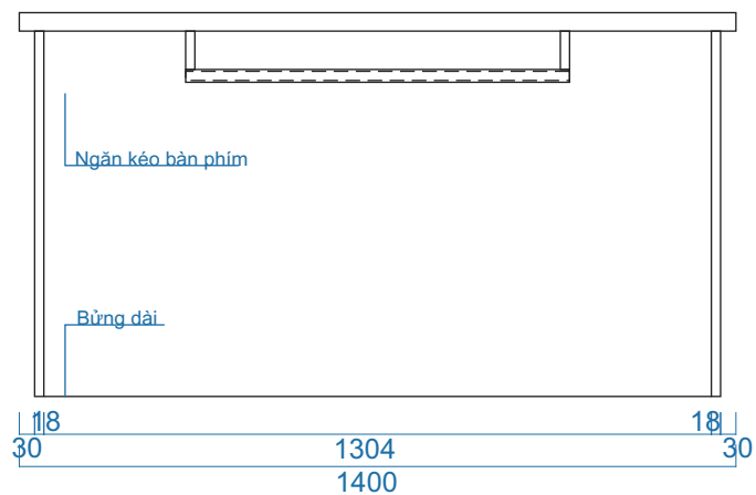
MẶT ĐỨNG
