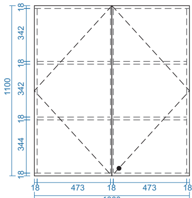
MẶT ĐỨNG
