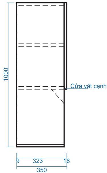
MẶT BÊN
