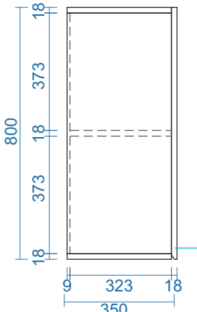
MẶT BÊN
