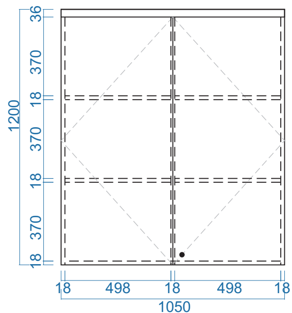
MẶT ĐỨNG
