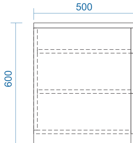
MẶT BÊN
