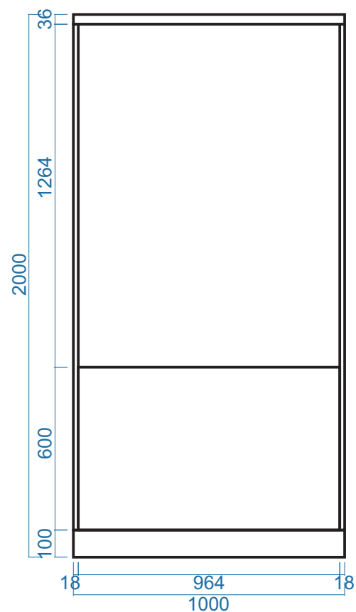
MẶT ĐỨNG
