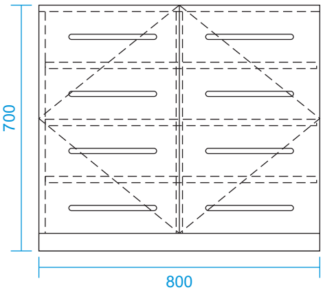
MẶT ĐỨNG
