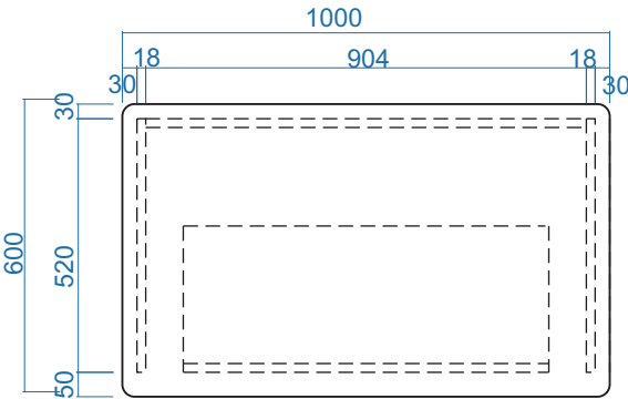
MẶT BẰNG
