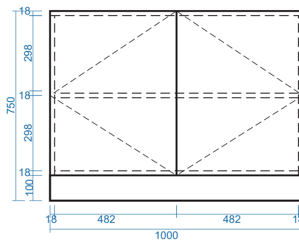
MẶT ĐỨNG
