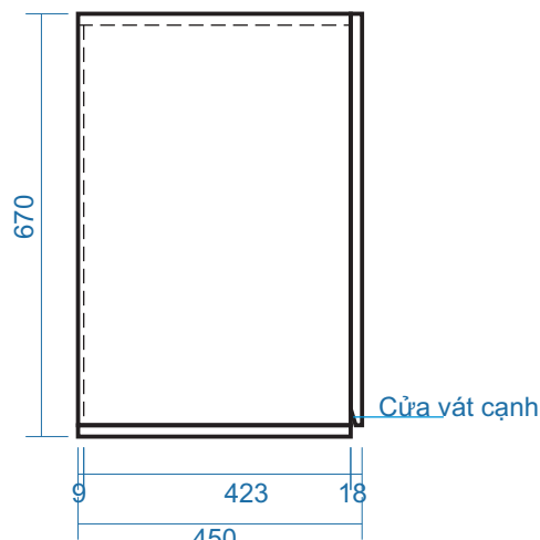
MẶT BÊN
