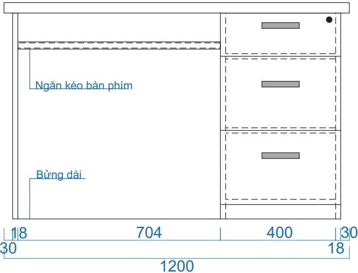
MẶT ĐỨNG
