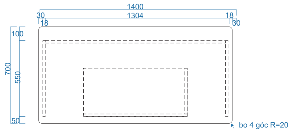
MẶT BẰNG
