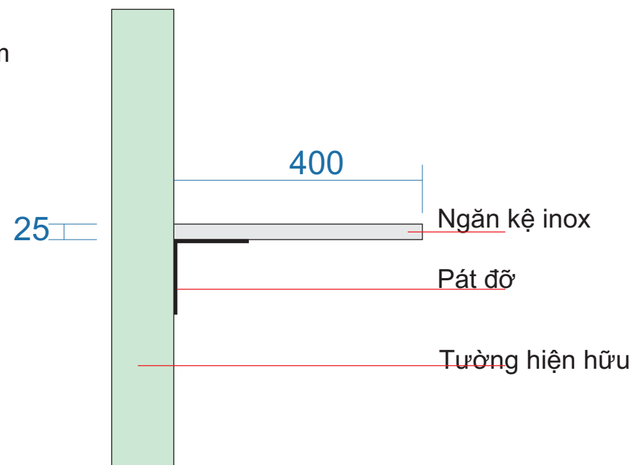
MẶT BÊN
