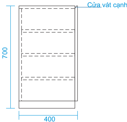
MẶT BÊN
