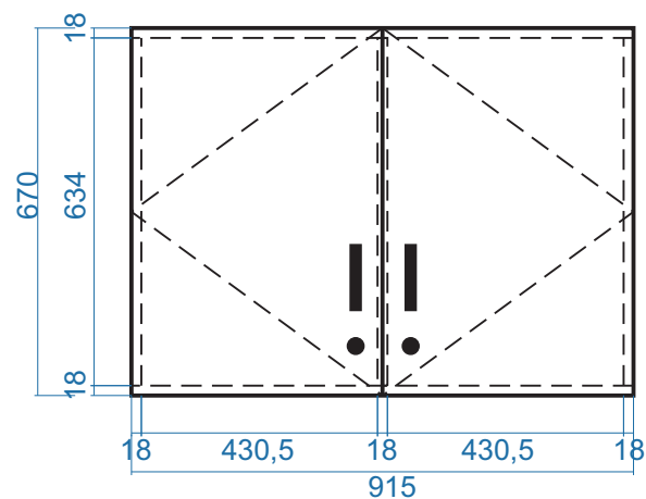
MẶT ĐỨNG
