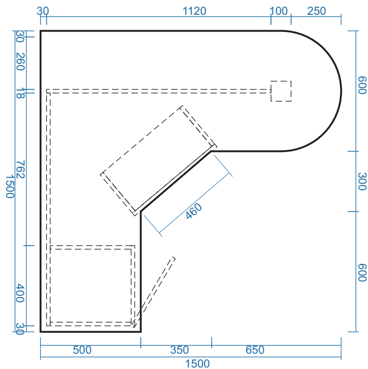
MẶT BẰNG
