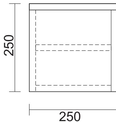
MẶT BÊN
