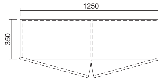
MẶT BẰNG
