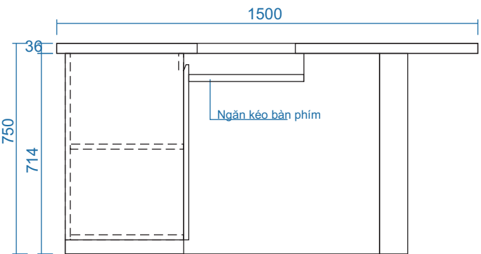
MẶT ĐỨNG
