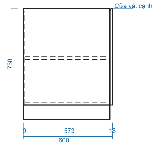
MẶT BÊN
