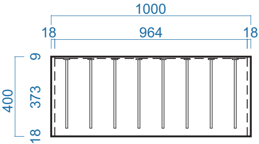
MẶT BẰNG
