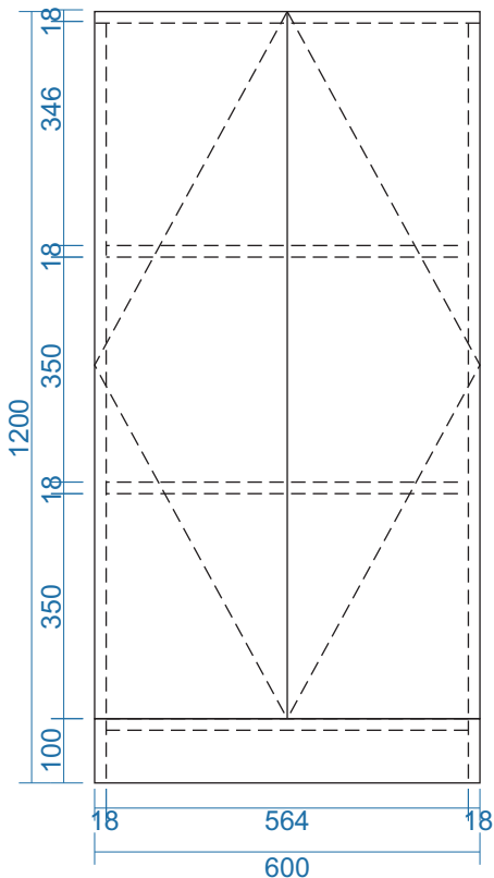
MẶT ĐỨNG
