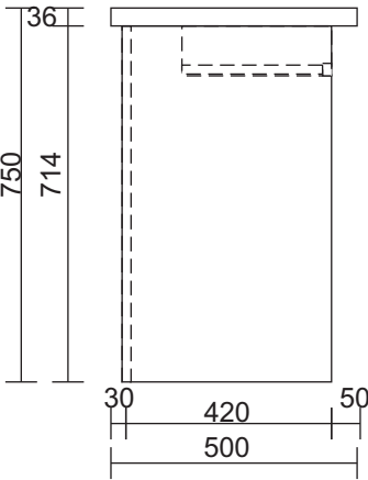
MẶT BÊN
