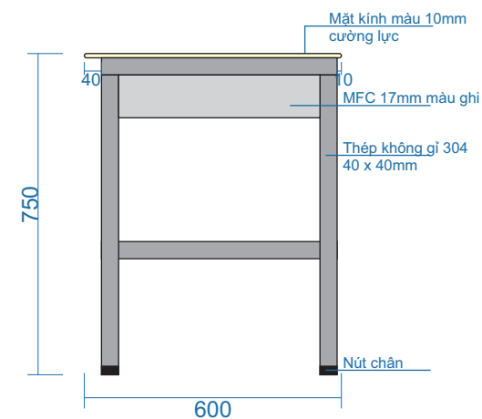
MẶT BÊN
