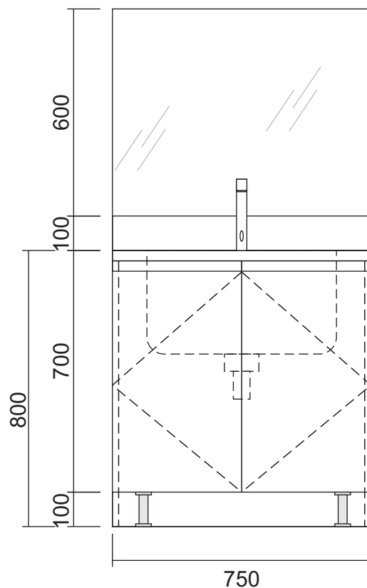
MẶT ĐỨNG
