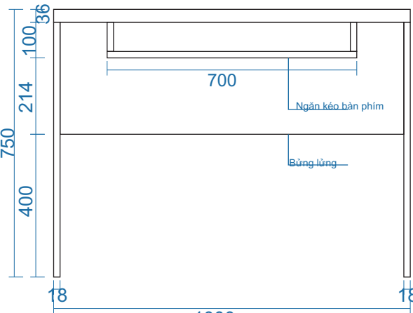
MẶT ĐỨNG
