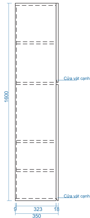
MẶT BÊN
