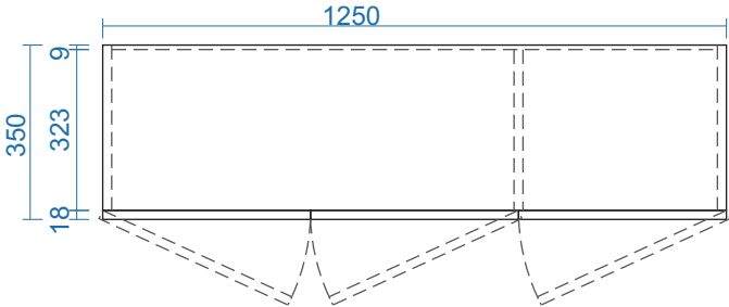
MẶT BẰNG
