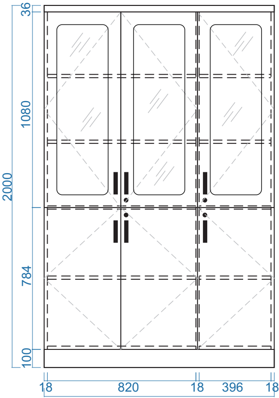
MẶT ĐỨNG
