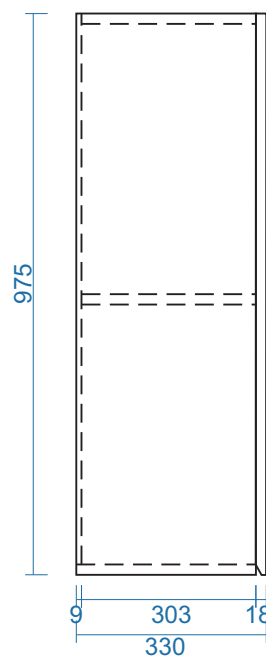
MẶT BÊN
