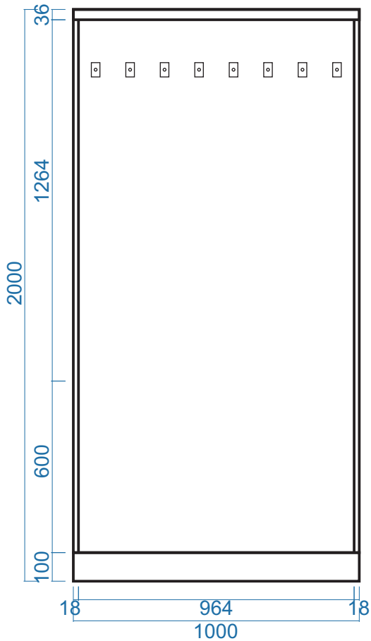
MẶT ĐỨNG
