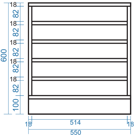
MẶT ĐỨNG
