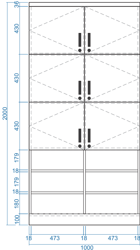
MẶT ĐỨNG
