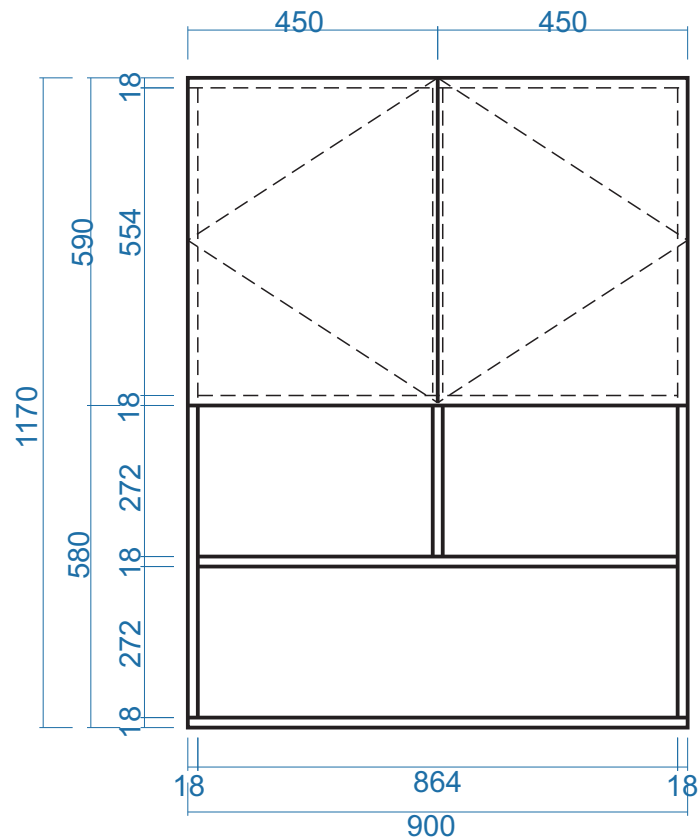
MẶT ĐÚNG
