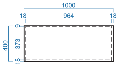
MẶT BÀNG
