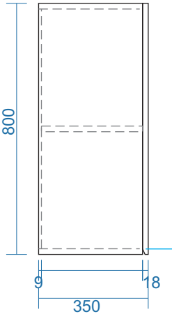
MẶT BÊN
