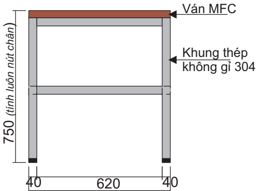
MẶT BÊN
