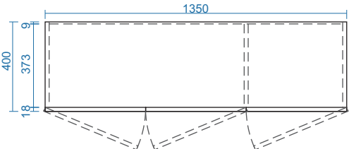
MẶT BẰNG
