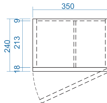
MẶT BẰNG
