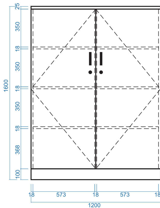
MẶT ĐỨNG
