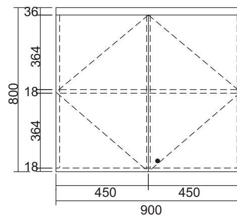
MẶT ĐỨNG
