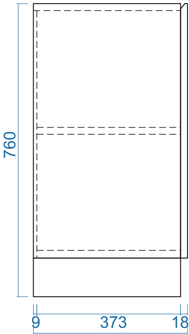
MẶT BÊN
