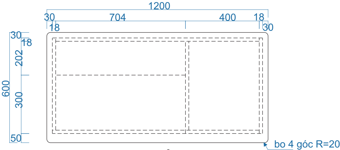
MẶT BẰNG
