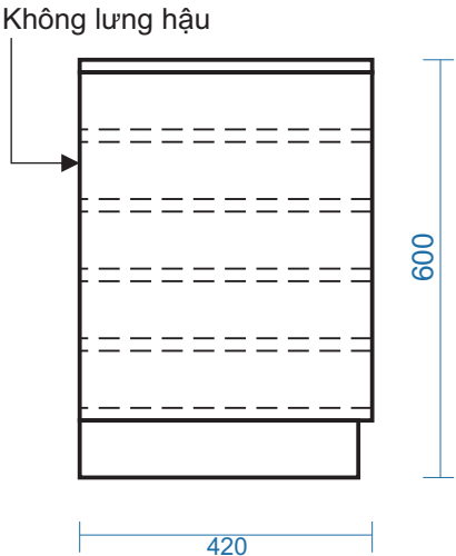
MẶT BÊN
