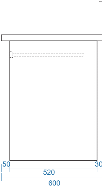
MẶT BÊN
