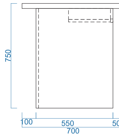
MẶT BÊN
