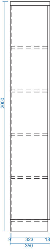
MẶT BÊN
