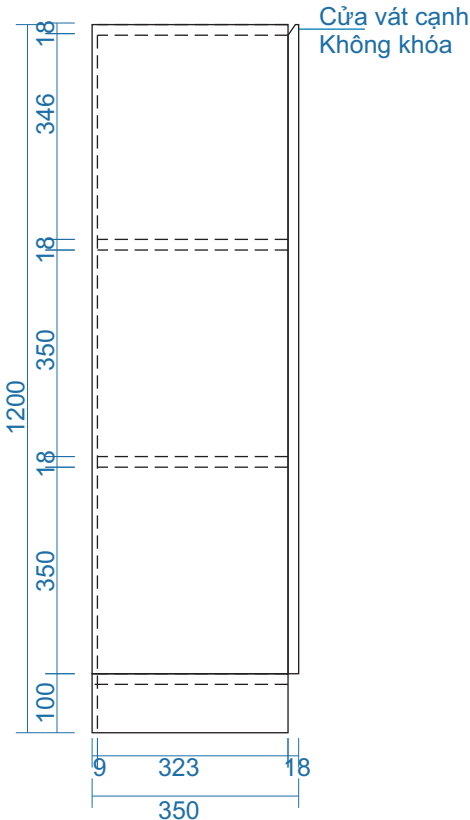
MẶT BÊN
