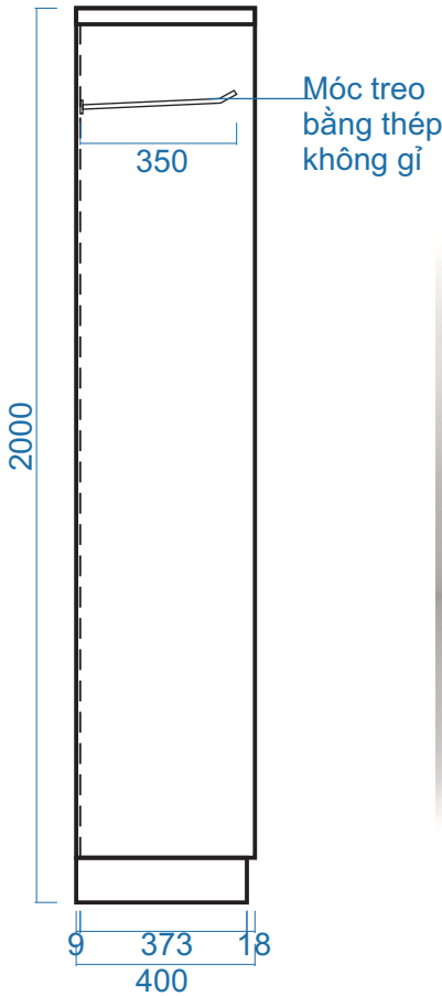
MẶT BÊN
