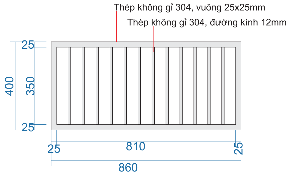
MẶT BẰNG
