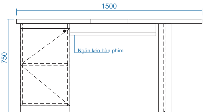
MẶT ĐỨNG
