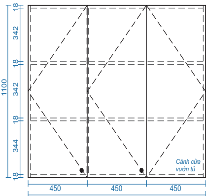
MẶT ĐỨNG
