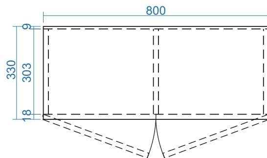
MẶT BẰNG
