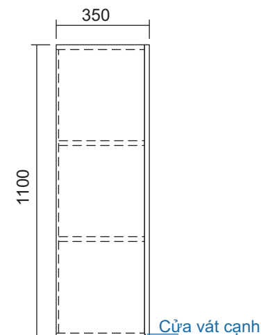
MẶT BÊN
