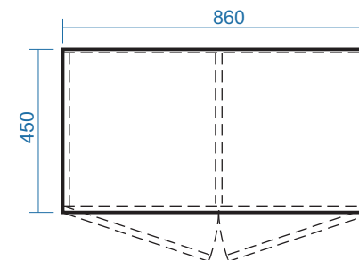
MẶT BẰNG
