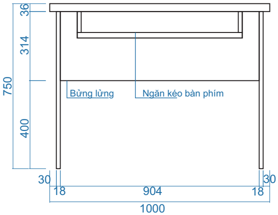
MẶT ĐỨNG
