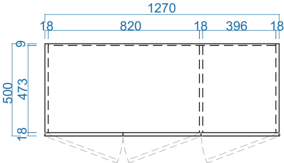
MẶT BẰNG
