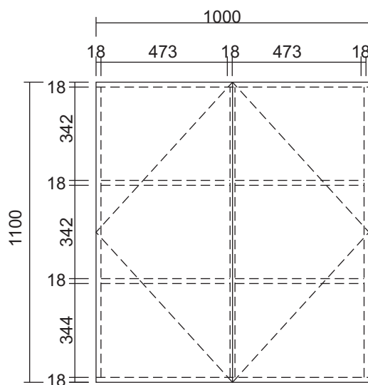
MẶT ĐỨNG
