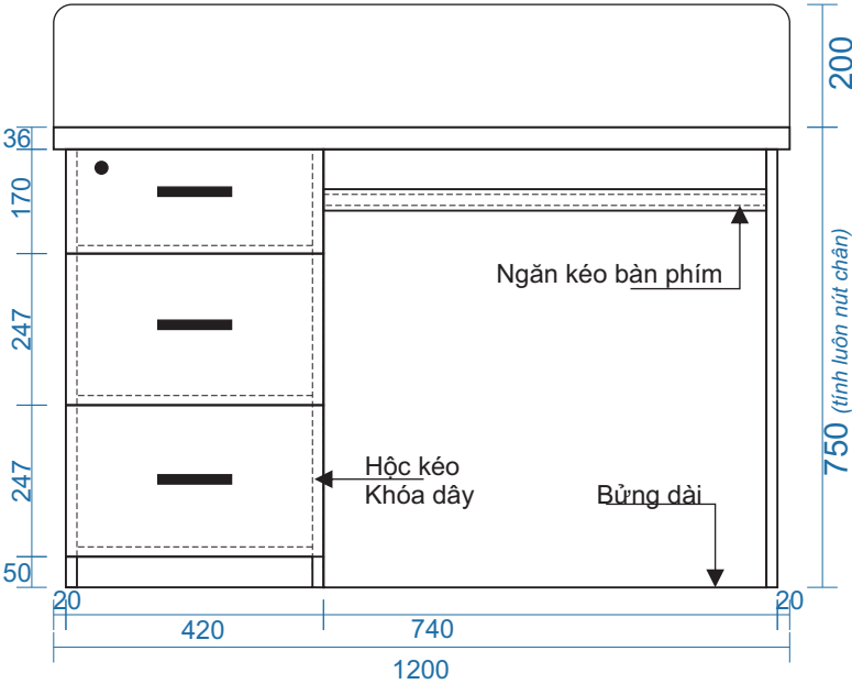
MẶT ĐỨNG
