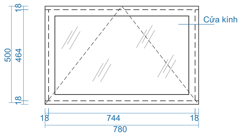
MẶT ĐỨNG
