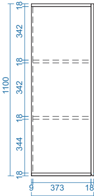
MẶT BÊN
