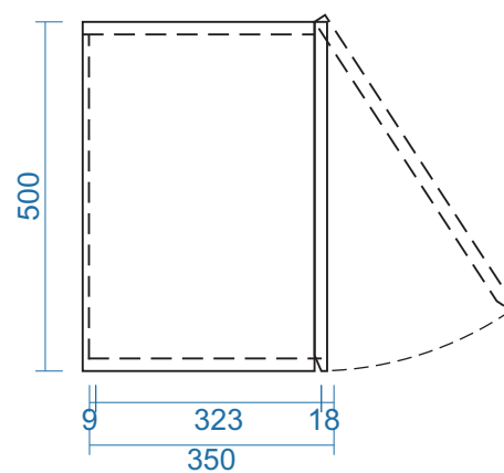
MẶT BÊN
