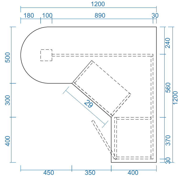
MẶT BẰNG
