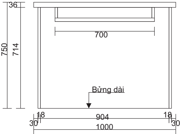
MẶT ĐỨNG
