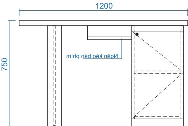
MẶT ĐỨNG
