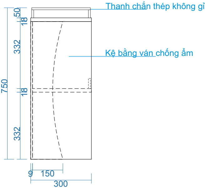
MẶT BÊN
