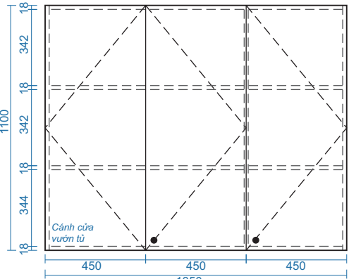
MẶT ĐỨNG
