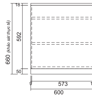
MẶT BÊN
