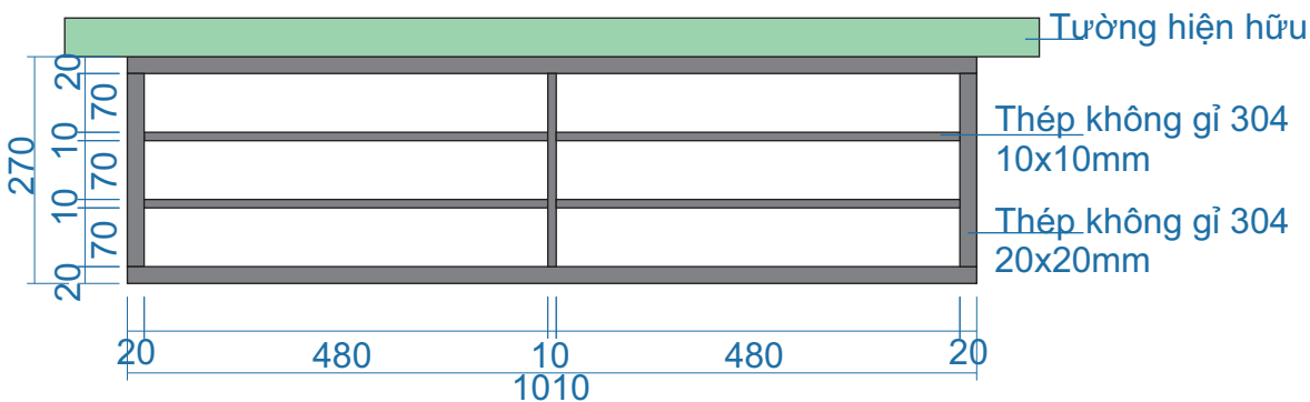
MẶT BẰNG
