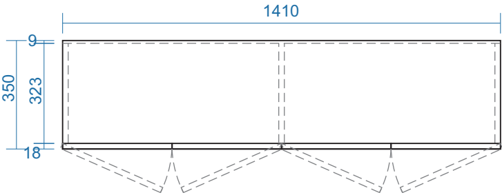
MẶT BẰNG
