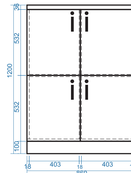
MẶT ĐỨNG
