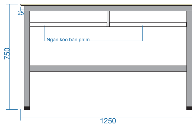
MẶT ĐỨNG
