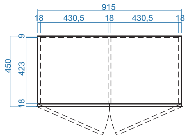
MẶT BẰNG
