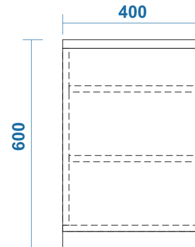
MẶT BÊN
