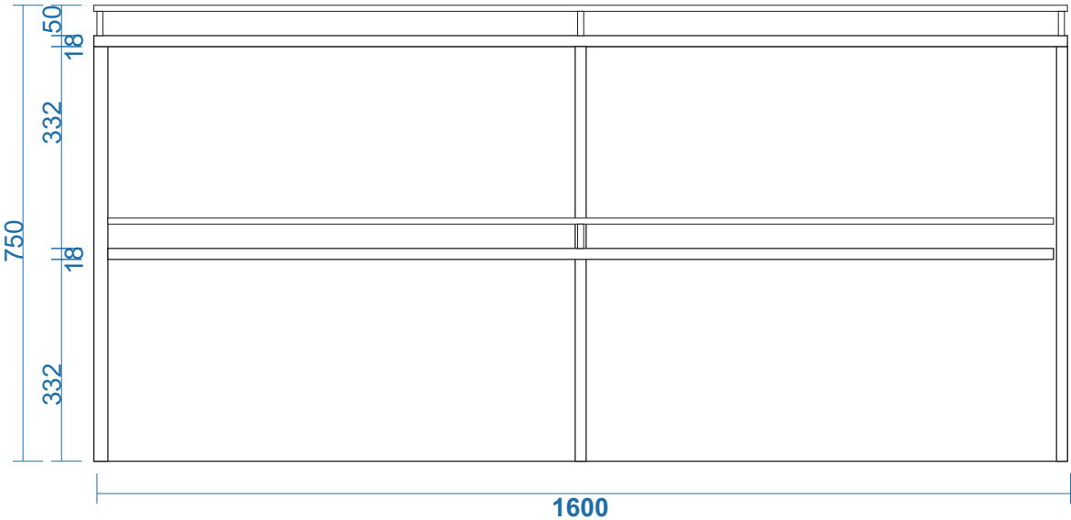
MẶT ĐỨNG
