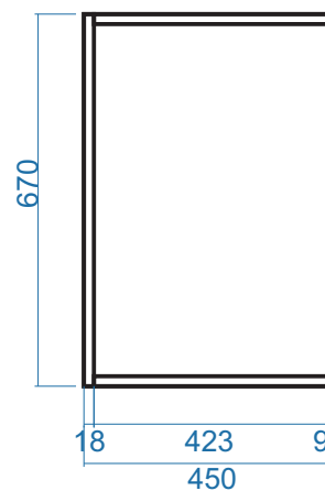
MẶT BÊN
