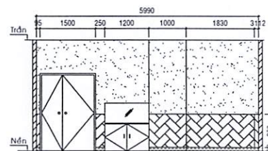
Hướng nhìn 5
