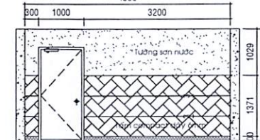
HƯỚNG NHÌN 8
