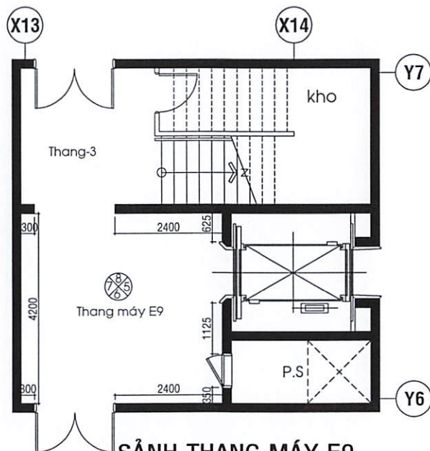
SẢNH THANG MÁY E9 (Hầm 2)
