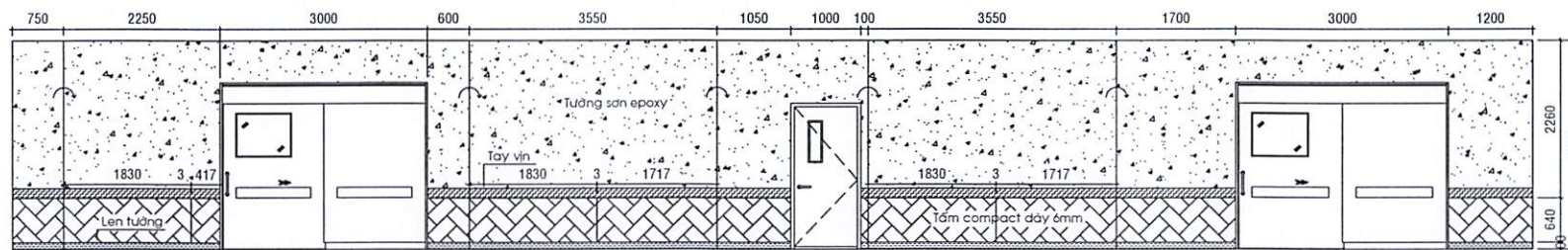
HƯỚNG NHÌN 10 LẦU 2
