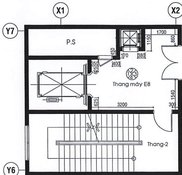
SẢNH THANG MÁY E8 (Lầu 3)
