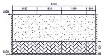
Hướng nhìn 2
