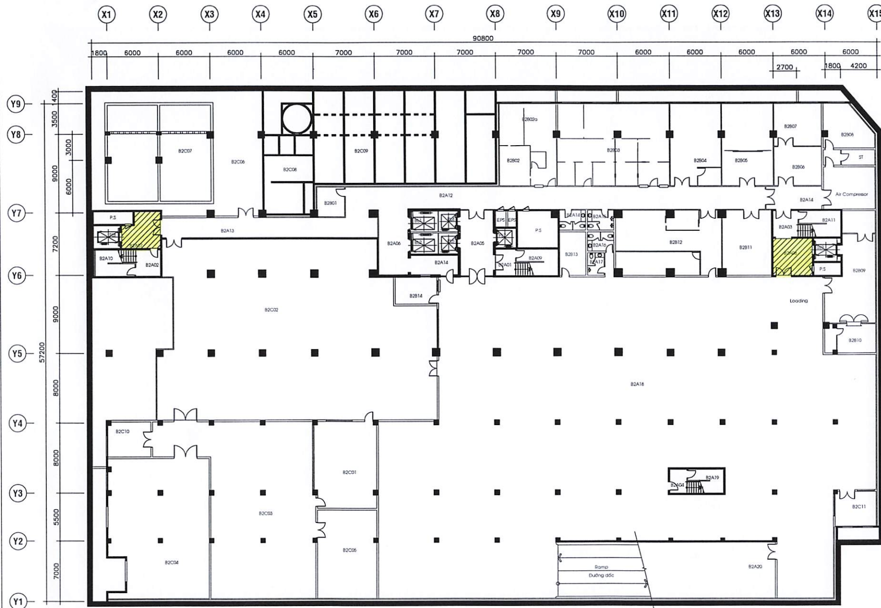
MẶT BẰNG TẦNG HẦM 2
