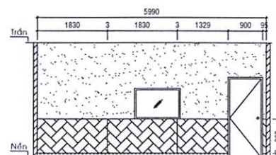
Hướng nhìn 7
