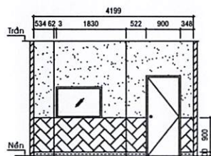
Hướng nhìn 1
