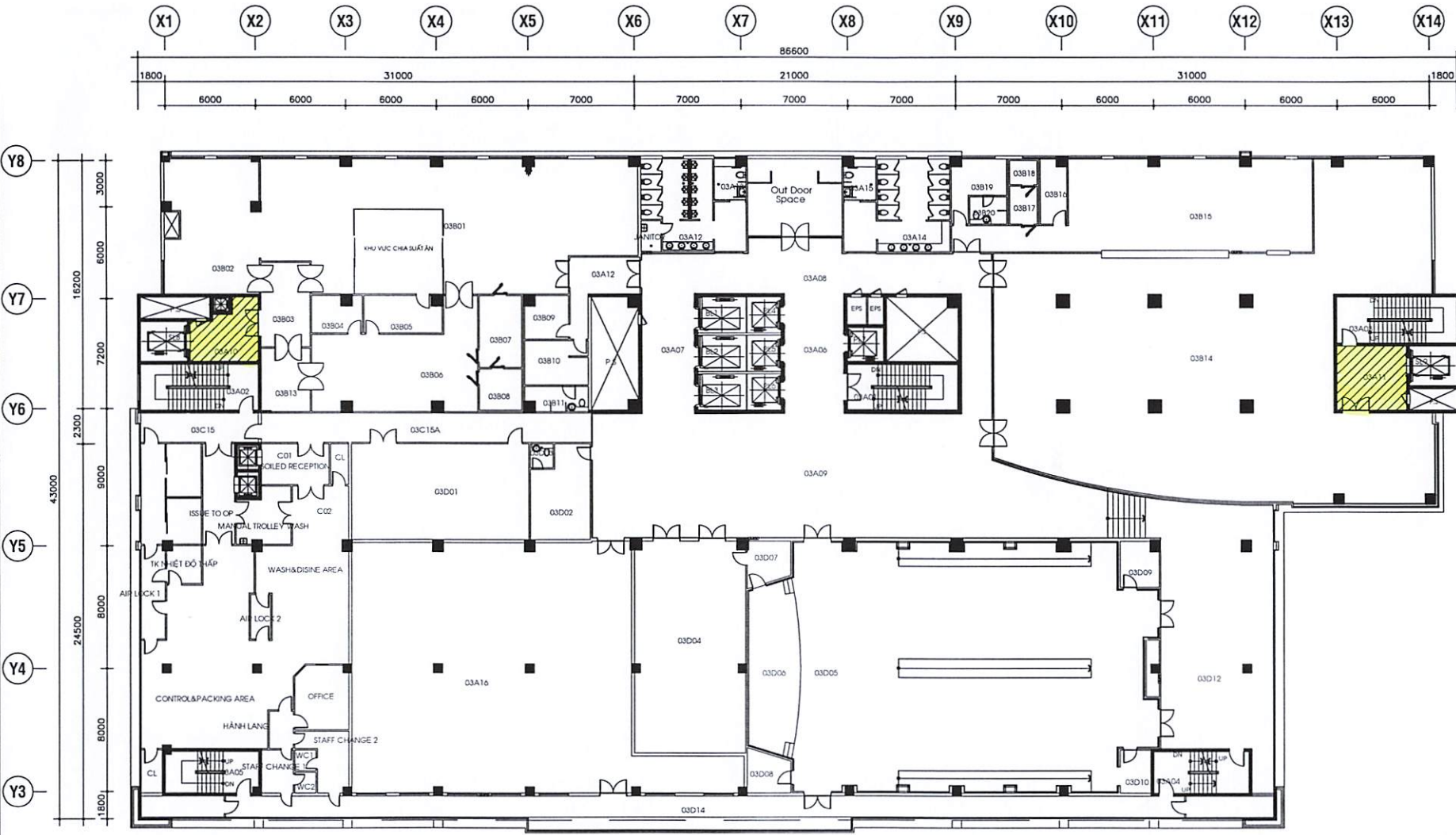
MẶT BẰNG LẦU 3
