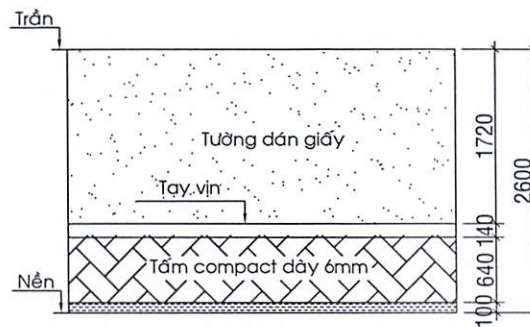
MẶT ĐỨNG ĐIỂN HÌNH LẦU 6
