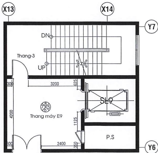
SẢNH THANG MÁY E9 (Lầu 3)
