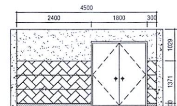
HƯỚNG NHÌN 6
