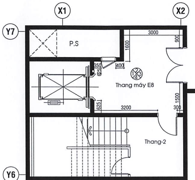
SẢNH THANG MÁY E8 (Hầm 1)
