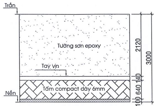
MẶT ĐỨNG ĐIỂN HÌNH LẦU 2
