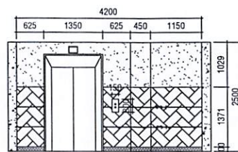
HƯỚNG NHÌN 1
