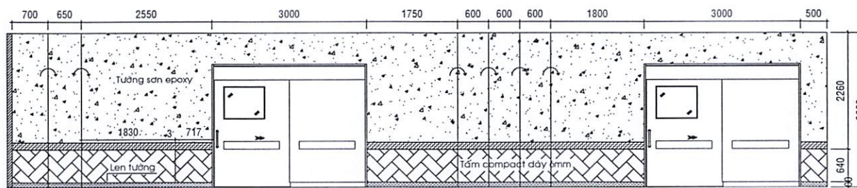
HƯỚNG NHÌN 6 LẦU 2
