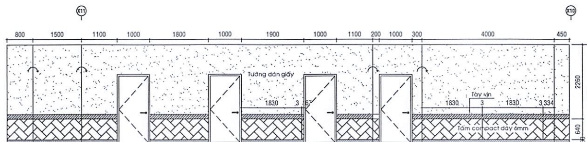
HƯỚNG NHÌN II LẦN 6
