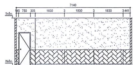
Hướng nhìn 8
