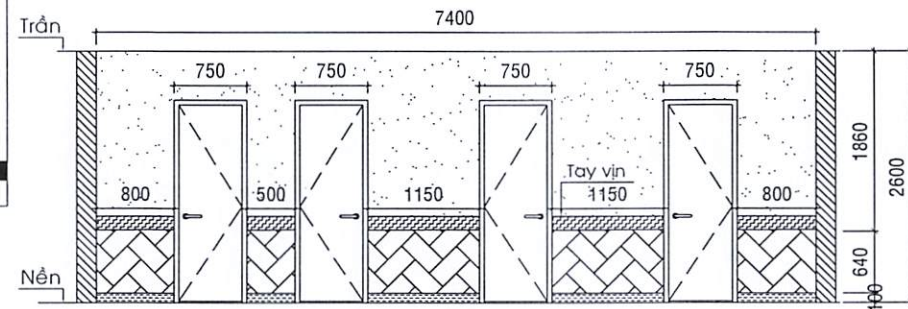
HƯỚNG NHÌN 3
