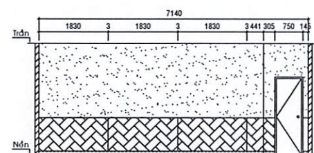
Hướng nhìn 8
