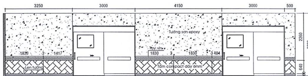
HƯỚNG NHÌN 8 LẦU 2
