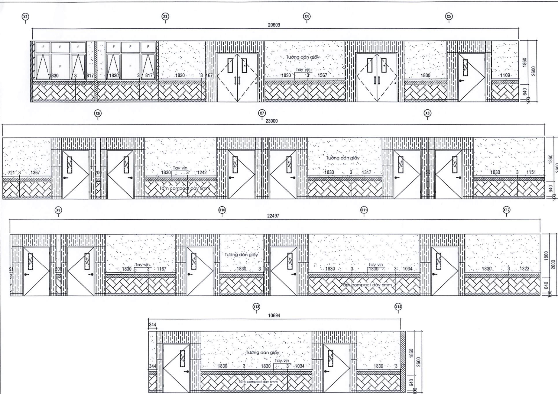
HƯỚNG NHÌN A LẦU 7
