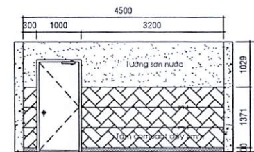
HƯỚNG NHÌN 4
