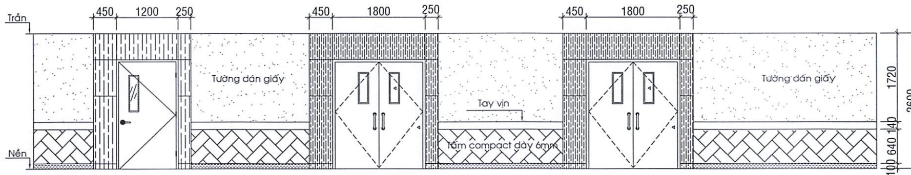
MẶT ĐỨNG ĐIỂN HÌNH HÀNH LANG LẦU 7-14
