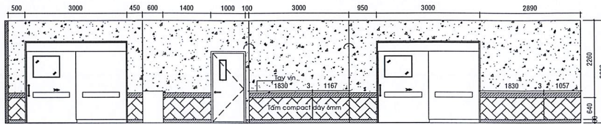
HƯỚNG NHÌN 7 LẦU 2
