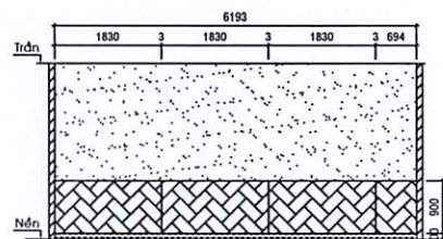
Hướng nhìn 2
