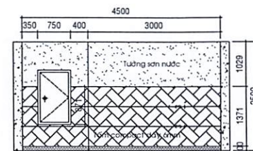
HƯỚNG NHÌN 2
