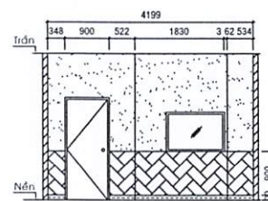
Hướng nhìn 5
