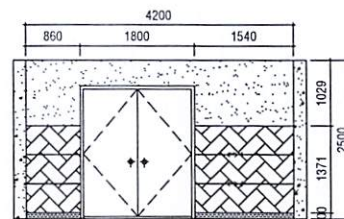
HƯỚNG NHÌN 3
