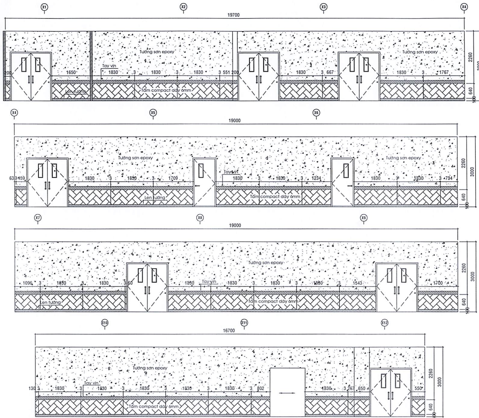
HƯỚNG NHÌN 1 LẦU 2
