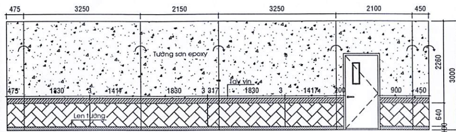
HƯỚNG NHÌN 3 LẦU 2
