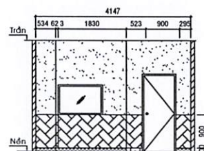
Hướng nhìn 5
