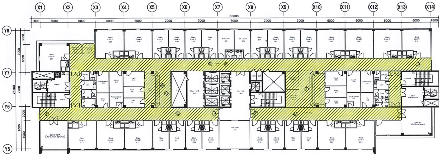
MẶT BẰNG LẦU 8 - 13
