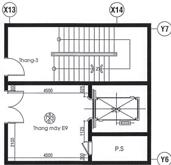
SẢNH THANG MÁY E9 (Hầm 1)
