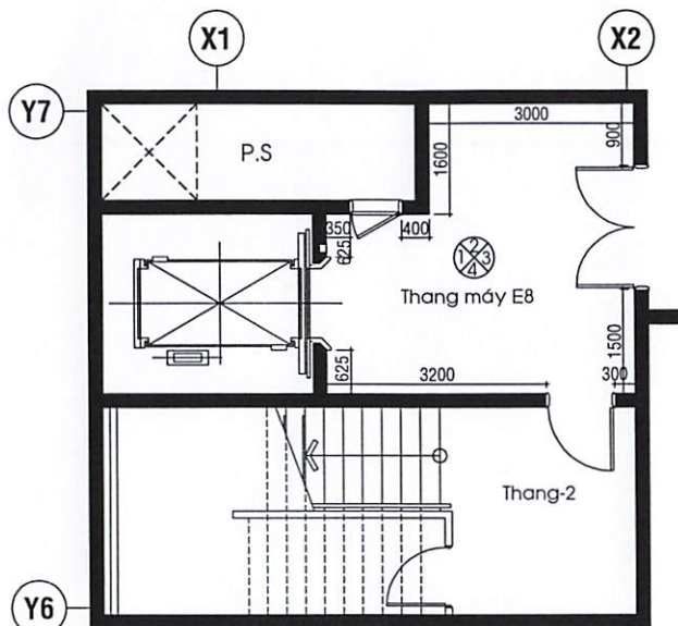
SẢNH THANG MÁY E8 (Hầm 2)
