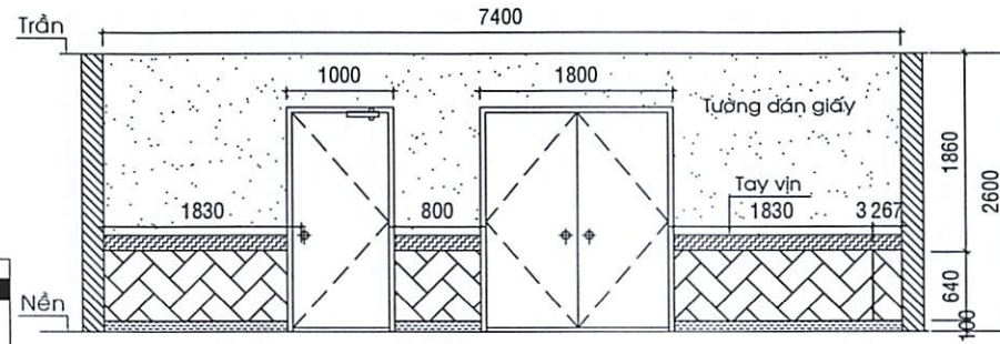
HƯỚNG NHÌN 1
