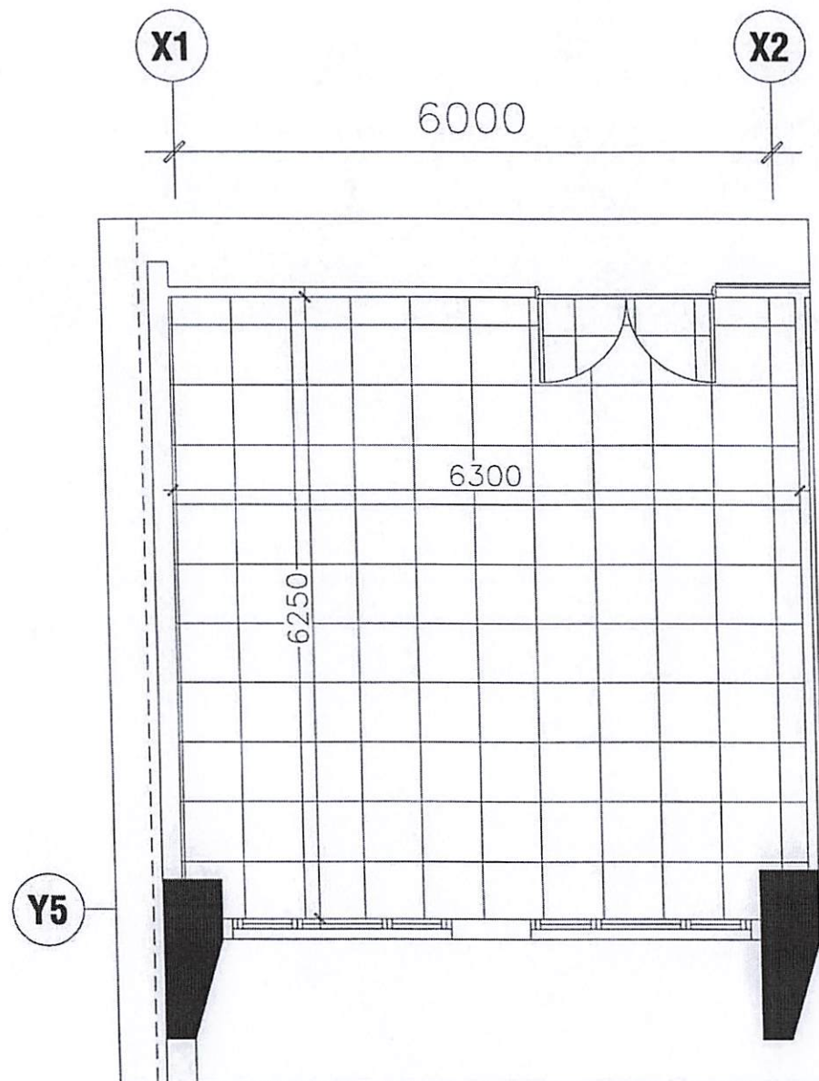
MẶT BẰNG LÓT THẨM PHÒNG 401 LẦU 4
