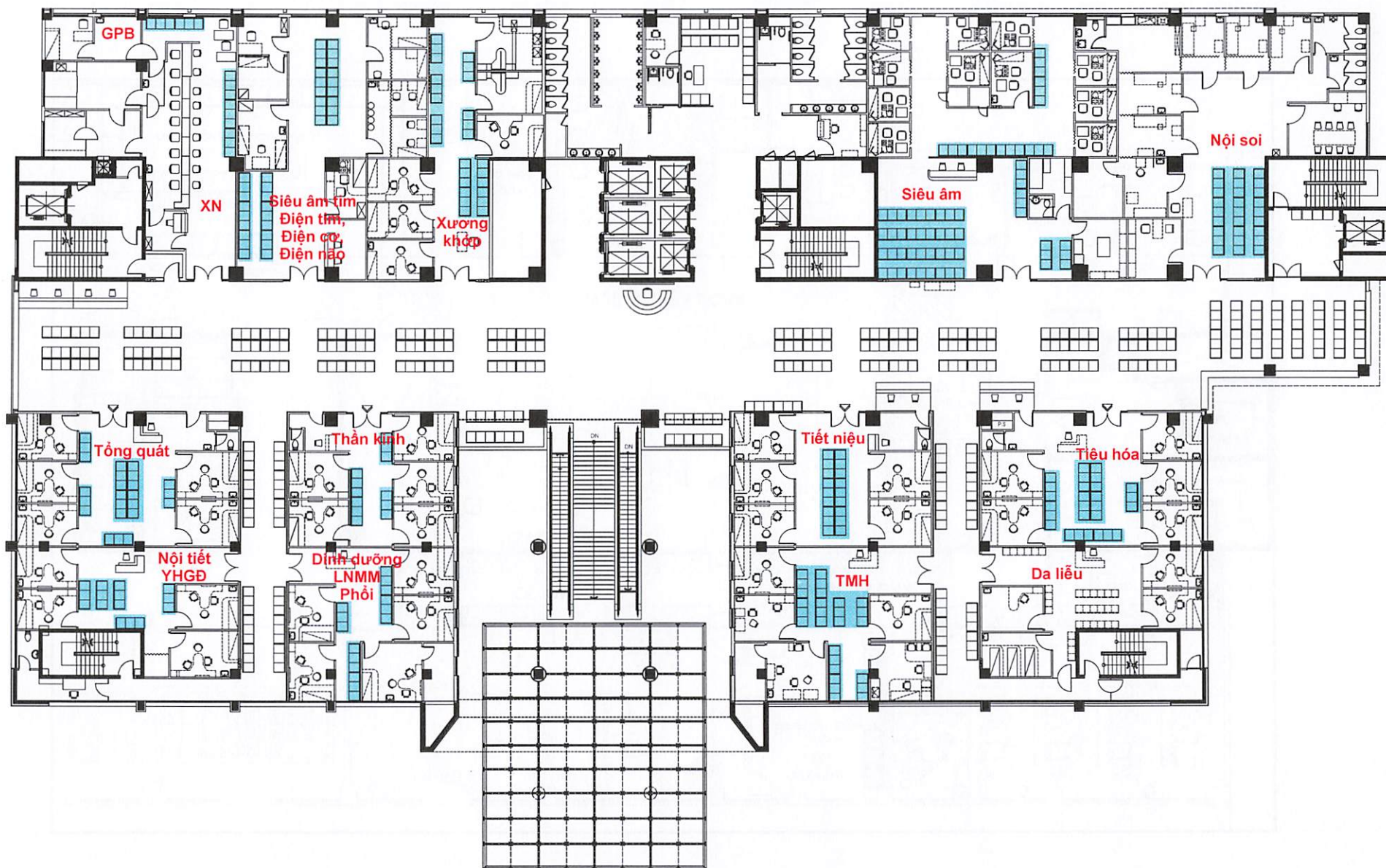
MẶT BẰNG BỐ TRÍ GHẾ BẰNG TẠI LẦU 1 KHU A
