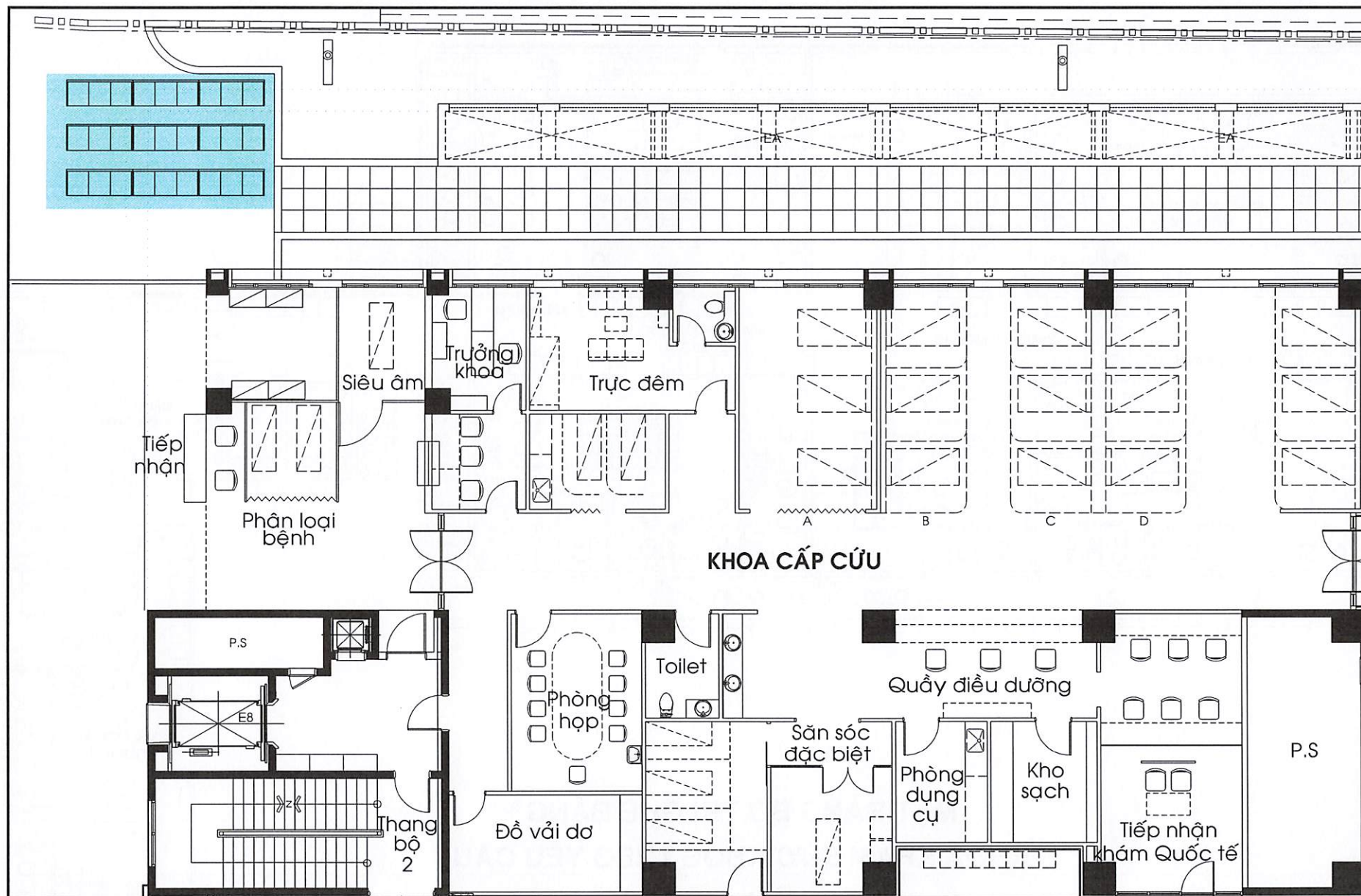
MẶT BẰNG BỐ TRÍ GHẾ BẰNG KHOA CẤP CỨU
