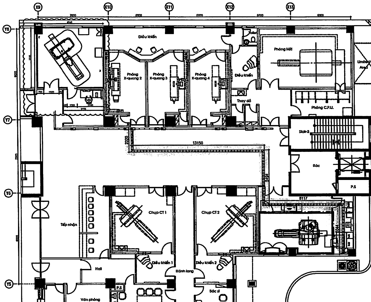
MẶT BẰNG CẤP NGUỒN PHÒNG MRI 2
