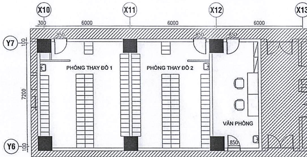
MẶT BẰNG HIỆN TRẠNG KHU VỰC PHÒNG THAY ĐỒ TẦNG HÀM 1
