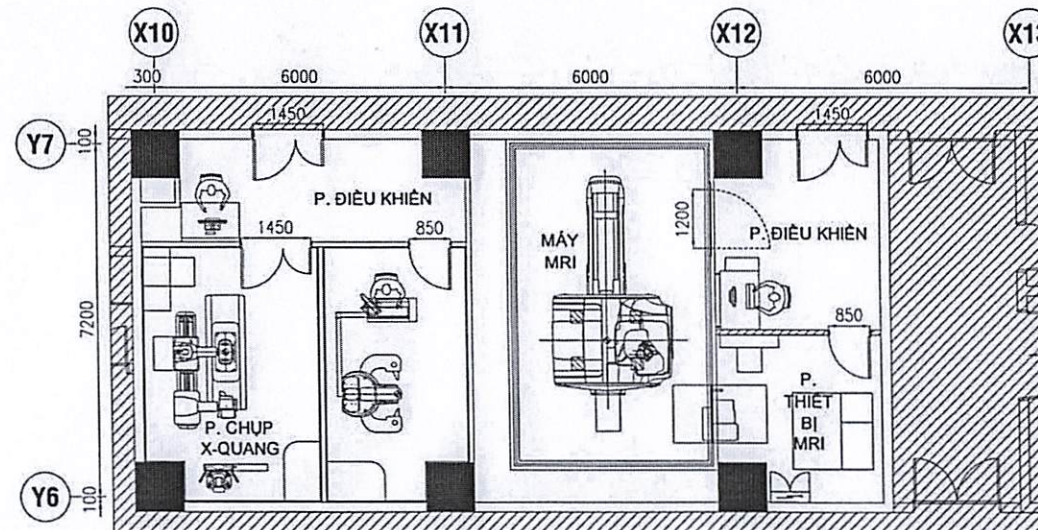
MẶT BẰNG CẢI TẠO KHU VỰC PHÒNG THAY ĐỒ TẦNG HÀM 1 THÀNH PHÒNG MRI VÀ PHÒNG CHỤP XQUANG
