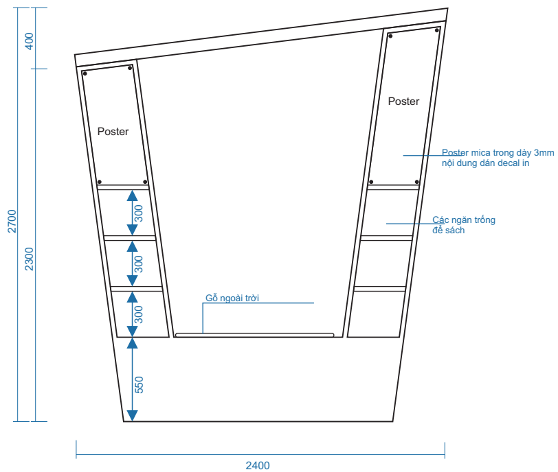
MẶT BÊN
