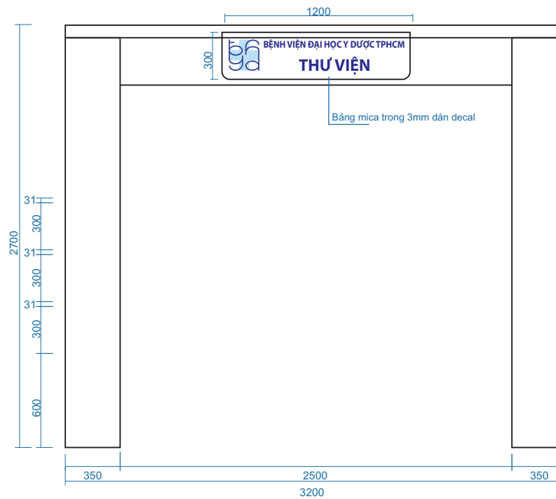
MẶT ĐÚNG
