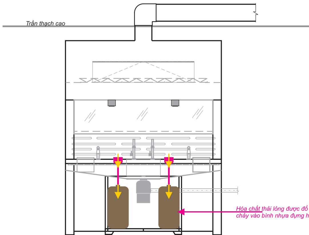
MẶT ĐỨNG
