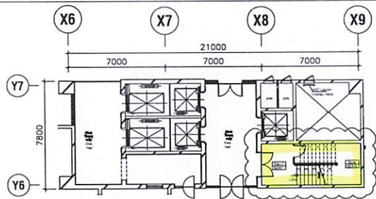
MẶT BẰNG THANG SỐ 1 (HẦM 2-HẦM 1)
