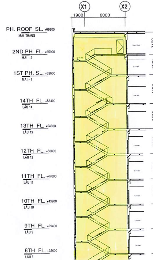
MẶT CẮT THANG SỐ 2 ( LẦU 8 ~ MÁI)
