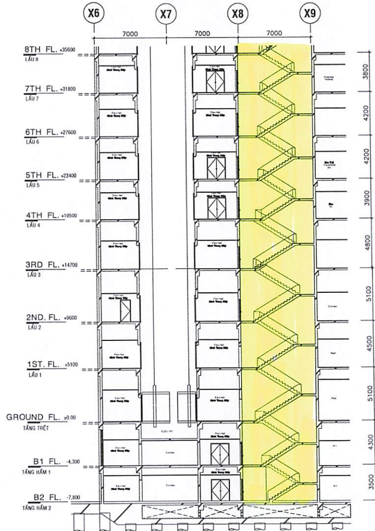
MẶT CẮT THANG SỐ 1 (HẦM 2-LẦU 8)
