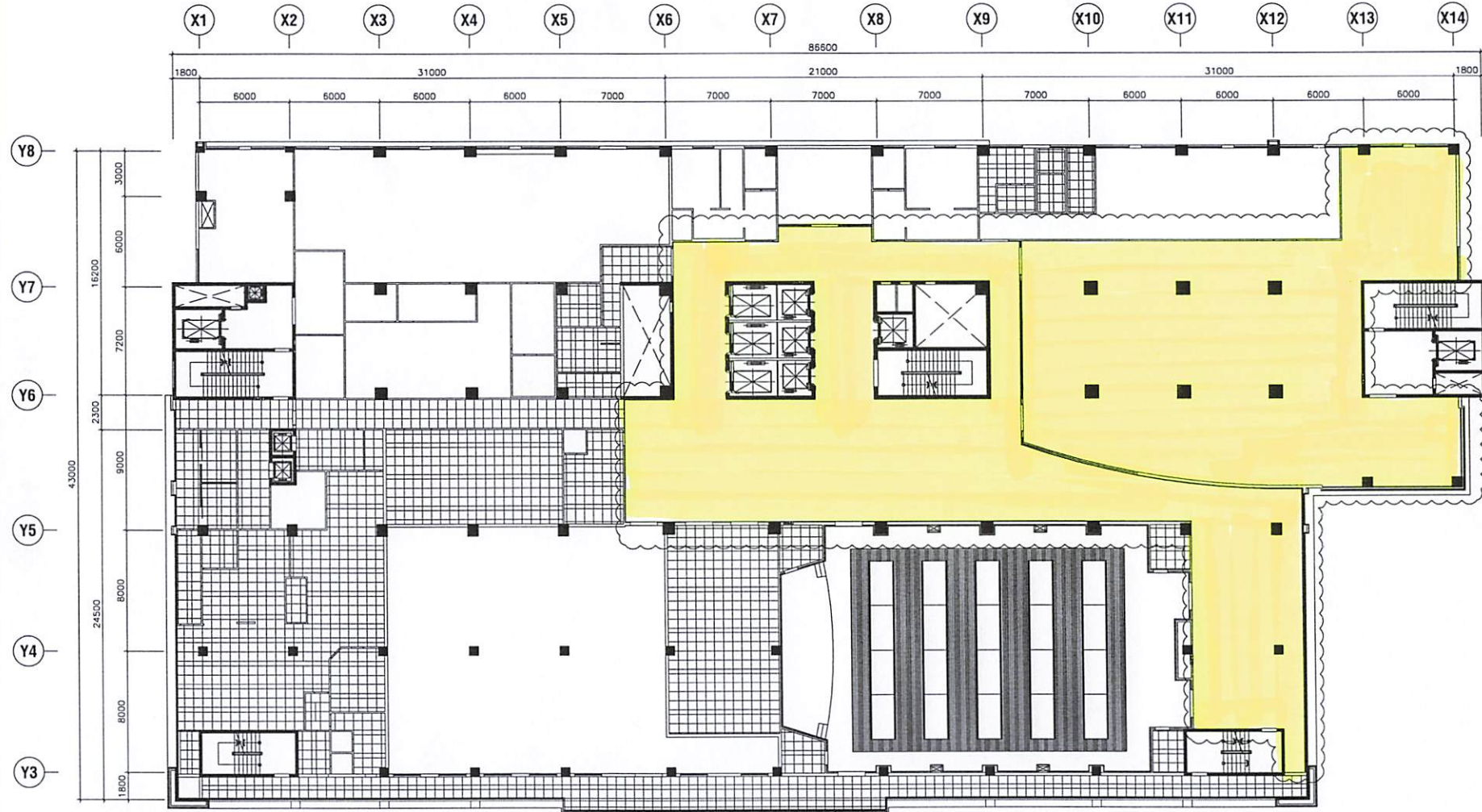
MẶT BẰNG TRẦN LẦU 3
