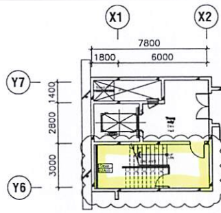
MẶT BẰNG THANG SỐ 2 (HẦM 2~HẦM 1)
