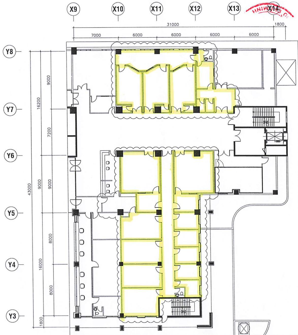
MẶT BẰNG KHOA CHẨN ĐOÁN HÌNH ẢNH TẦNG TRỆT
