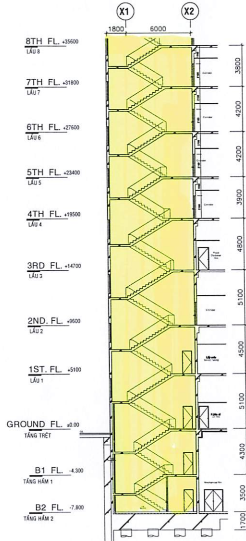
MẶT CẮT THANG SỐ 2 ( HẦM 2~ LẦU 8)
