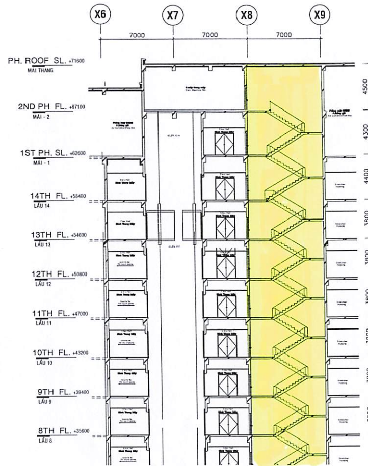
MẶT CẮT THANG SỐ 1 (LẦU 8-MÁI)
