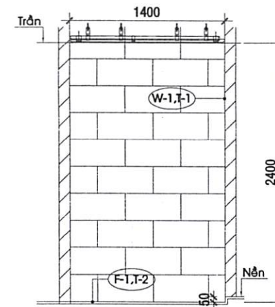
HƯỚNG NHÌN 4
