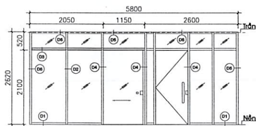
VÁCH KÍNH INOX HIỆN HỮU
