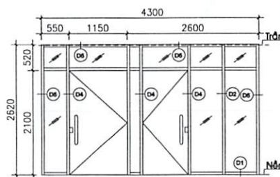
VÁCH KÍNH INOX SAU KHI SỬA CHỮA
