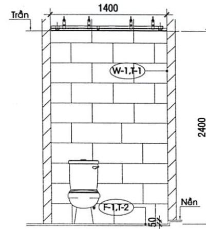
HƯỚNG NHÌN 2
