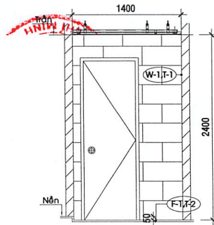
HƯỚNG NHÌN 1
