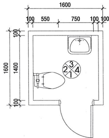
MẶT BẰNG NHÀ VỆ SINH LẦU 8
