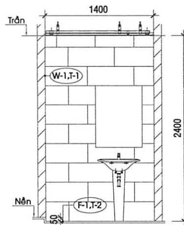
HƯỚNG NHÌN 3
