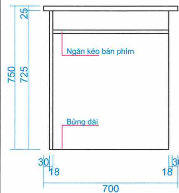
MẶT ĐỨNG
