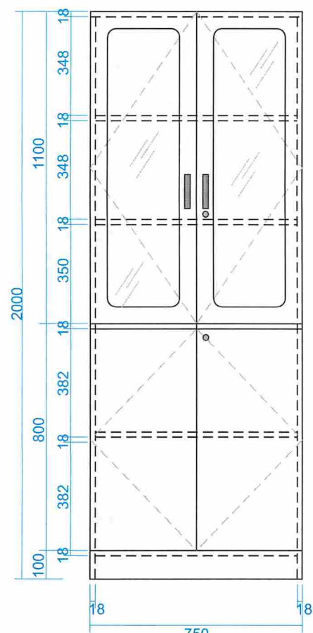
MẶT ĐỨNG
