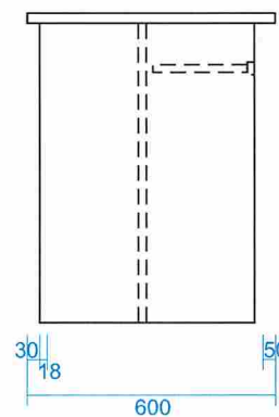
MẶT BÊN
