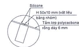
CHI TIẾT 1
