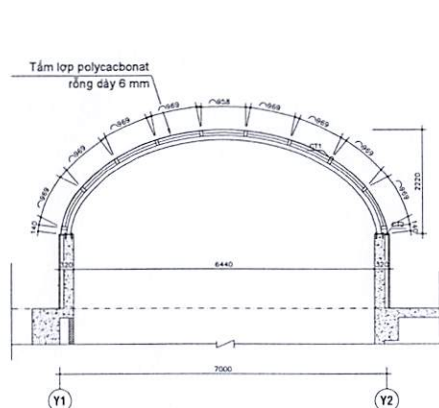
MẶT CẮT 2-2
