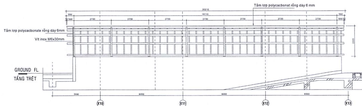
MẶT CẮT 1 - 1
