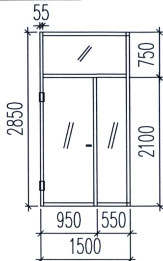
MẶT CHIẾU ĐỨNG HƯỚNG NHÌN 1
