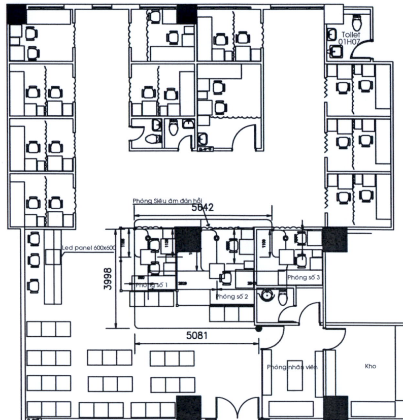
MẶT BẰNG LẮP ĐÈN PHÒNG SIÊU ÂM LẦU 1 KHU A TỈ LỆ : 1/100
