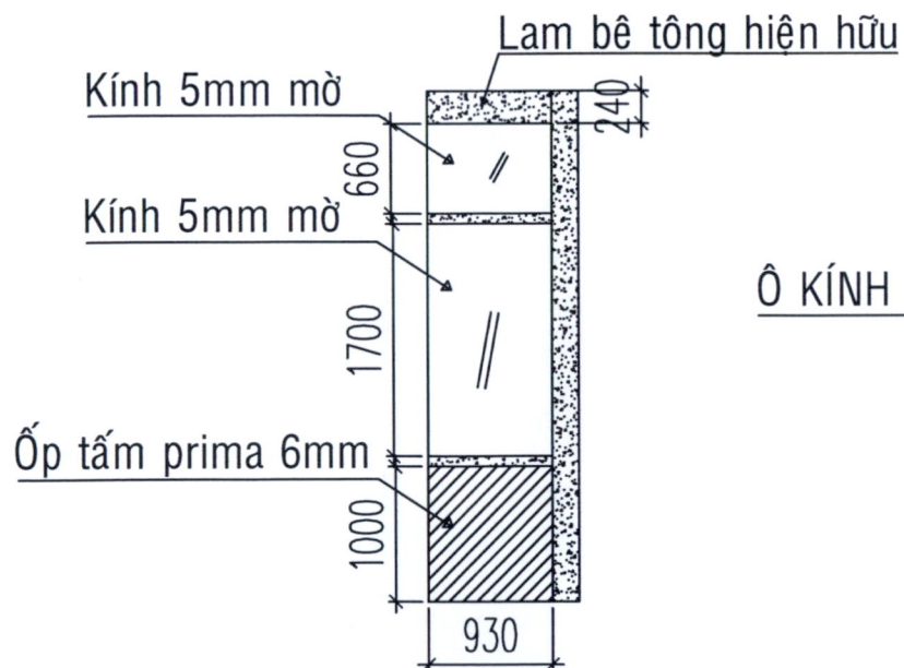
MẶT CHIẾU ĐỨNG HƯỚNG NHÌN 3
