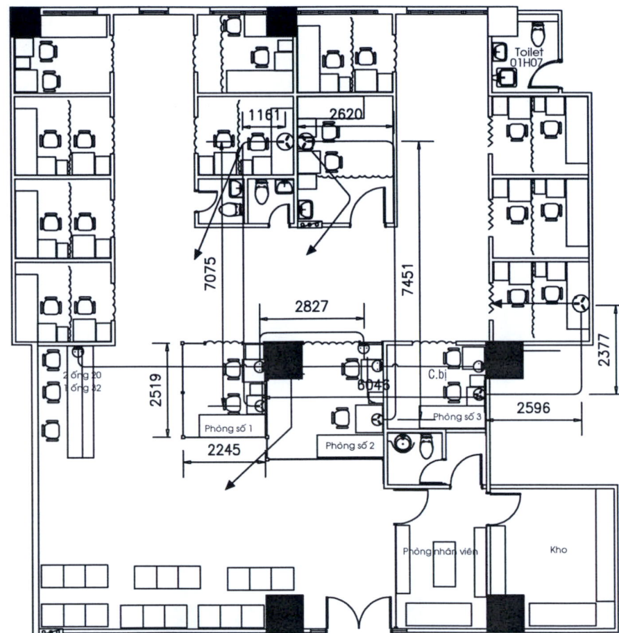
MẶT BẰNG LẮP ĐẶT Ổ CẮM ĐIỆN PHÒNG SIÊU ÂM LẦU 1 KHU A TỈ LỆ : 1/100
