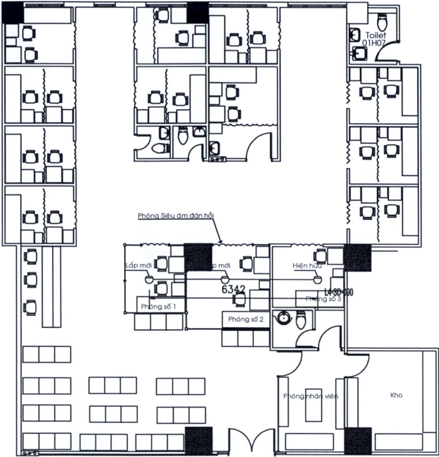
MẶT BẰNG LẮP ĐẦU BÁO KHÓI SIÊU ÂM LẦU 1 KHU A TỈ LỆ : 1/100
