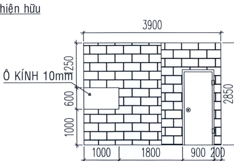
MẶT CHIẾU ĐỨNG HƯỚNG NHÌN 2
