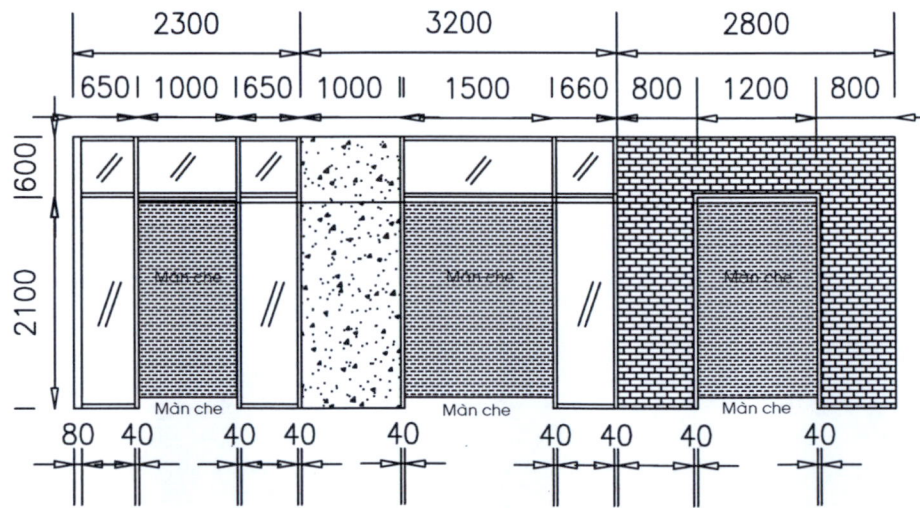
HÌNH CHIẾU 2
