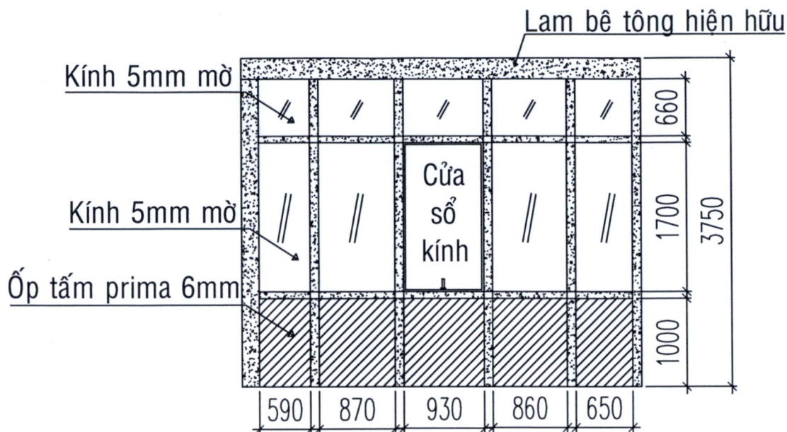
MẶT CHIẾU ĐỨNG HƯỚNG NHÌN 2
