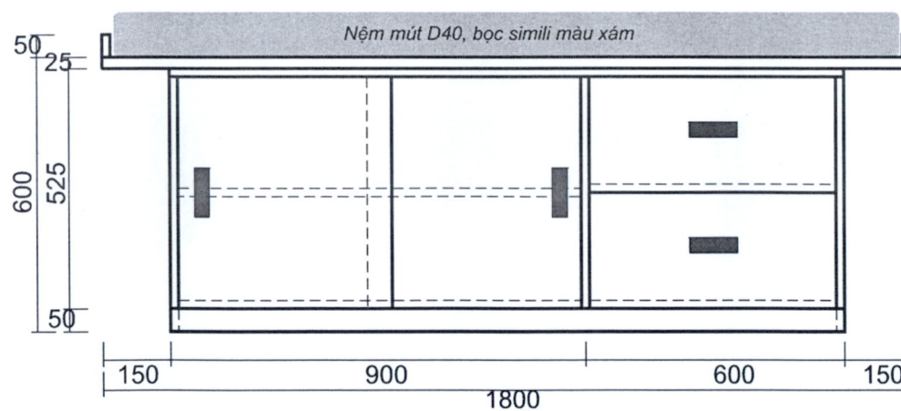
MẶT ĐỨNG
