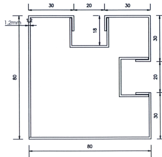
MẶT CẮT THANH 2 MẶT KÍNH
