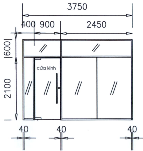
HÌNH CHIẾU 4
