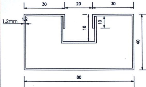
MẶT CẮT THANH 1 MẶT KÍNH
