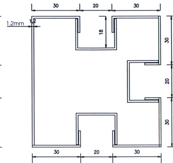
MẶT CẮT THANH 3 MẶT KÍNH
