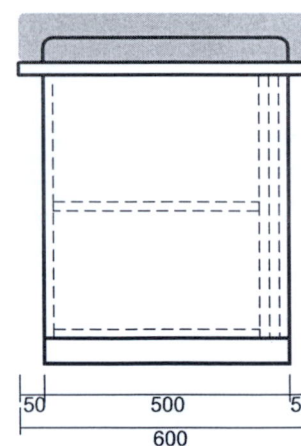
MẶT BÊN
