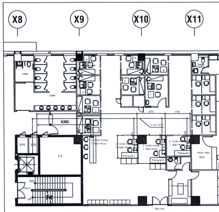
MẶT BẰNG LẮP ĐẶT MẠNG, ĐIỆN THOẠI SIÊU ÂM LẦU 1 KHU A
