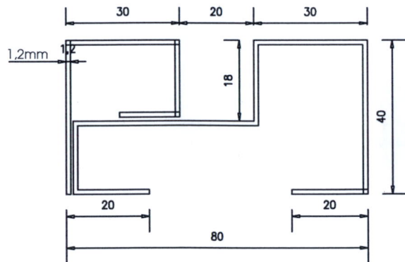
MẶT CẮT THANH DƯỚI CHÂN
