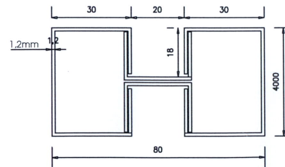
MẶT CẮT THANH GIỮA
