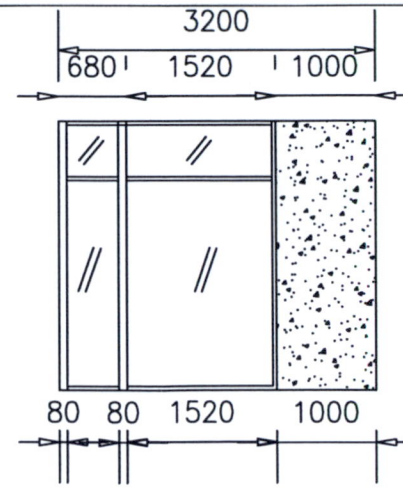
HÌNH CHIẾU 3
