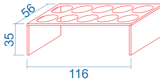
PHỐI CẢNH
