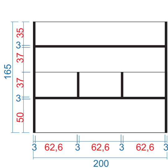
MẶT ĐỨNG
