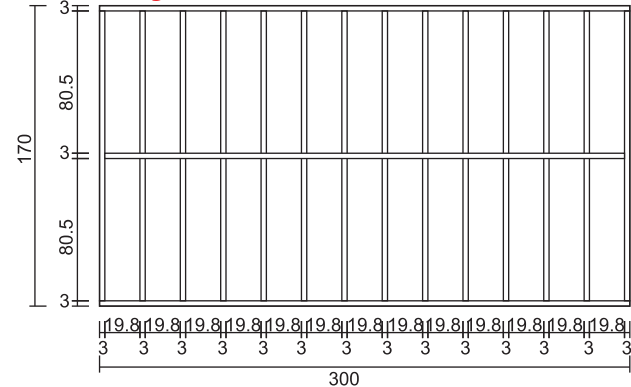
MẶT BẰNG
