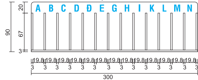
MẶT ĐÚNG
