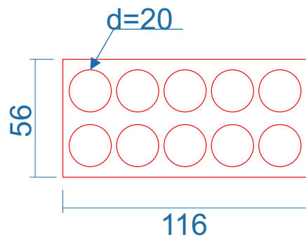
MẶT BẰNG
