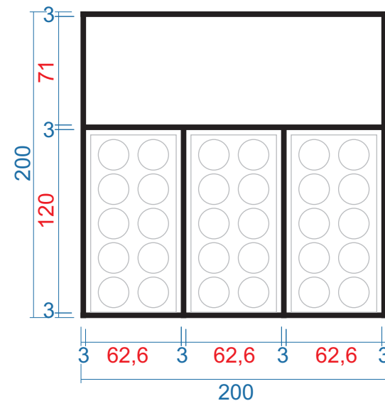
MẶT BẰNG
