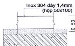
CHI TIẾT D1
