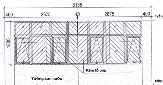
MẶT ĐÚNG BỐ TRÍ RÈM TỔ ONG VÁCH KÍNH VK5
