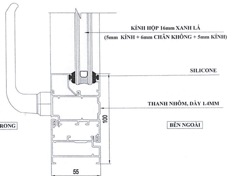
CHI TIẾT 4
