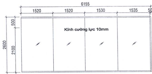
VÁCH INOX KÍNH CƯỜNG LỰC VK2 (Trước khi cải tạo)
