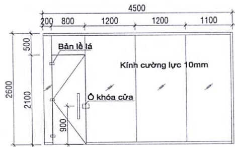
VÁCH INOX KÍNH CƯỜNG LỰC VK3
