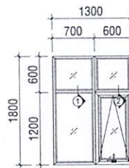
MẶT ĐÚNG CỬA SỔ VK4
