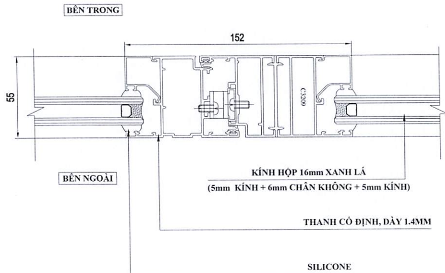
CHI TIẾT 7
