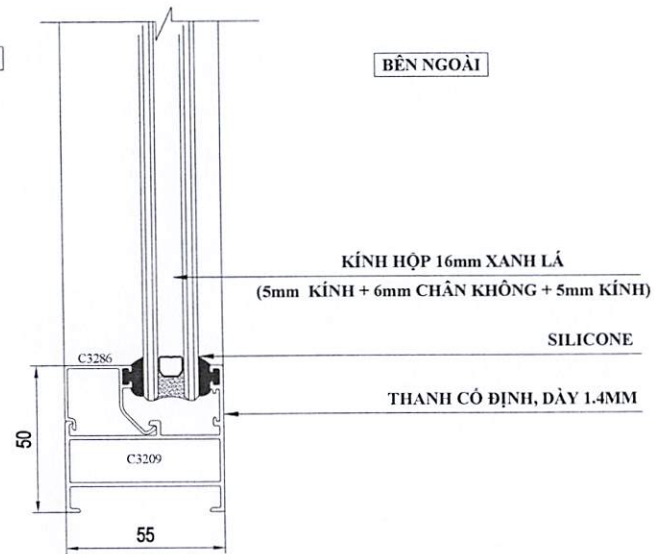
CHI TIẾT 1
