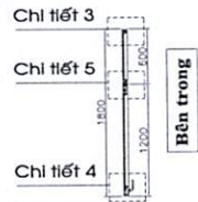
MẶT CẮT 2-2
