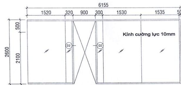
VÁCH INOX KÍNH CƯỜNG LỰC VK2 (Sau khi cải tạo)
