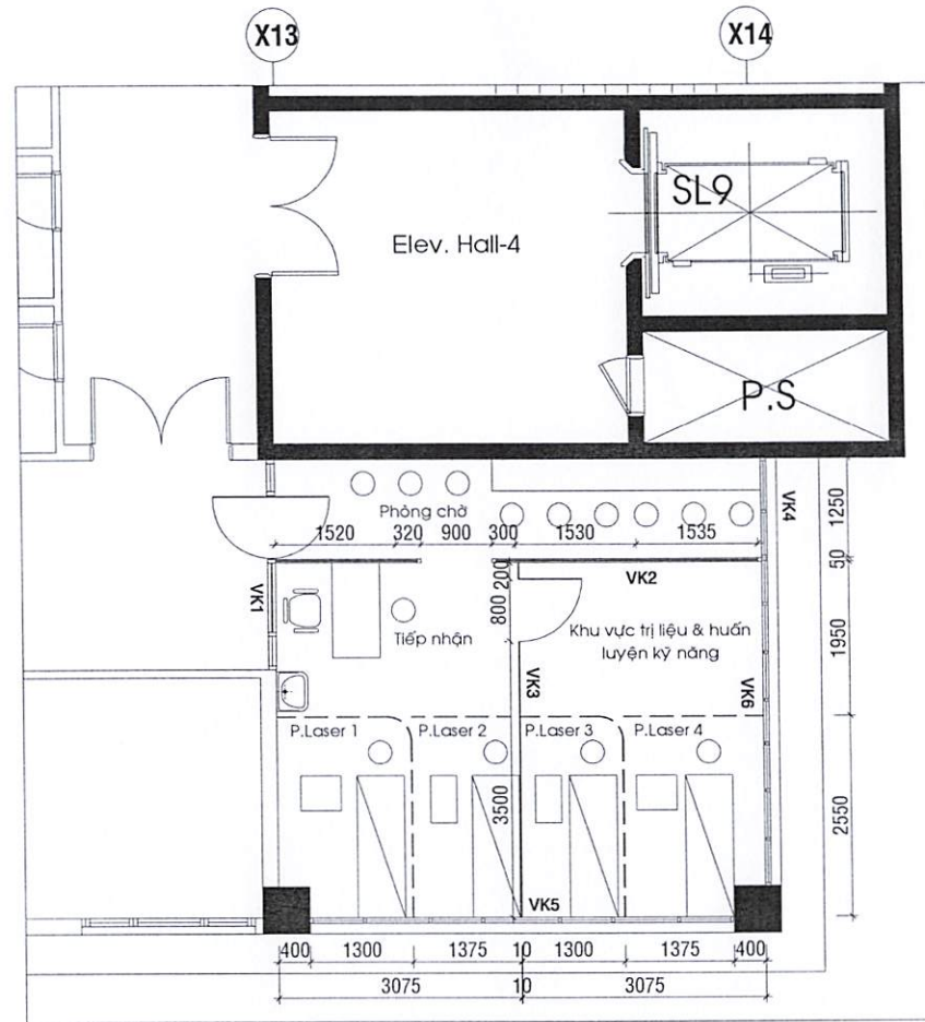
MẶT BẰNG OUTDOOR LẦU 8 BLOCK B SAU KHI CẢI TẠO ( ĐƠN VỊ LASER, ẢNH SÁNG VÀ SÓNG TRONG DA LIỀU )
