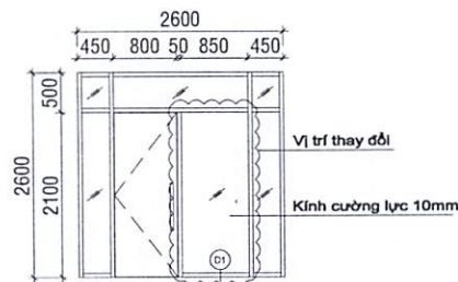
VÁCH INOX KÍNH CƯỜNG LỰC VK1 (Sau khi cải tạo)
