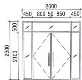
VÁCH INOX KÍNH CƯỜNG LỰC VK1 (Trước khi cải tạo)
