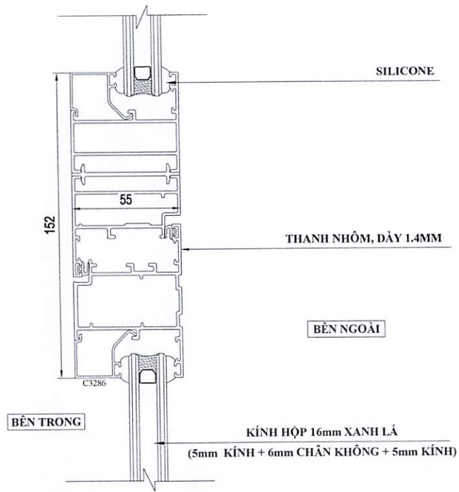
CHI TIẾT 5
