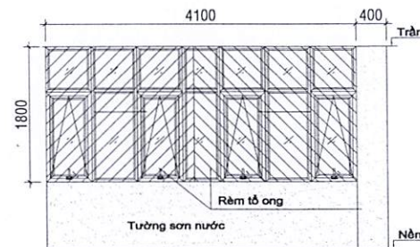
MẶT ĐÚNG BỐ TRÍ RÈM TỔ ONG VÁCH KÍNH VK6
