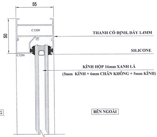
CHI TIẾT 1
