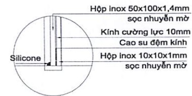
CHI TIẾT D2
