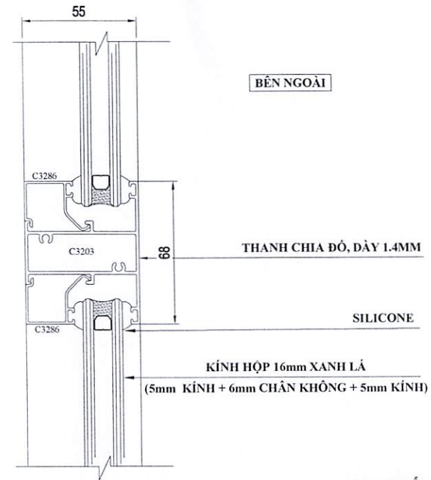
CHI TIẾT 2
