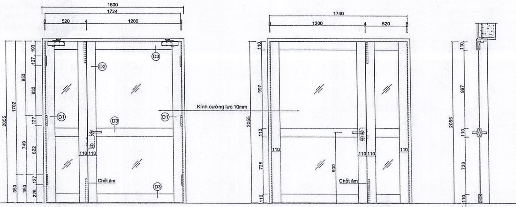
MẶT ĐỪNG NGOÀI
