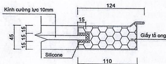
CHI TIẾT D2
