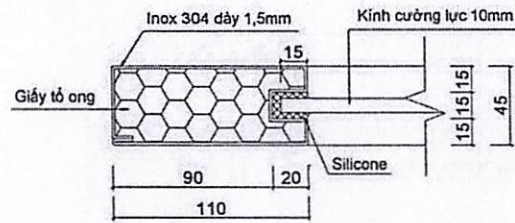
CHI TIẾT D1
