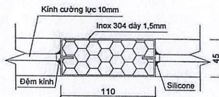
CHI TIẾT D3
