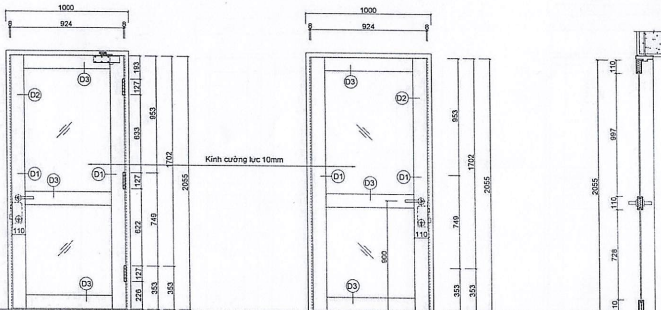
MẶT ĐỨNG NGOÀI
