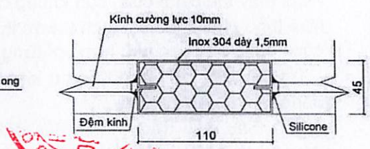
CHI TIẾT D3
