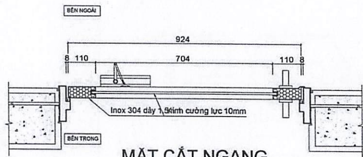
MẶT CẮT NGANG
