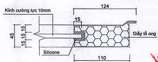
CHI TIẾT D2
