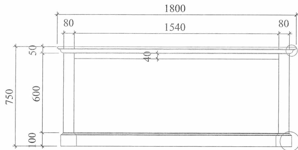
MẶT SAU
