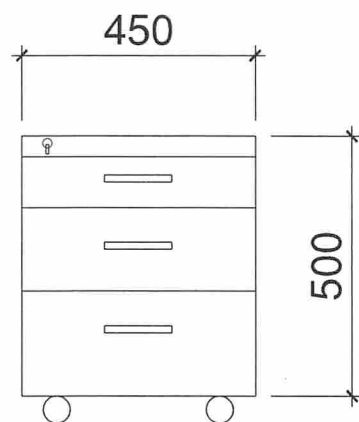
MẶT ĐỨNG
