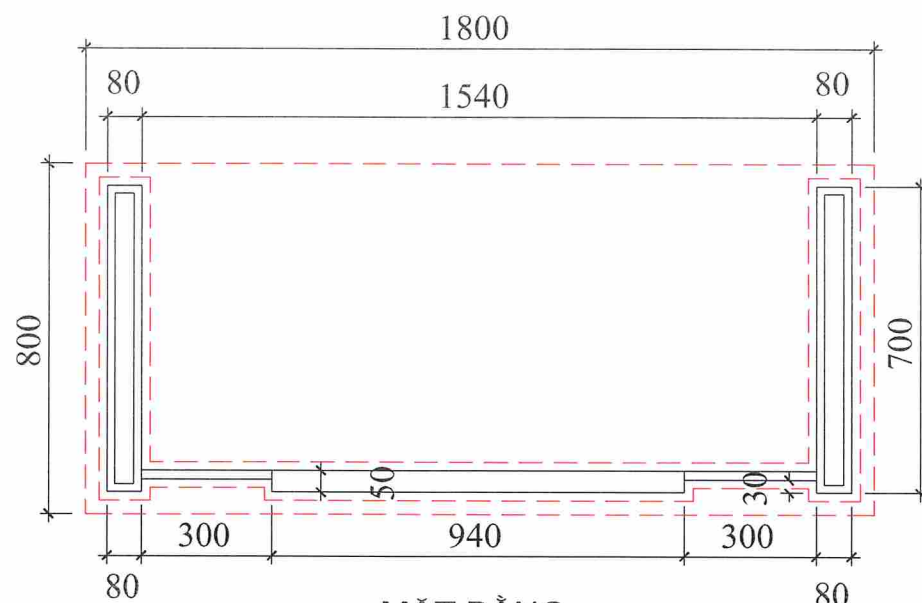
MẶT BẰNG
