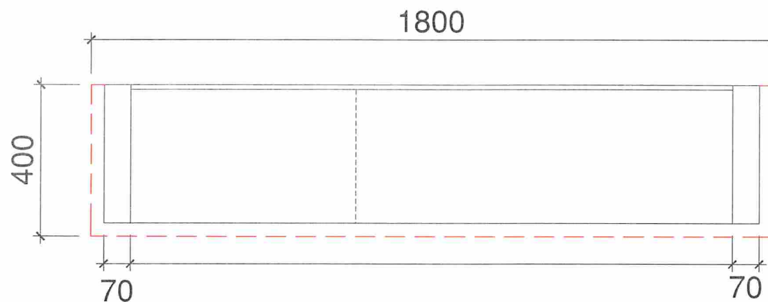
MẶT BẰNG
