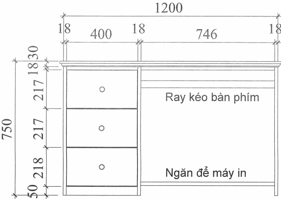
MẶT ĐỨNG
