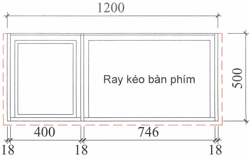
MẶT BẰNG
