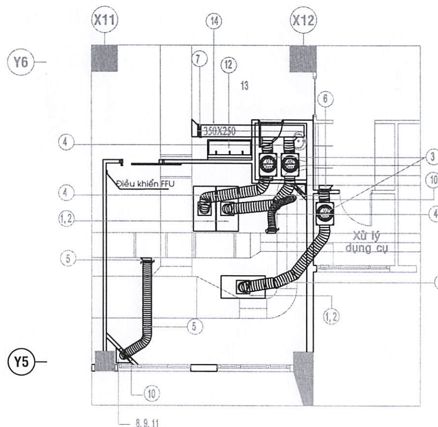
MẶT BẰNG BỐ TRÍ ỐNG GIÓ PHÒNG MỔ 3 (THAY ĐỔI)
