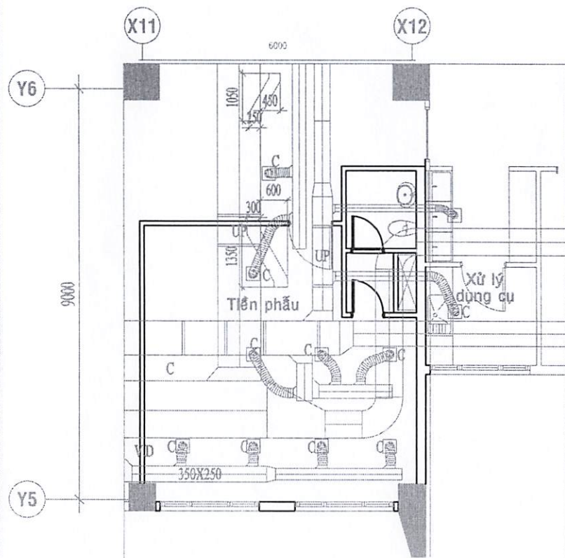
MẶT BẰNG BỐ TRÍ ỐNG GIÓ- LẦU 6 (HIỆN HỮU)
