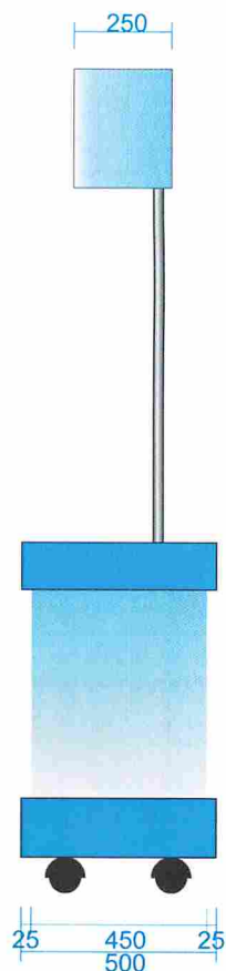
Mặt bên
