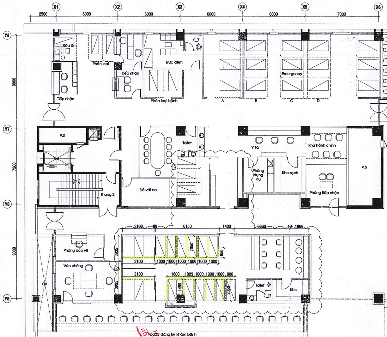
MẶT BẰNG RÈM CHE Y TẾ KHOA CẤP CỨU TẦNG TRỆT
