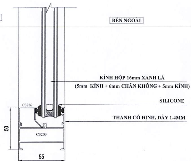
CHI TIẾT 1
