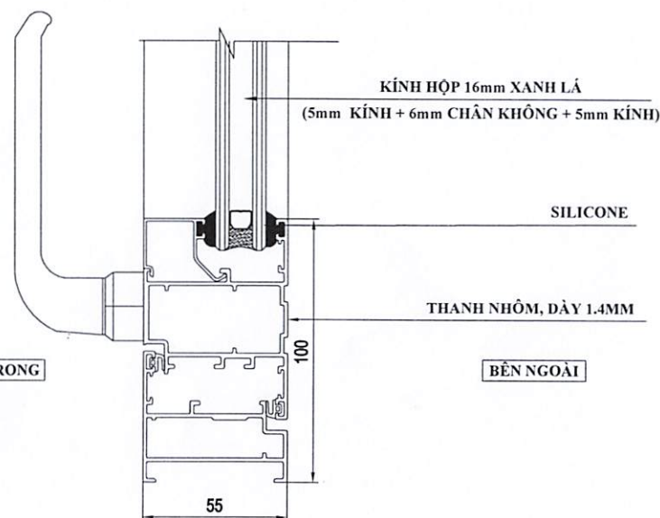
CHI TIẾT 4
