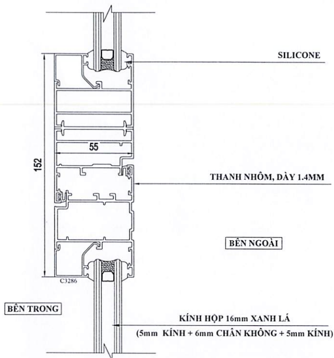
CHI TIẾT 5
