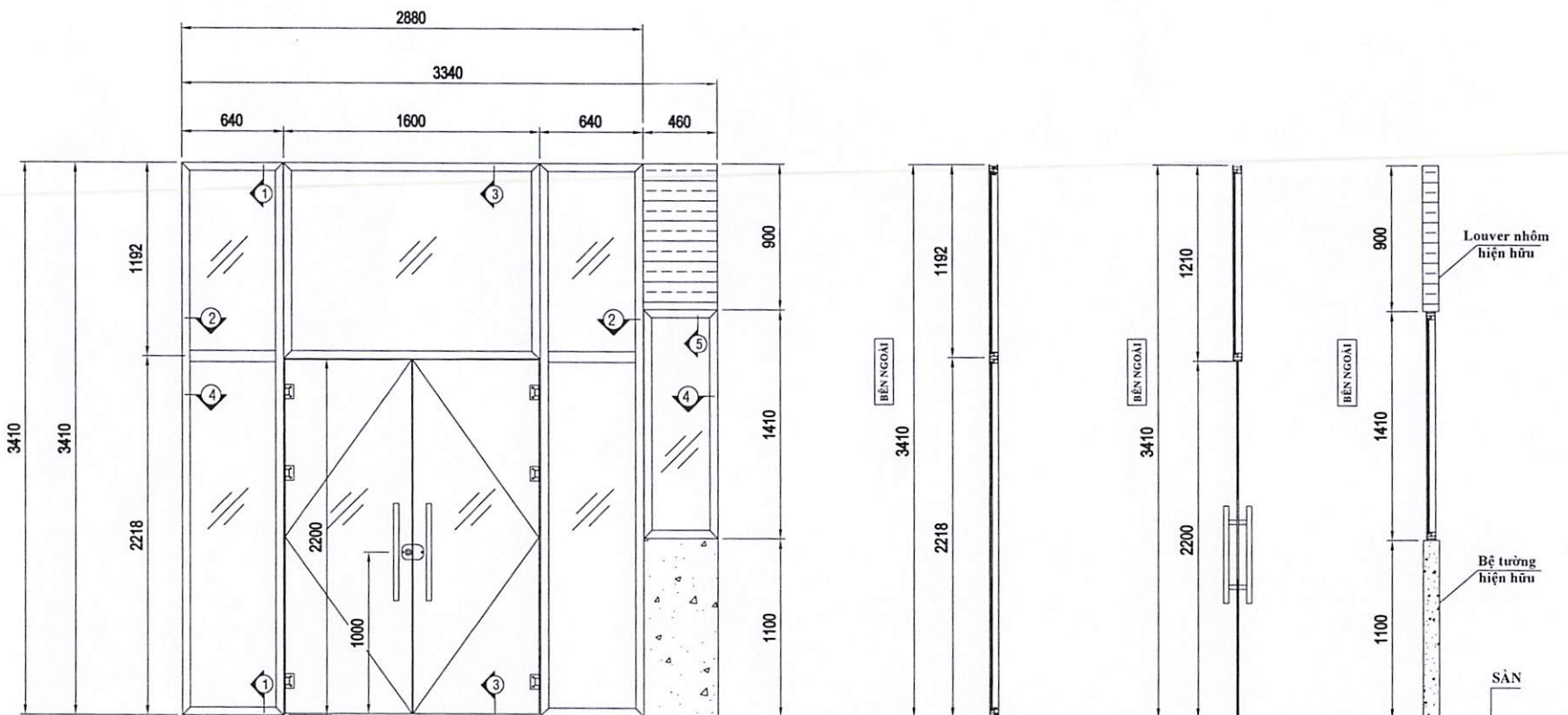
MẶT BẰNG VÁCH NHÔM KÍNH
