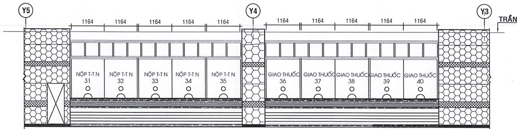
MẶT ĐỨNG HIỆN TRẠNG NHÀ THUỐC TẦNG TRỆT KHU A
