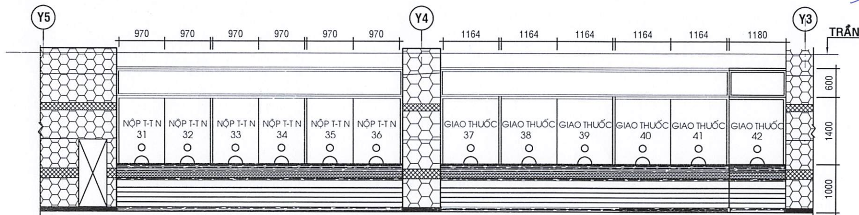
MẶT ĐỨNG NHÀ THUỐC TẦNG TRỆT KHU A (SAU KHI SỬA CHỮA)
