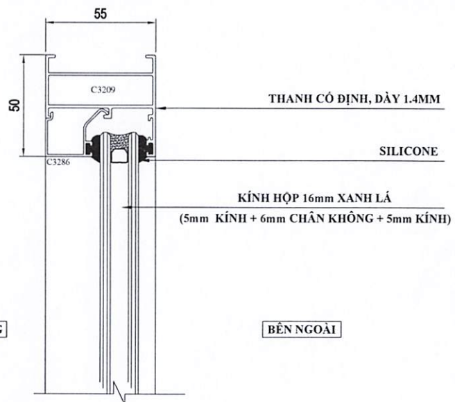
CHI TIẾT 1
