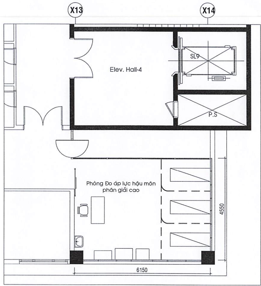
MẶT BẰNG KHU VỰC NGOÀI TRỜI LẦU 12 BLOCK B TL:1/100 (TRƯỚC KHI CẢI TẠO)
