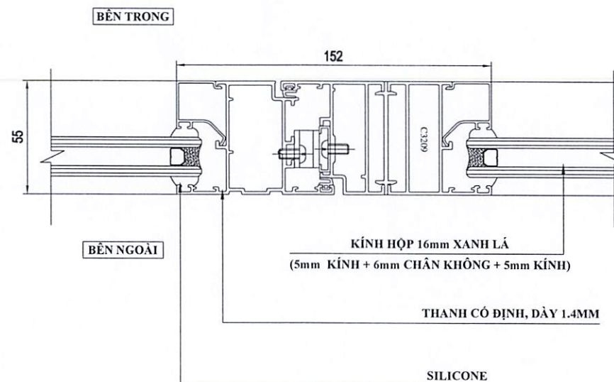
CHI TIẾT 7
