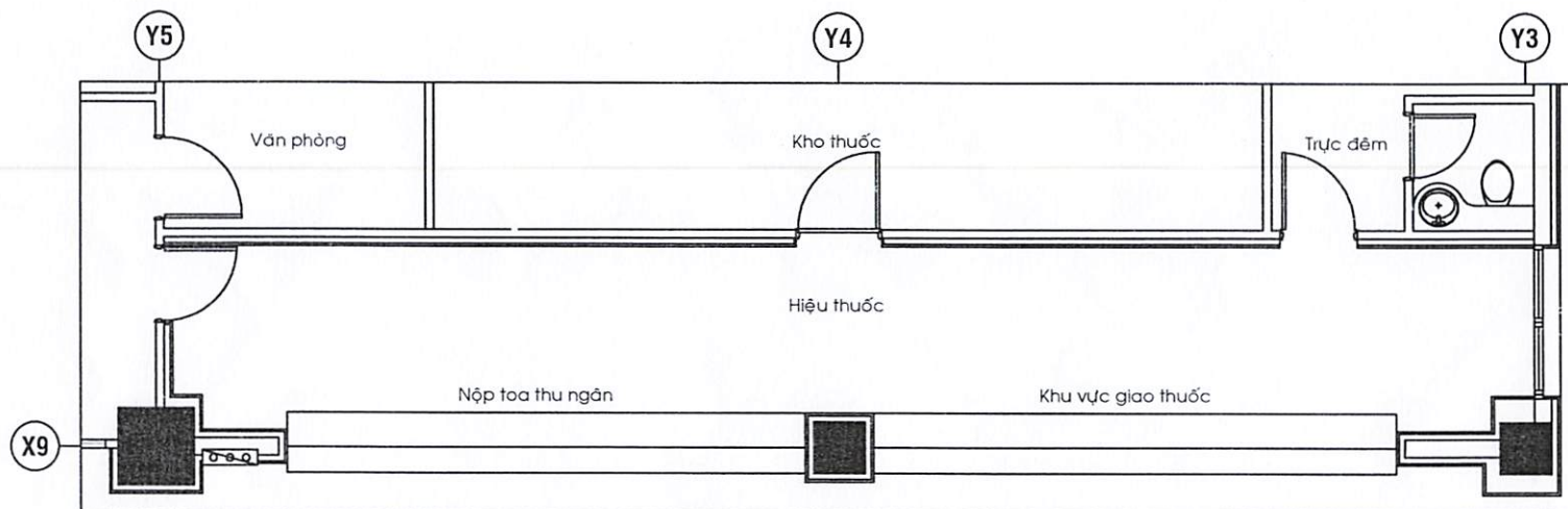
MẶT BẰNG HIỆN TRẠNG NHÀ THUỐC TẦNG TRỆT KHU A
