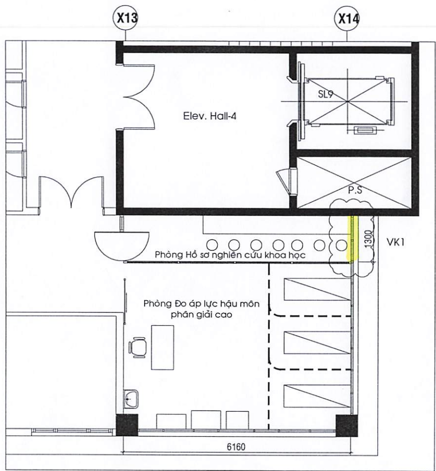
MẶT BẰNG KHU VỰC NGOÀI TRỜI LẦU 12 BLOCK B TL:1/100 (SAU KHI CẢI TẠO) ( PHÒNG HỒ SƠ NGHIÊN CỨU KHOA HỌC)
