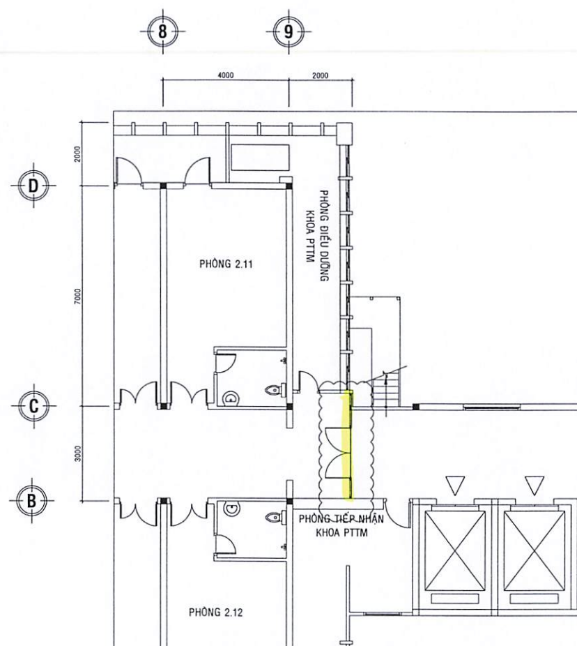
MẶT BẰNG LẦU 2 KHU B SAU KHI SỬA CHỮA
