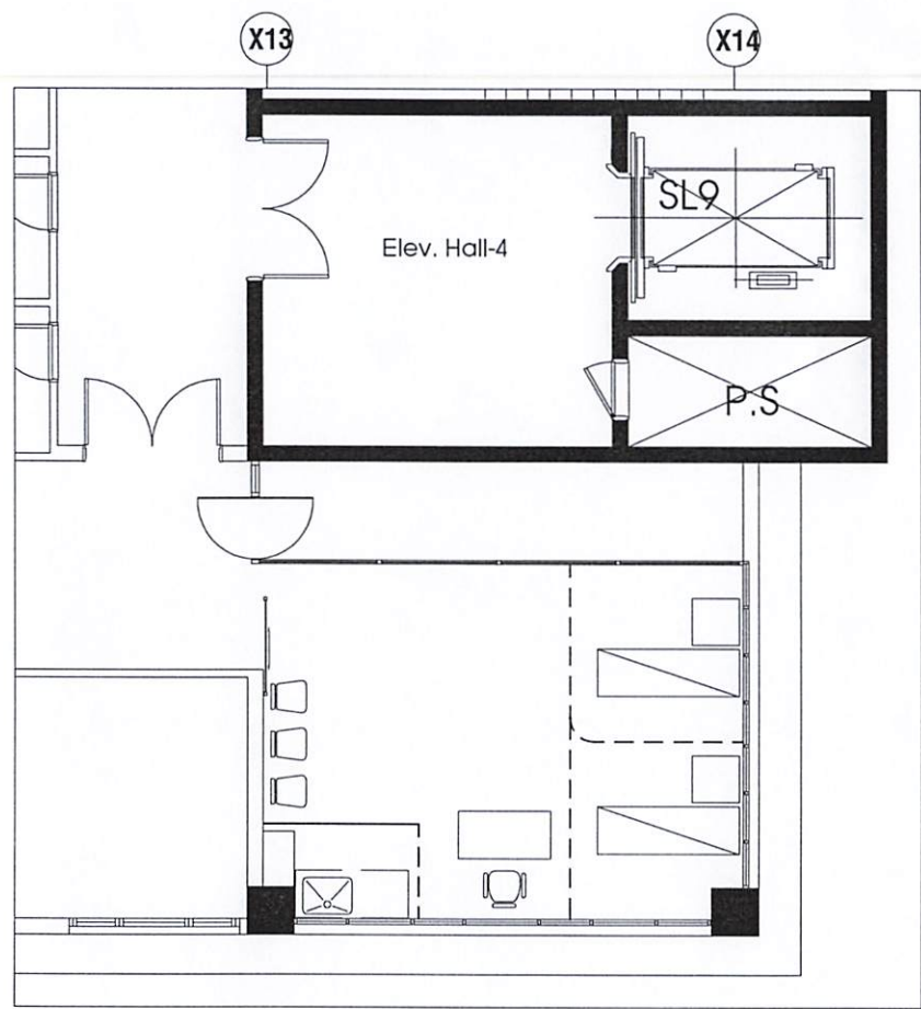
MẶT BẰNG KHU VỰC NGOÀI TRỜI LẦU 13 BLOCK B TL:1/100 (TRƯỚC KHI CẢI TẠO)
