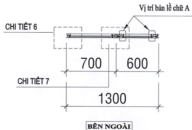
MẶT BẰNG CỬA SỔ VK1
