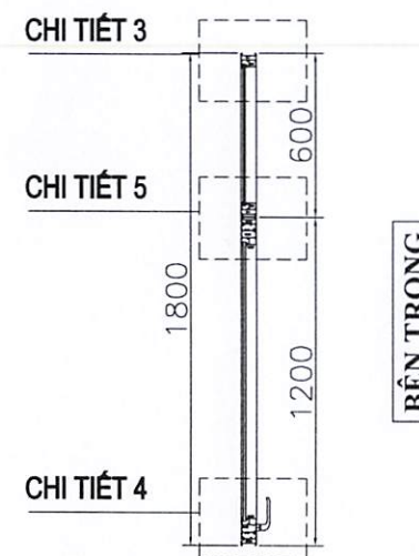
MẶT CẮT 2-2
