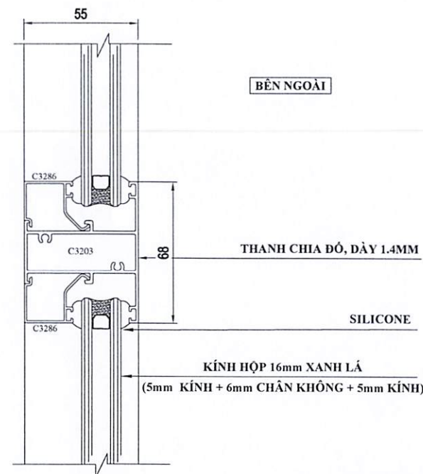
CHI TIẾT 2
