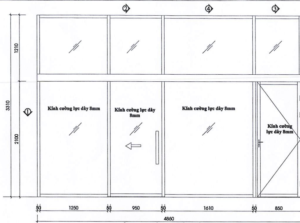
MẶT ĐÚNG (HƯỚNG NHÌN TỪ NGOÀI VÀO)
