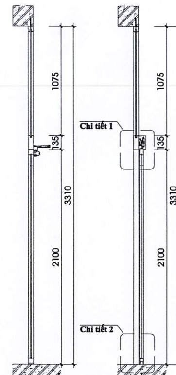
MẶT CẮT 2-2 (Tỷ lệ 1/30)
