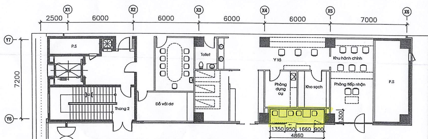
MẶT BẰNG TẦNG TRỆT TRƯỚC KHI SỬA CHỮA
