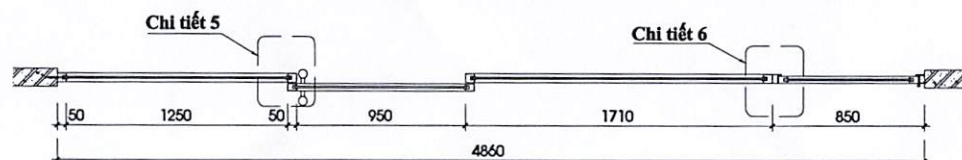
MẶT CẮT 1-1
