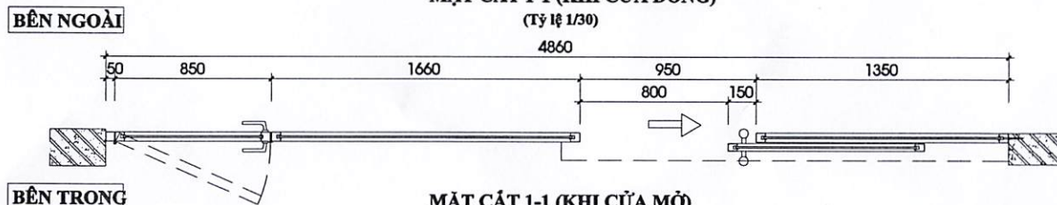
MẶT CẮT 1-1 (KHI CỬA MỞ) (Tỷ lệ 1/30)
