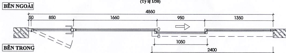
MẶT CẮT 1-1 (KHI CỬA ĐÓNG) (Tỷ lệ 1/30)
