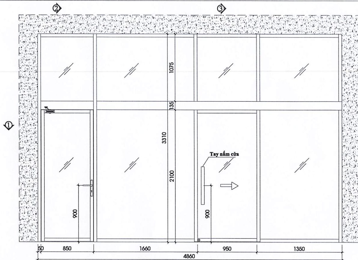
MẶT ĐÚNG (HƯỚNG NHÌN TỪ TRONG RA) (Tỷ lệ 1/30)
