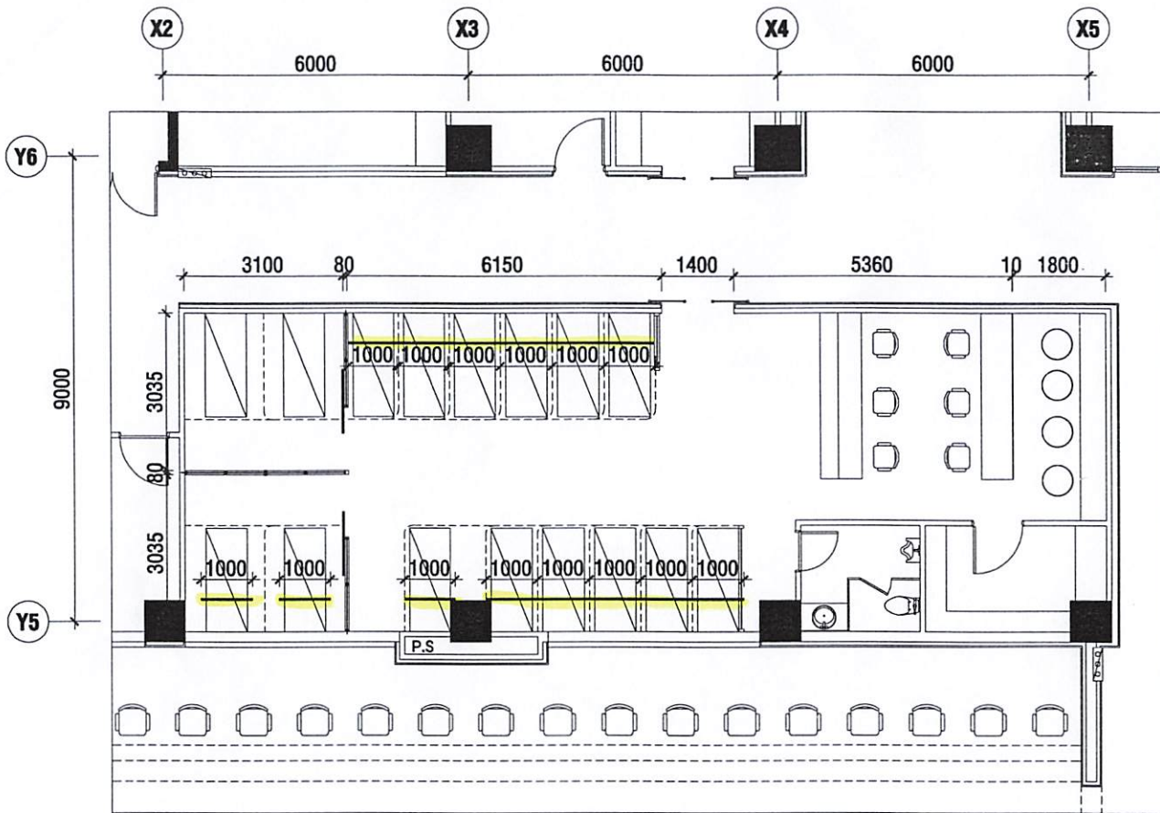
MẶT BẰNG THANH TREO DỊCH TRUYỀN KHOA CẤP CỨU TẦNG TRỆT
