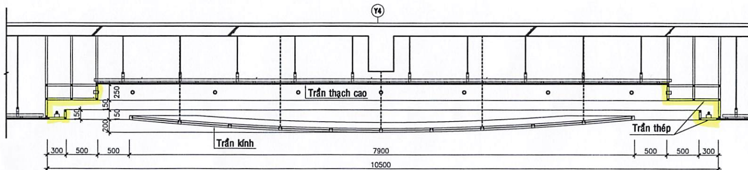
MẶT CẮT 1 - 1
