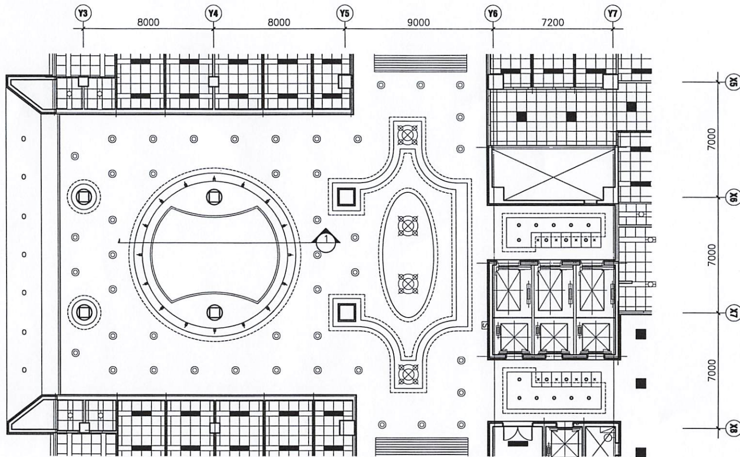
MẶT BẰNG TRẦN SÂN H CHÍNH LẦU 1
