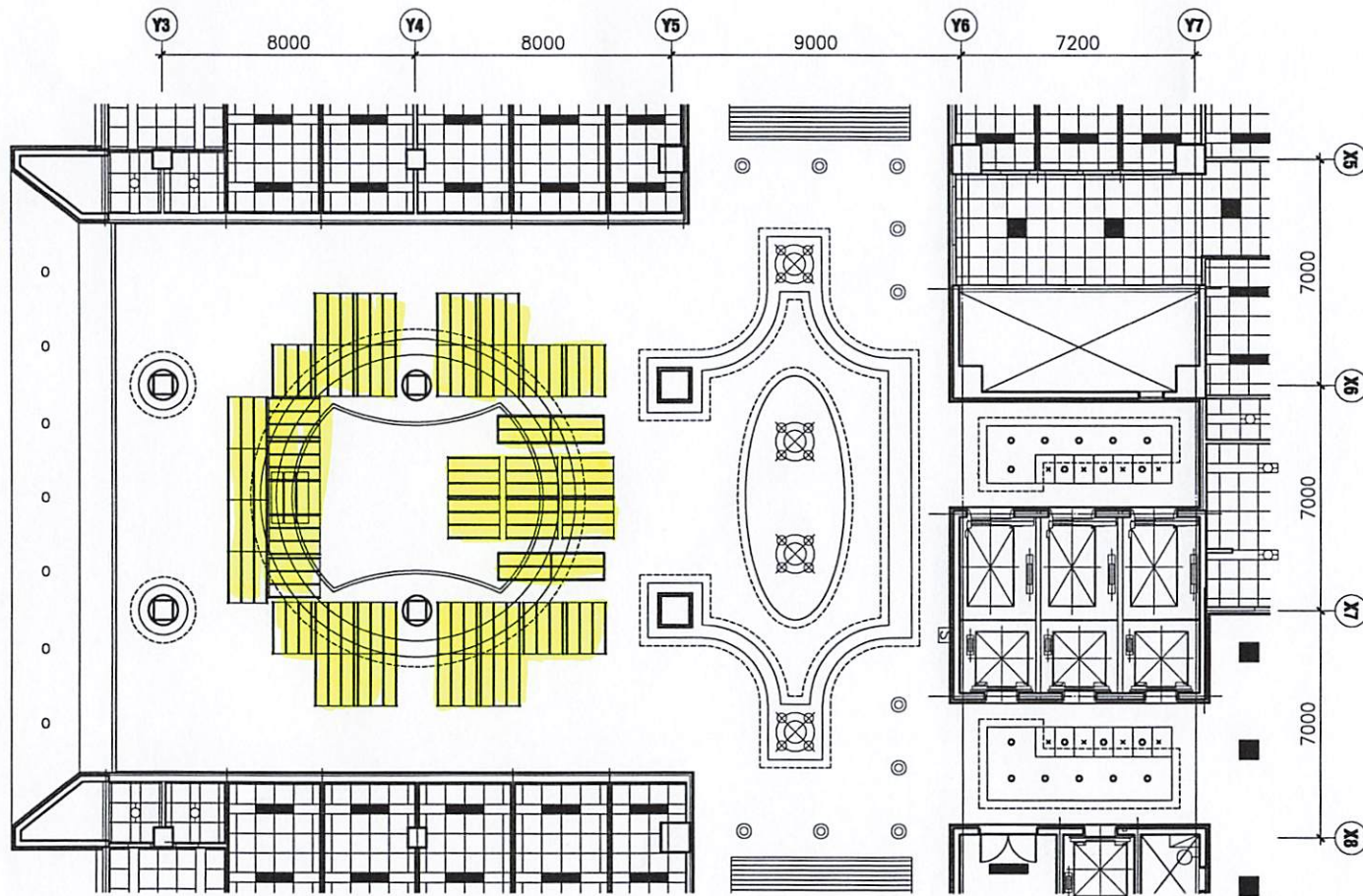
MẶT BẰNG BỐ TRÍ GIÀN GIÁO TRẦN SẢNH CHÍNH LẦU 1
