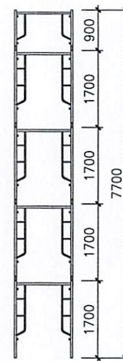
CHIỀU CAO GIÀN GIÁO
