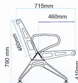
MẶT BÊN
